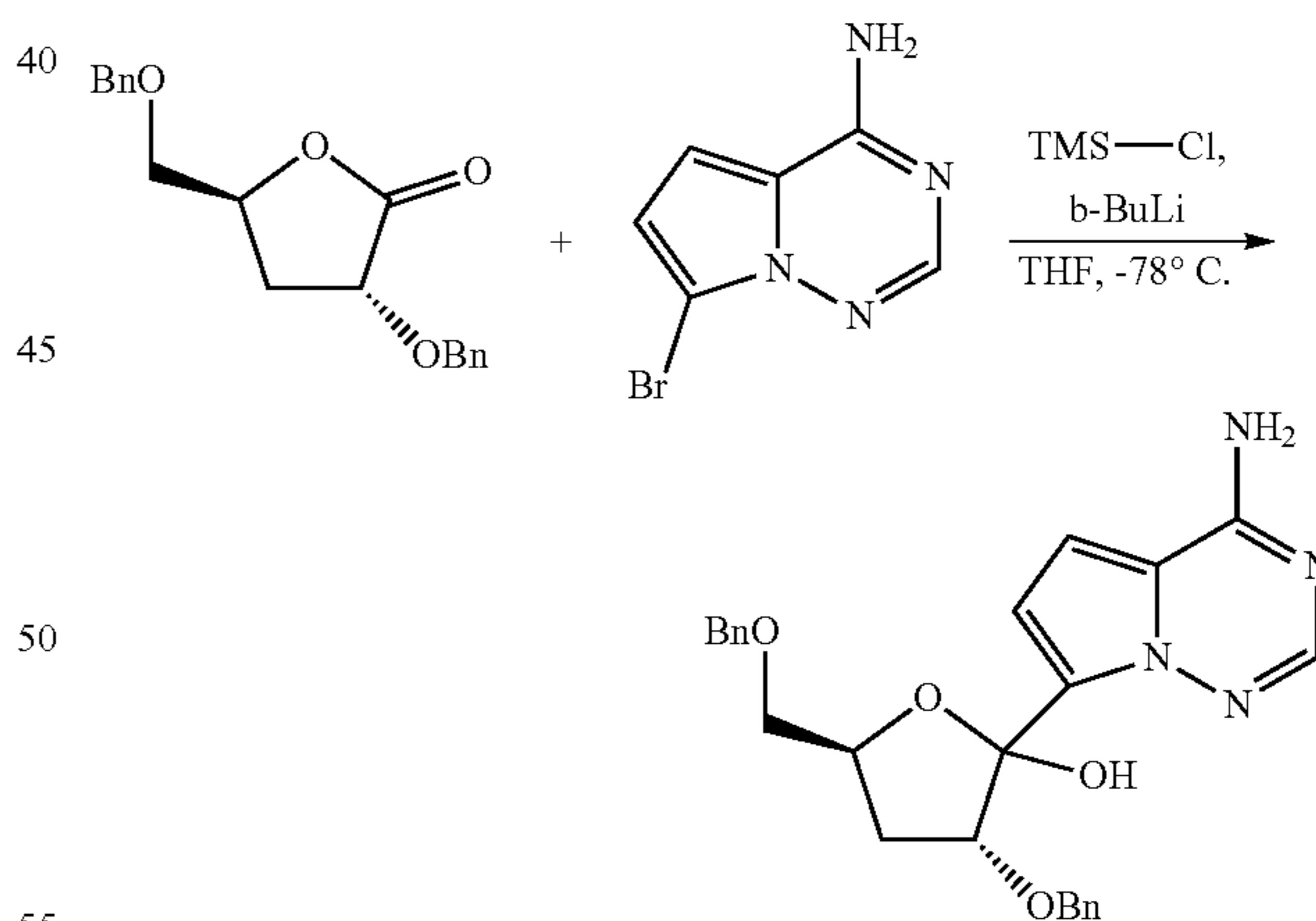
(3R,5S)-2-(4-aminopyrrolo[1,2-f][1,2,4]triazin-7-yl)-3-(benzyloxy)-5-(benzyloxymethyl)-tetrahydrofuran-2-ol
