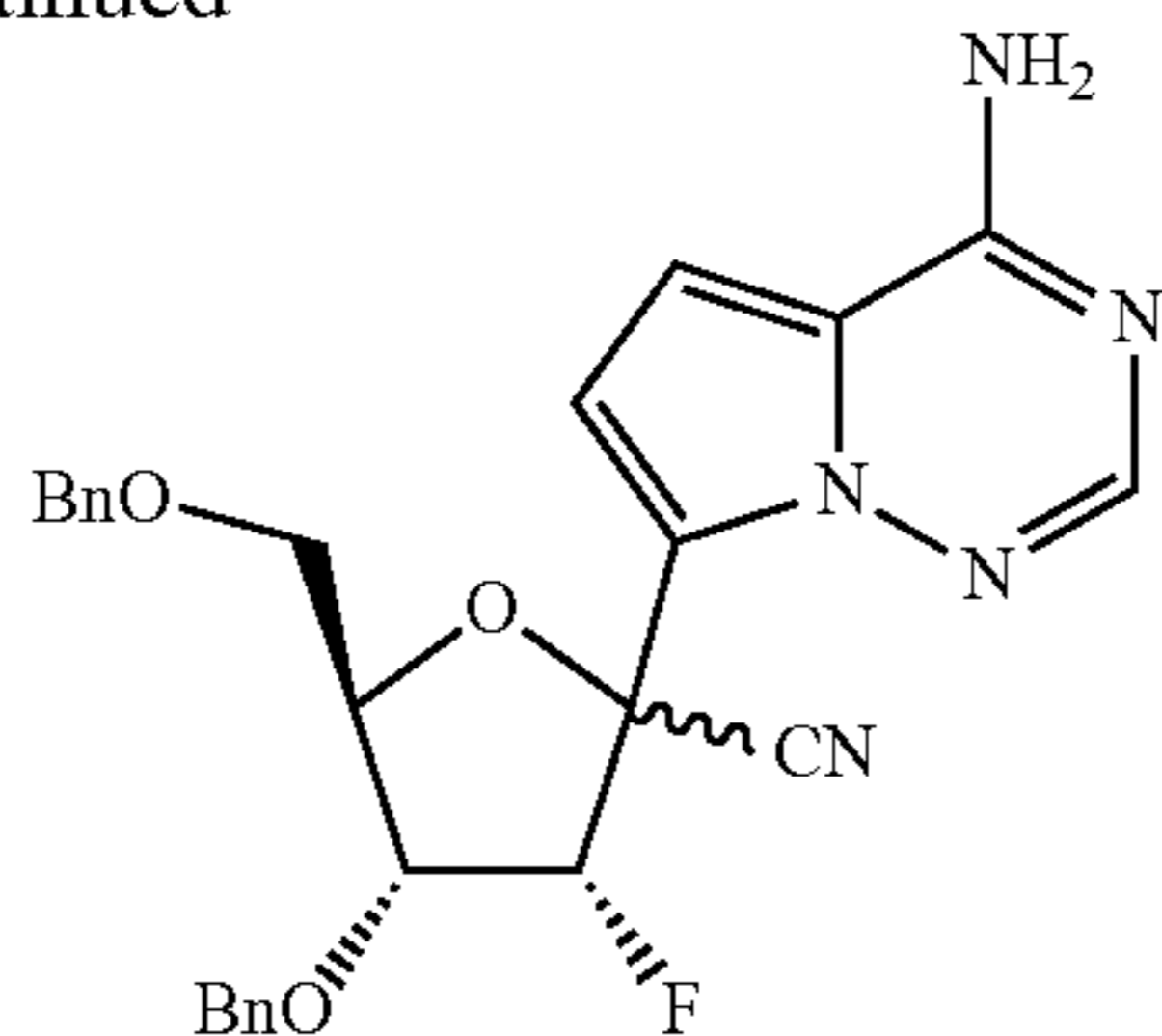
(3R, 4R, 5R)-2-(4-aminopyrrolo[1,2-f][1,2,4]triazin-7-yl)-4-(benzyloxy)-5-(benzyloxymethyl)-3-fluorotetrahydrofuran-2-carbonitrile
