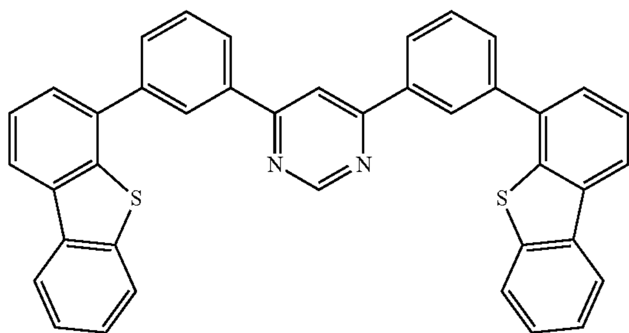
4,6mDBTP2Pm-II
