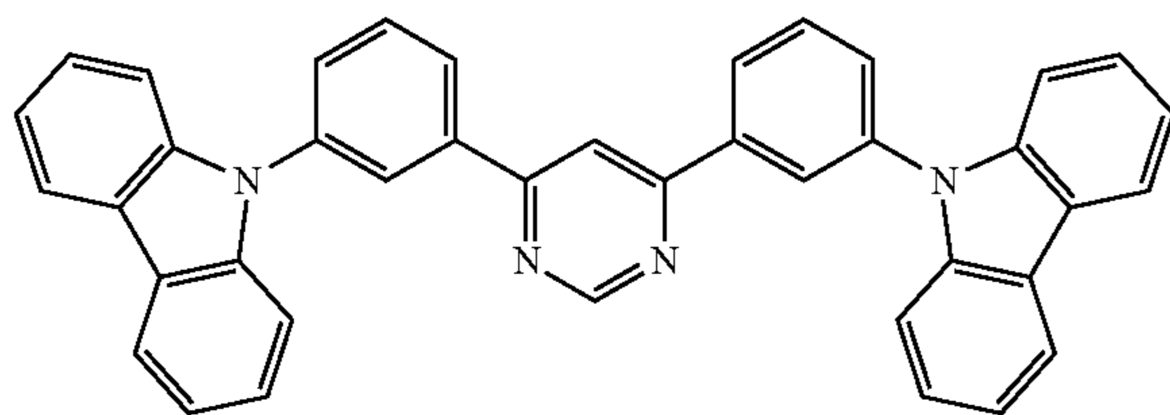
4,6mCzP2Pm
