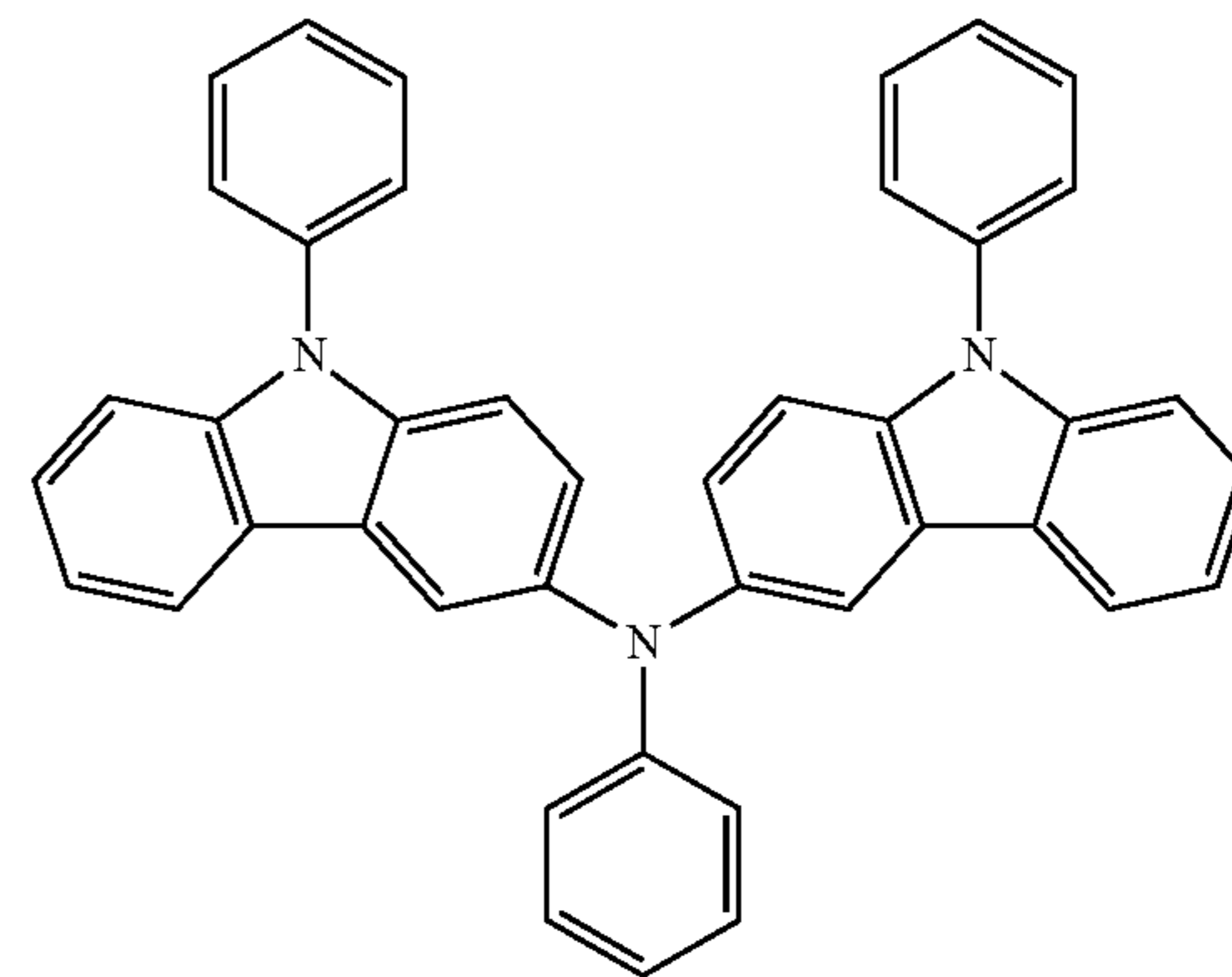
PCzPCA1
