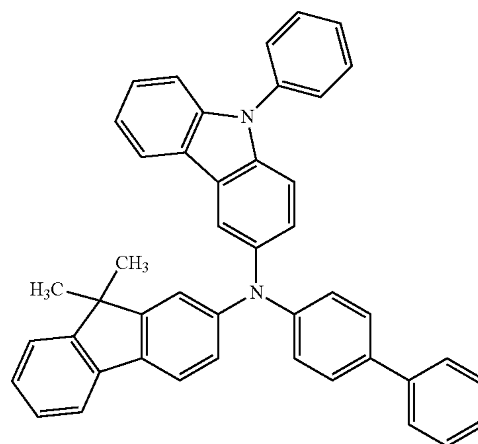
PCBiF
