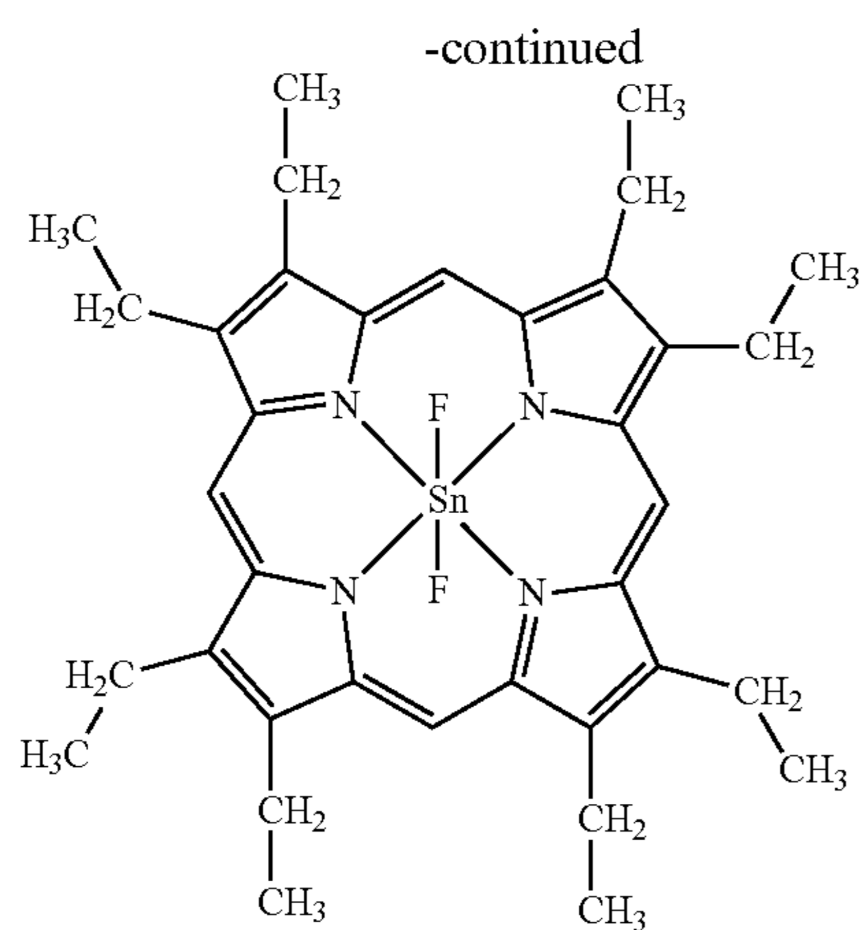
SnF 2 (OEP)
