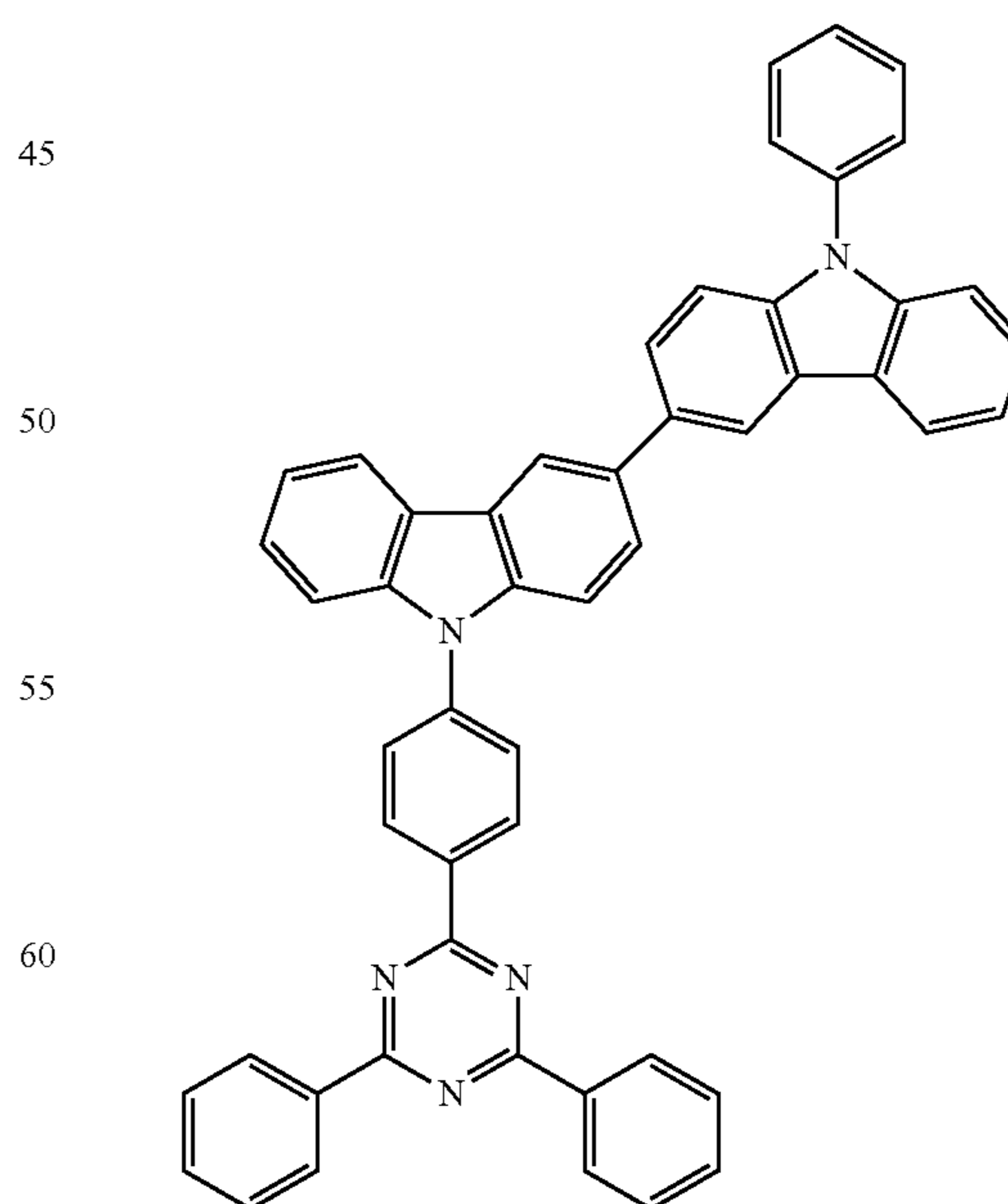
PCCzPTzn
