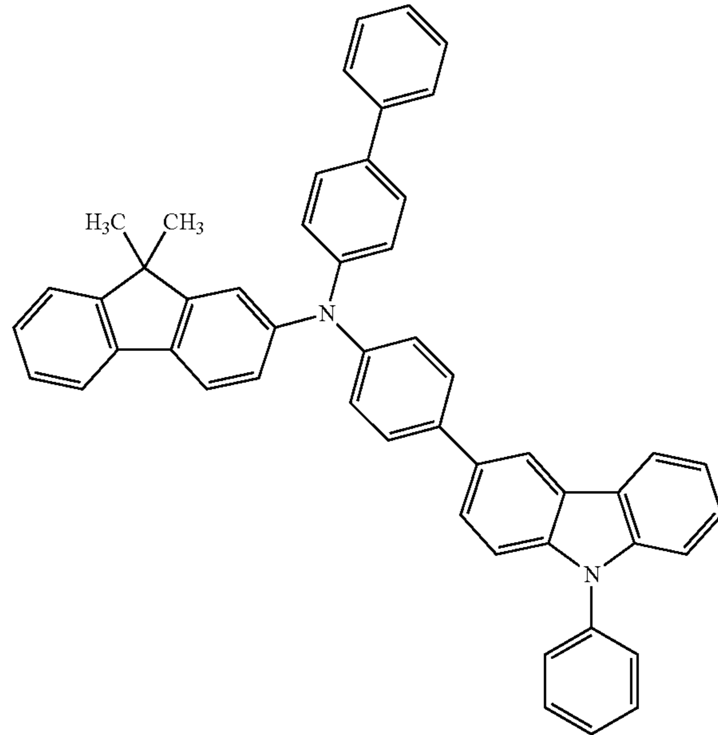
PCBBiF
