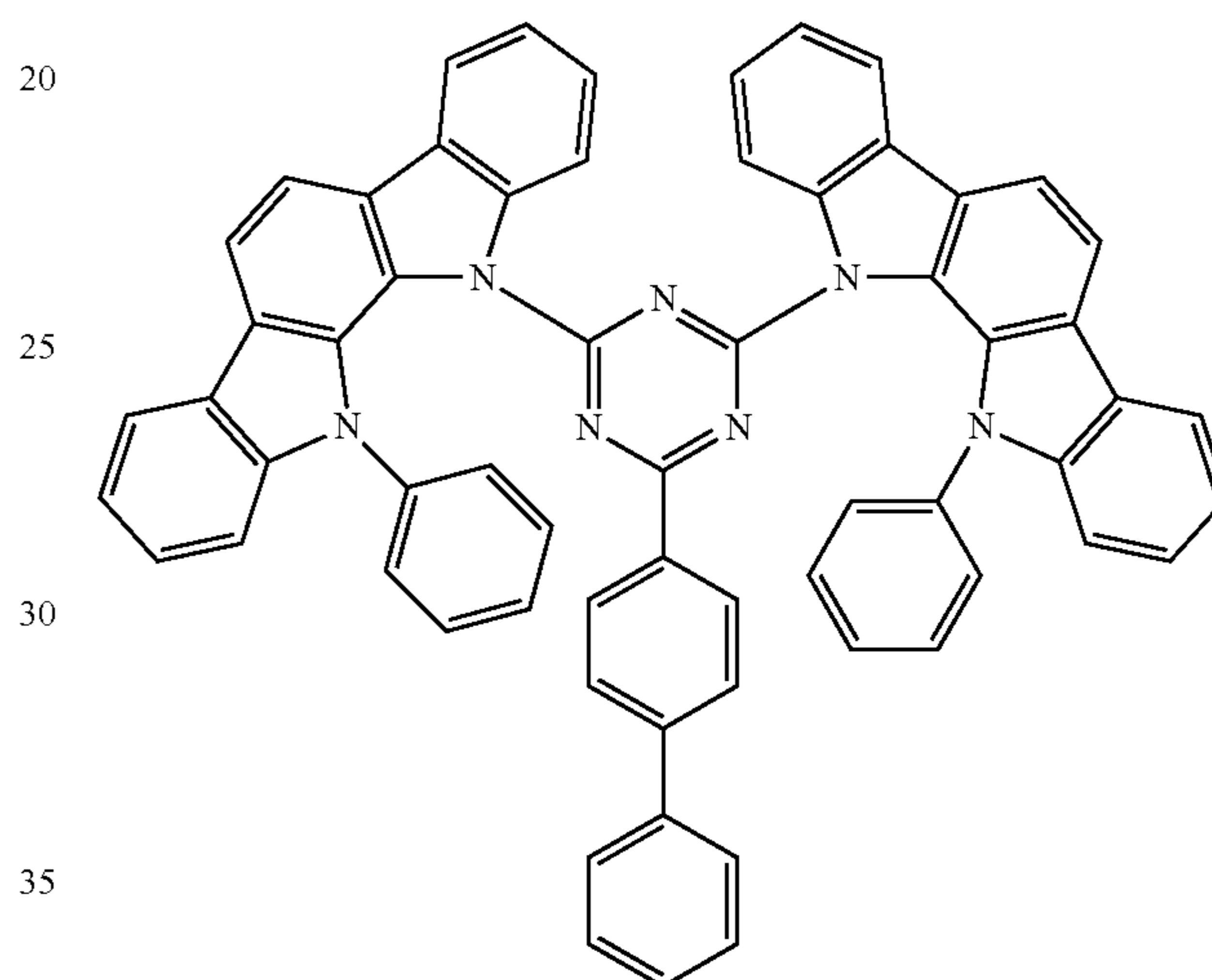
PIC-TRZ
