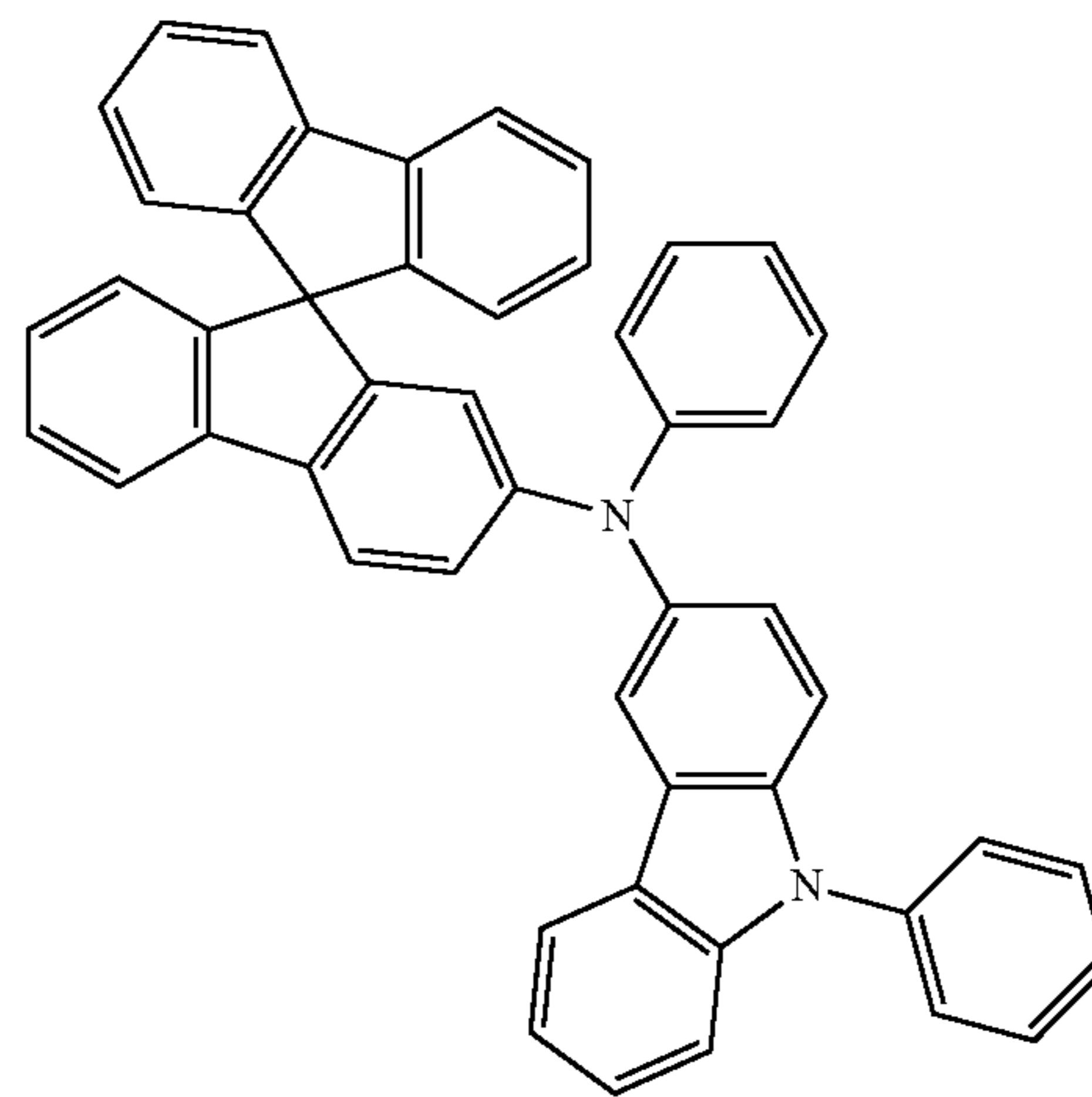
PCASF
