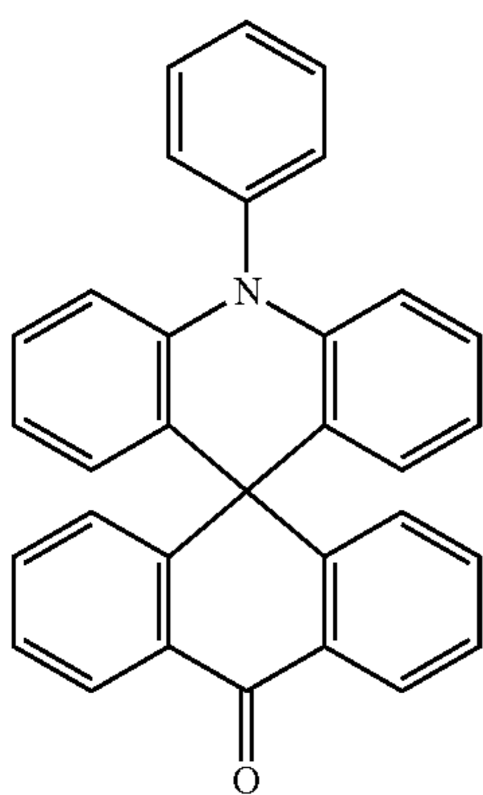
ACRSA
