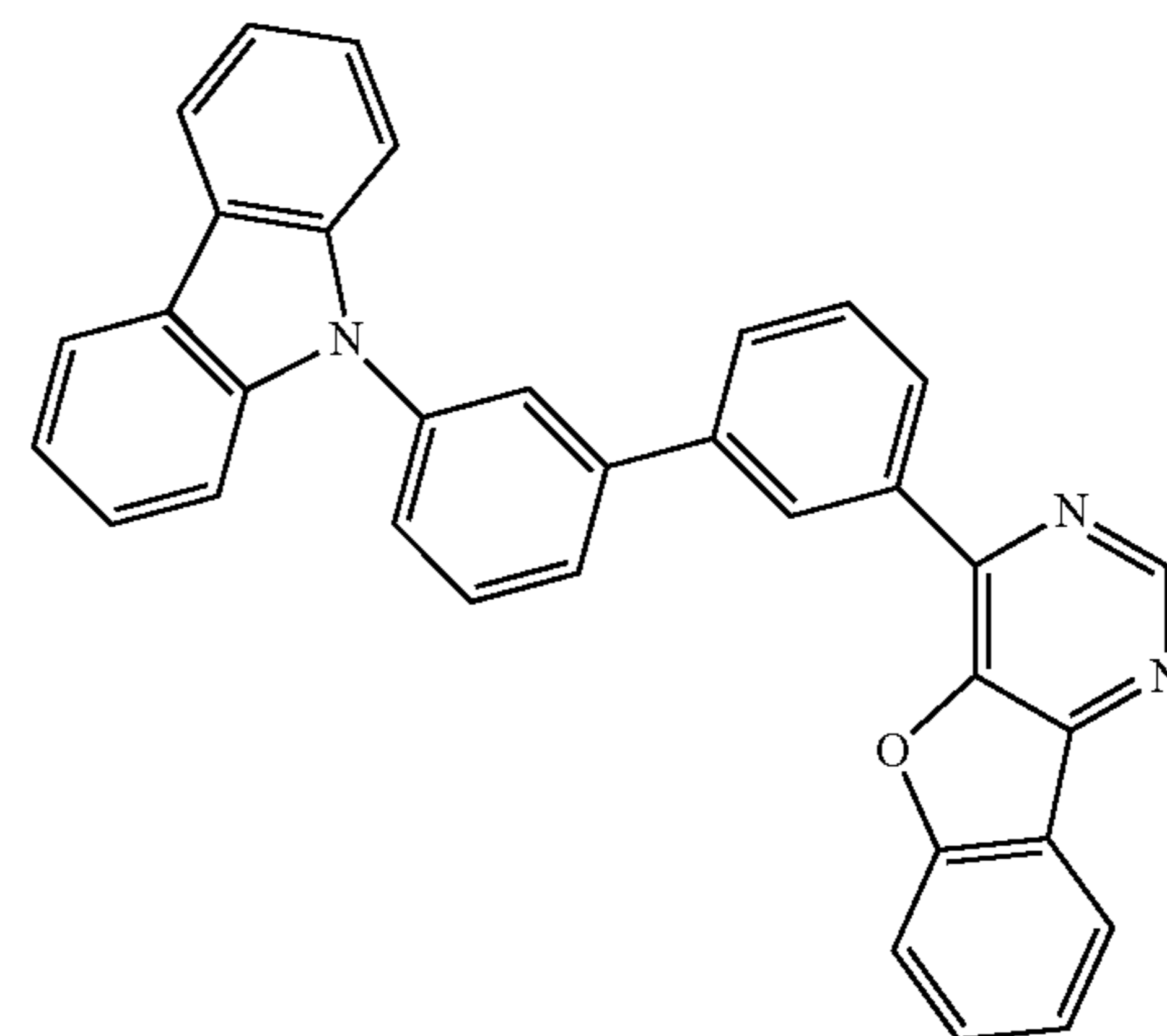
4mCzBPBfPm
