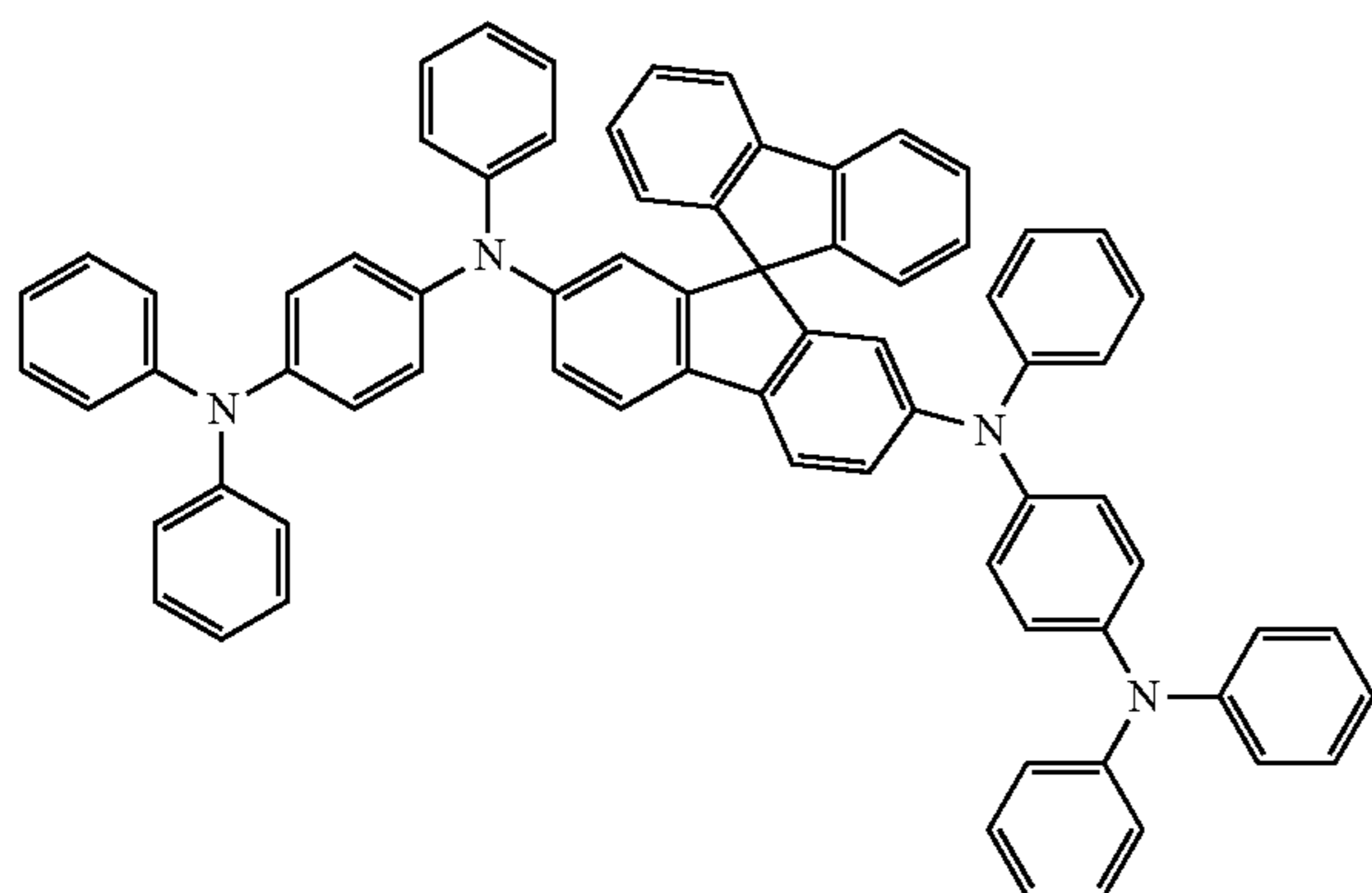
DPA2SF
