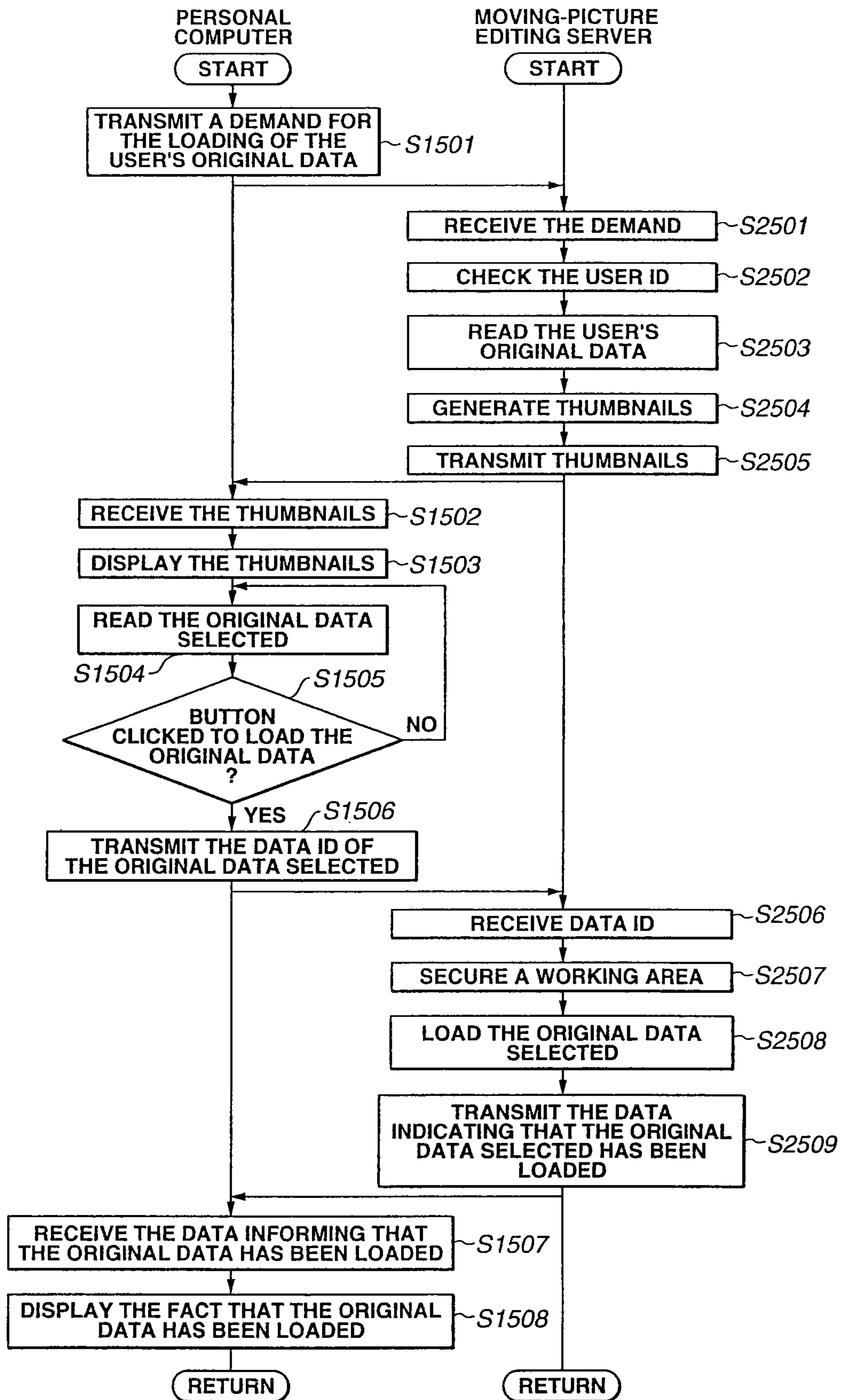
FIG.37
