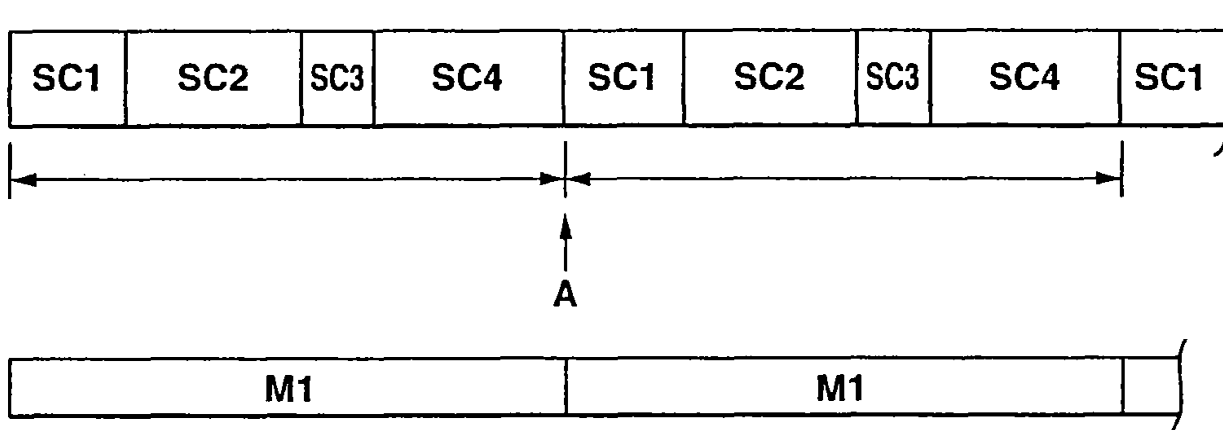
FIG. 45D
