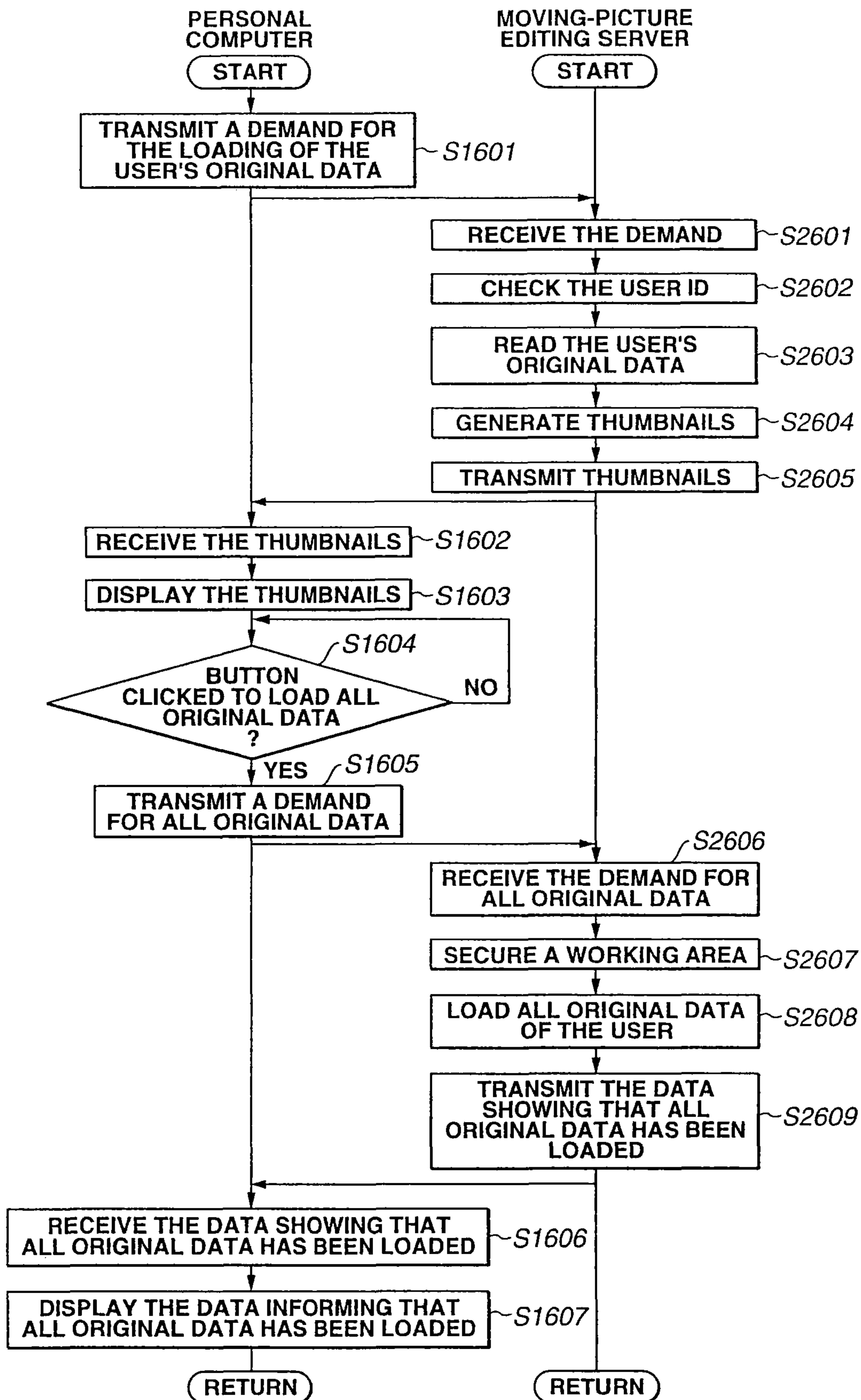
FIG.38
