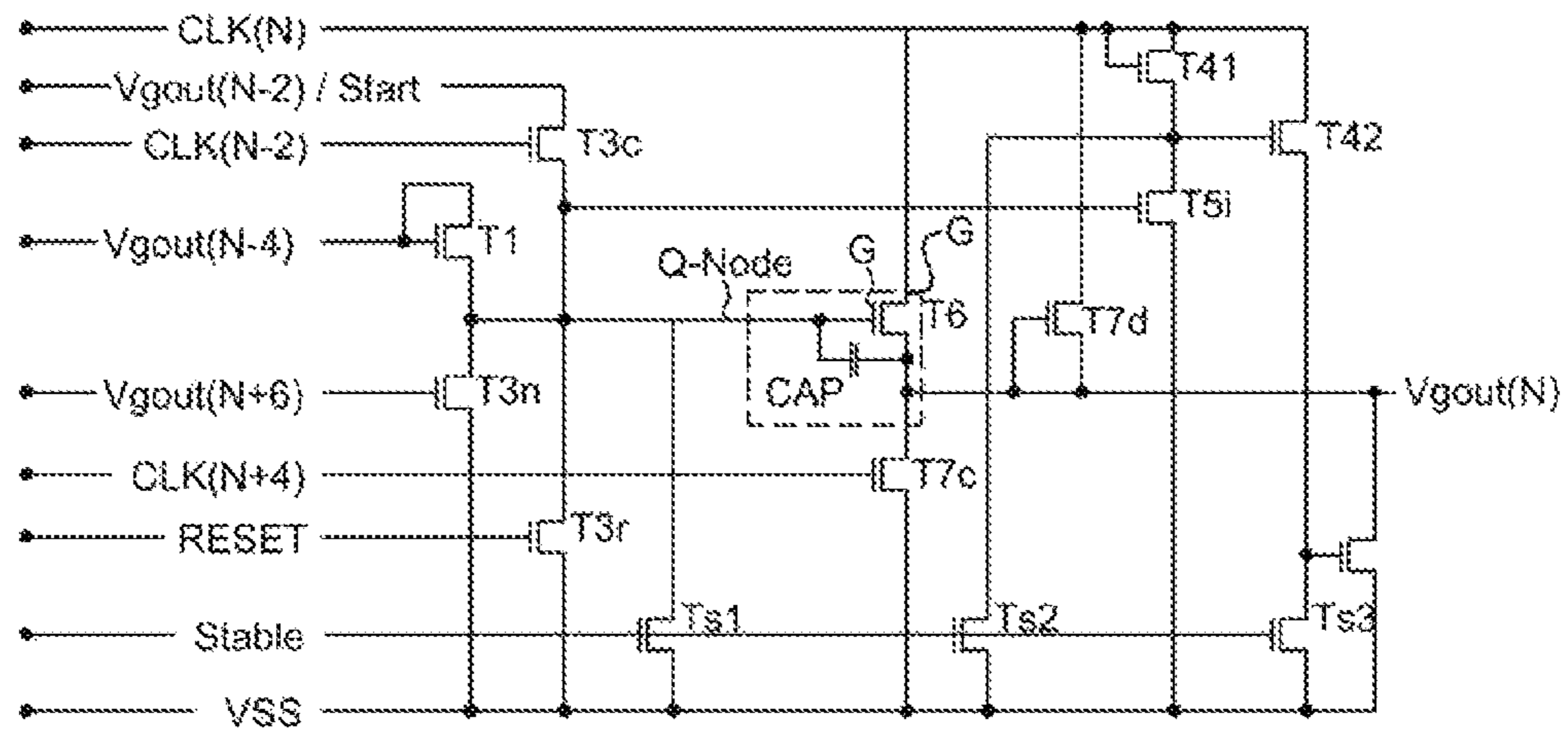
[GIP Stage(N)]
