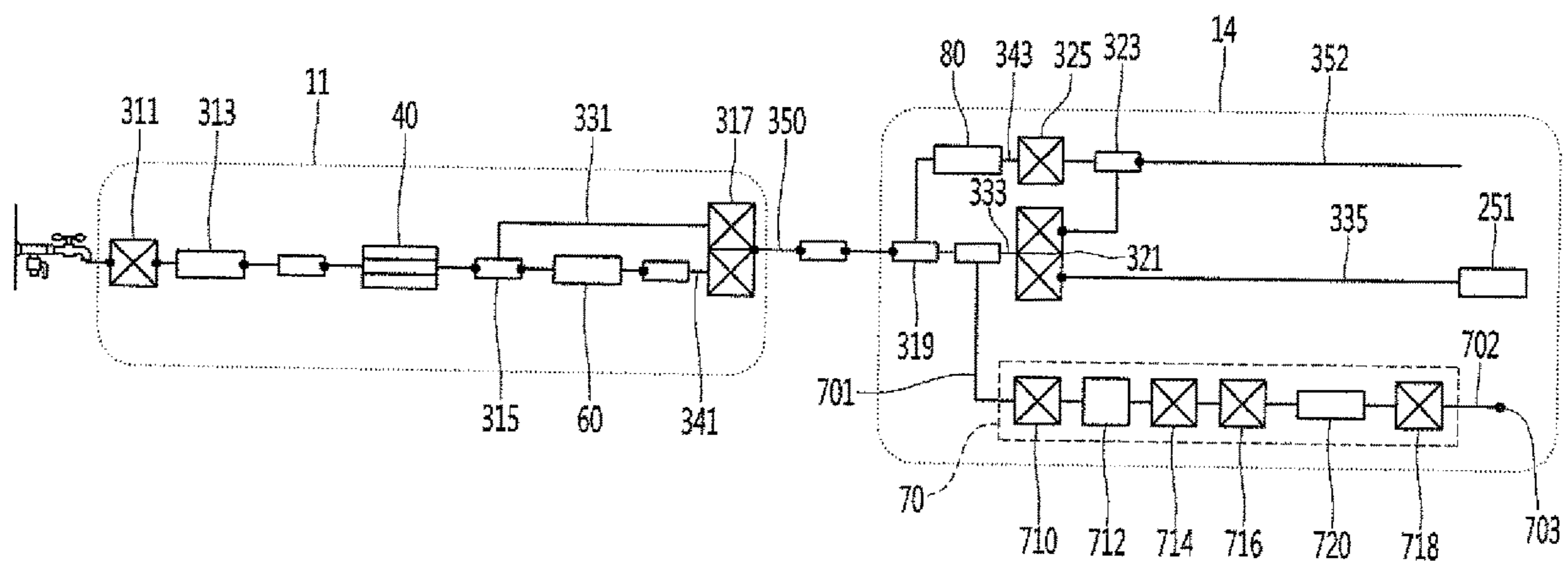
FIG. 3
