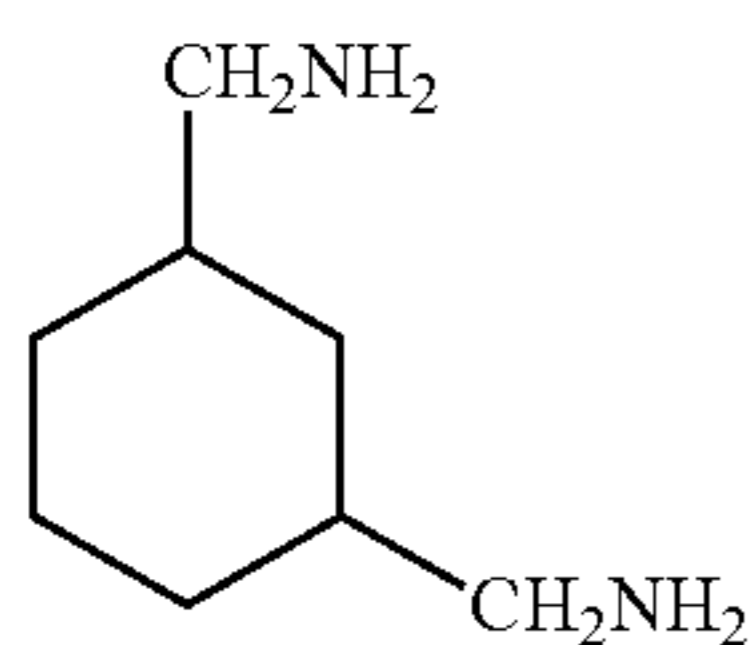
1,3-bis(methylamine)-cyclohexane,
