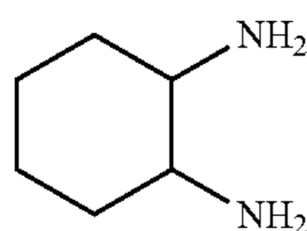
Cyclohexane-1,2-diamine
