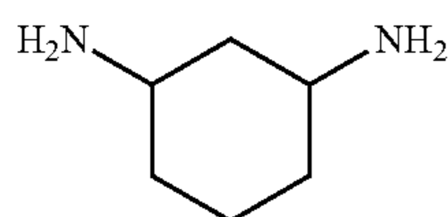
Cyclohexane-1,3-diamine,
