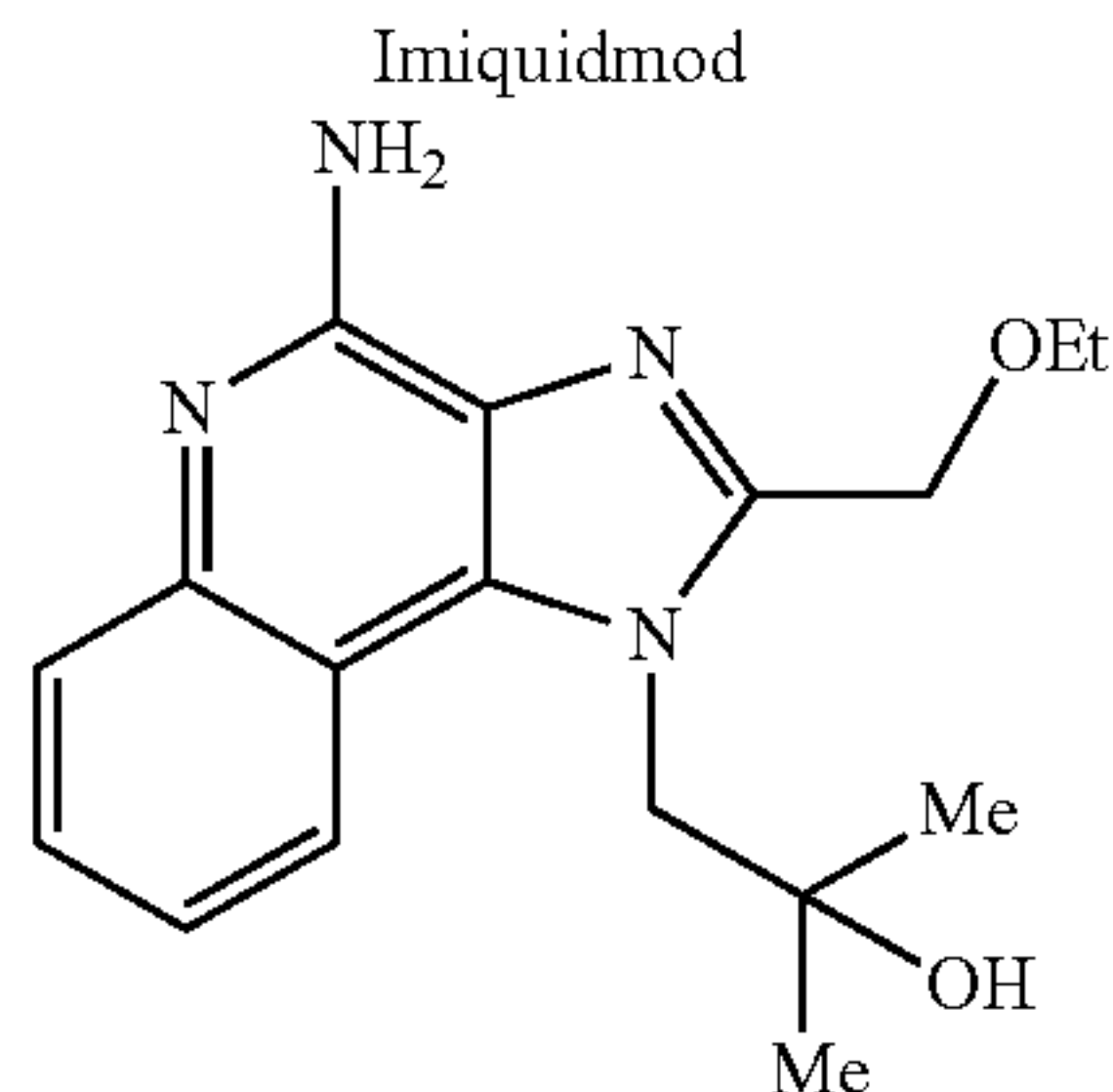
Resiquimod
