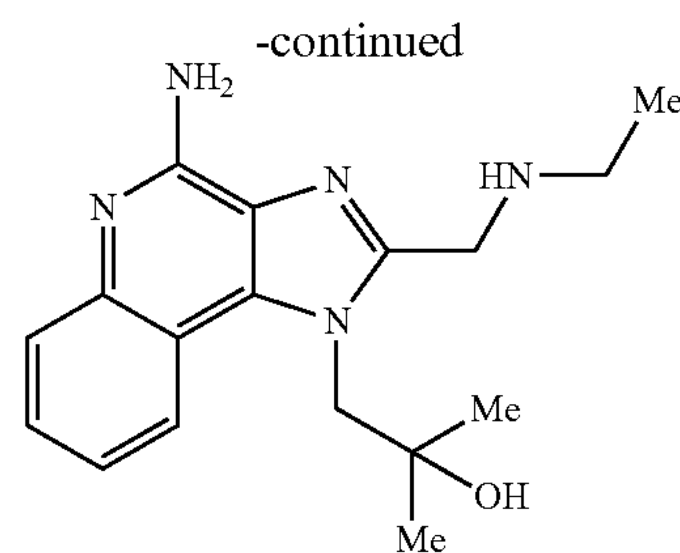
Gardiquimod
