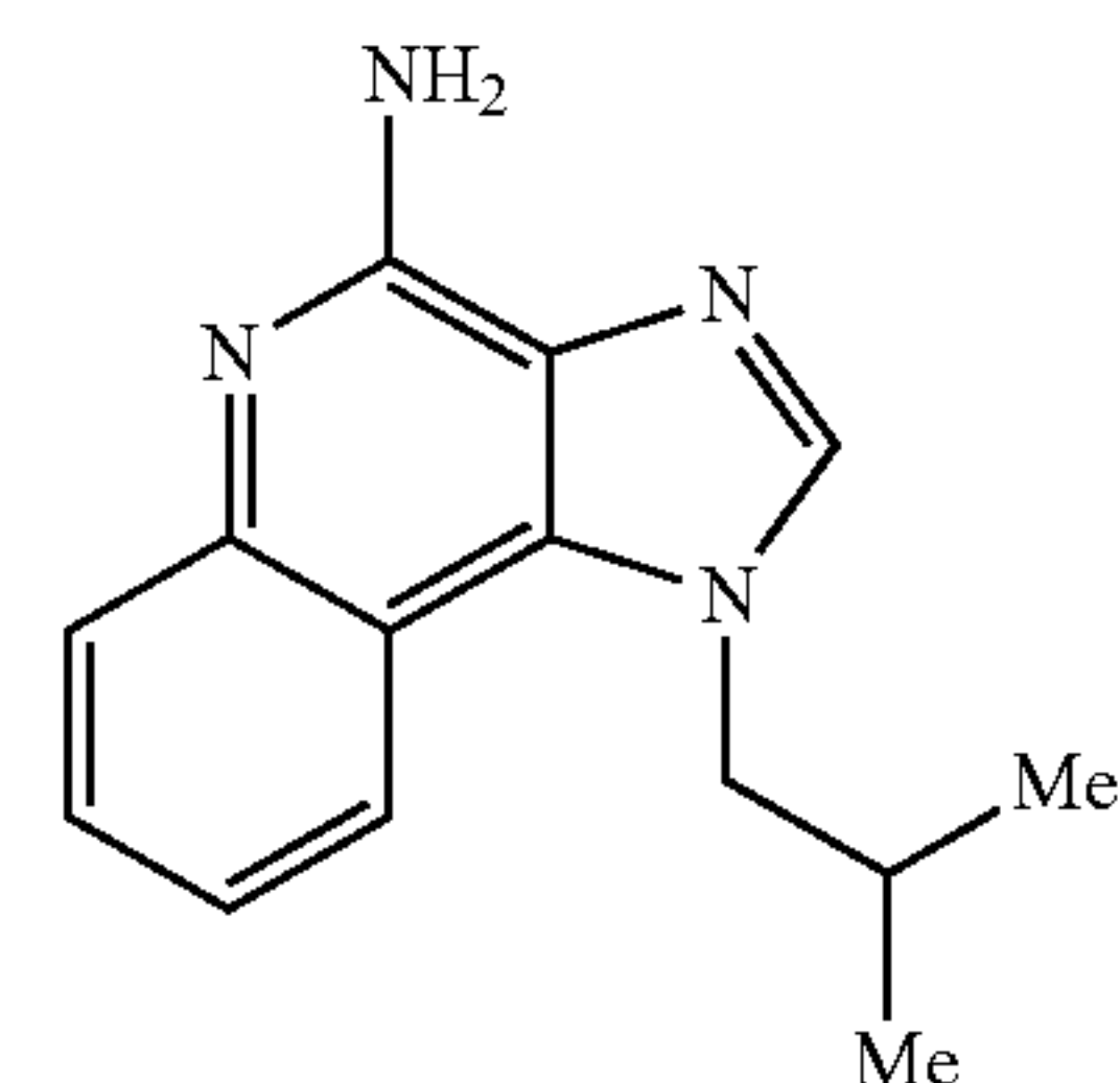
Imiquimod
