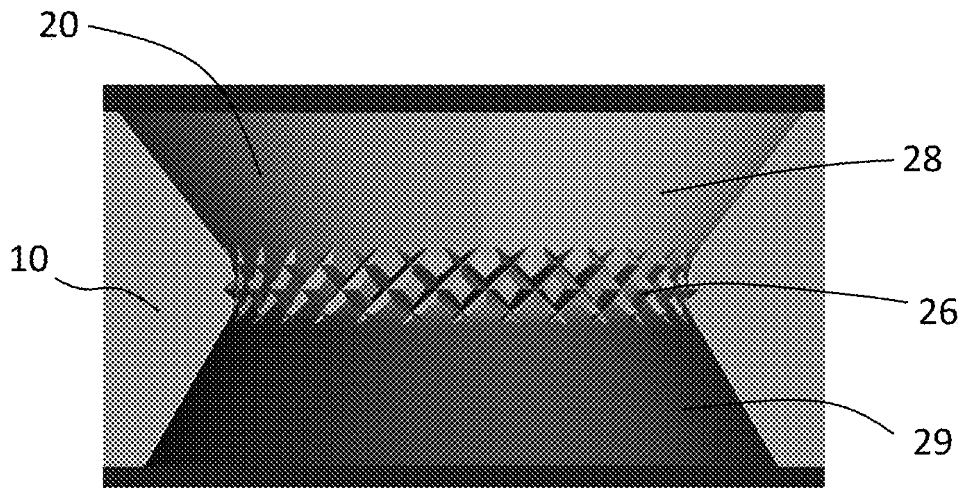
FIG. 18B
