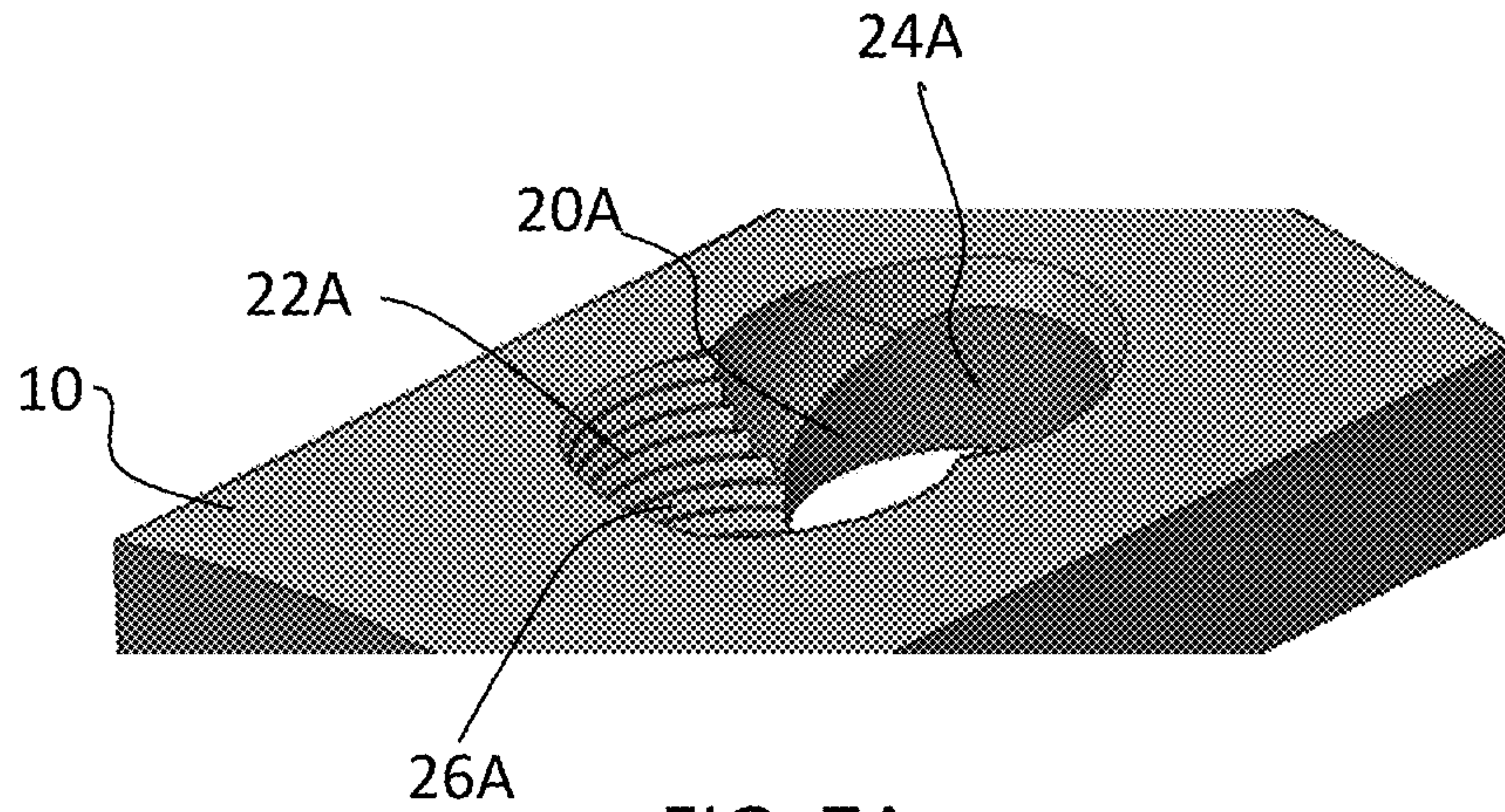
FIG. 7A
