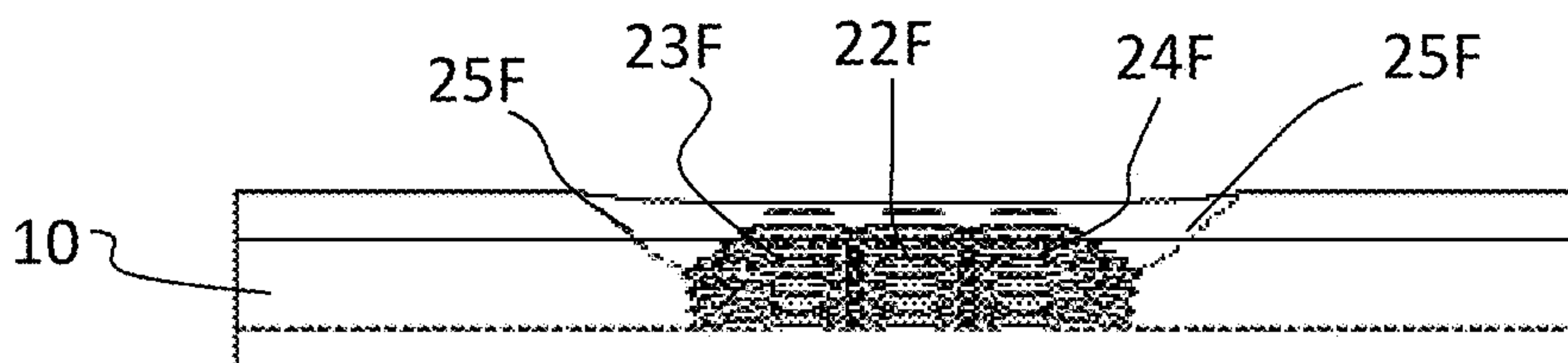
FIG. 12C
