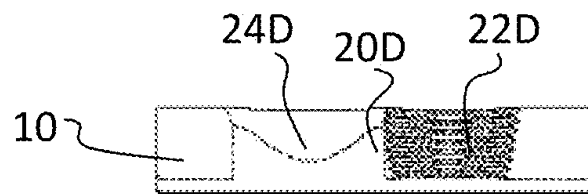
FIG. 10B
