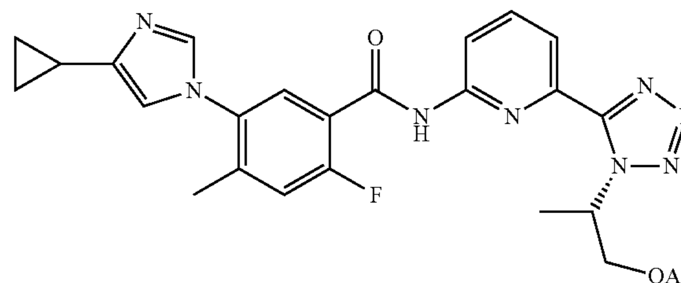
Example 4a
