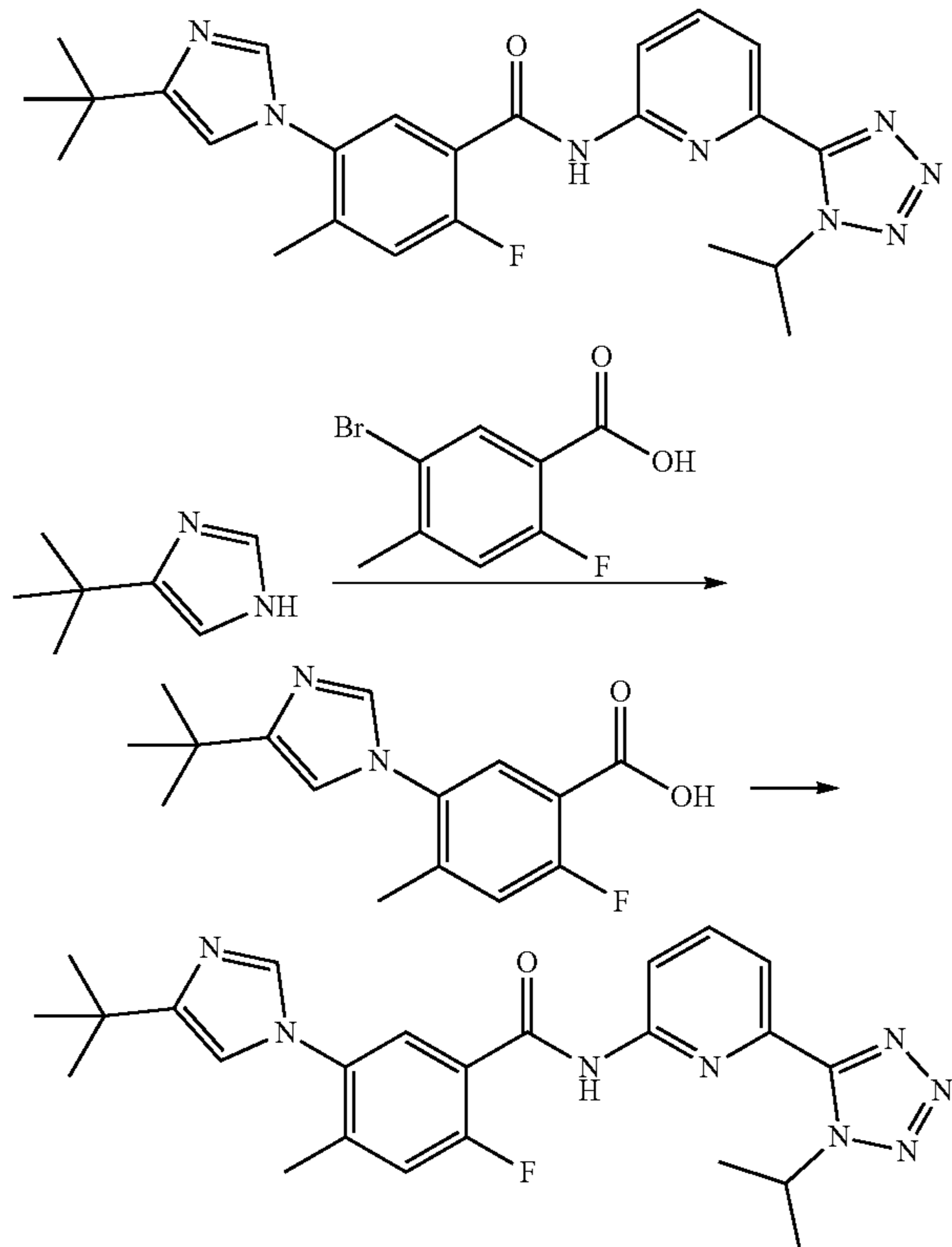
Example 29a
