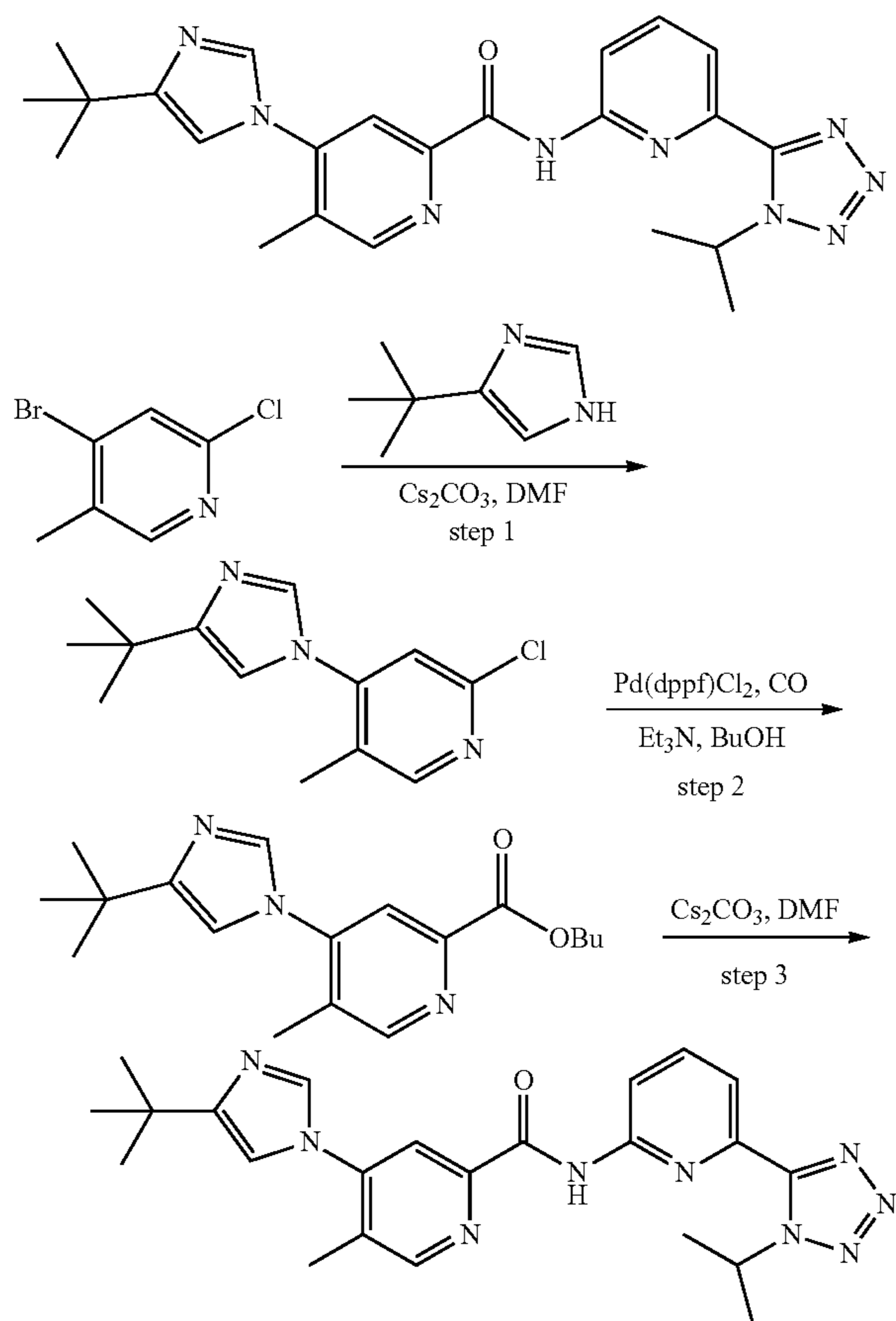
Example 52a
