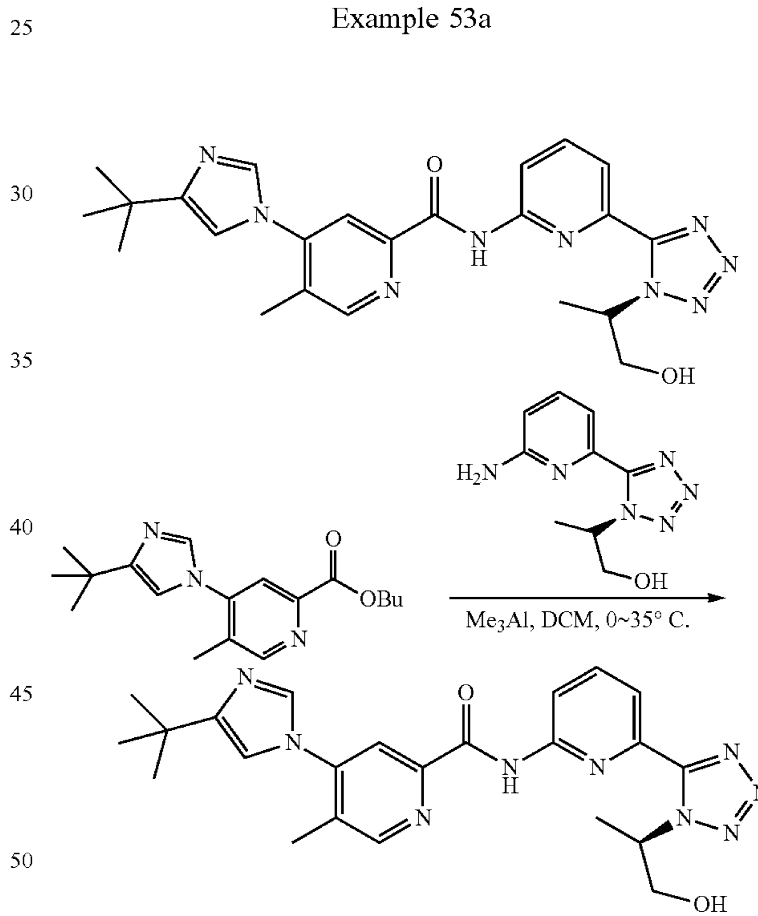
Example 53a
