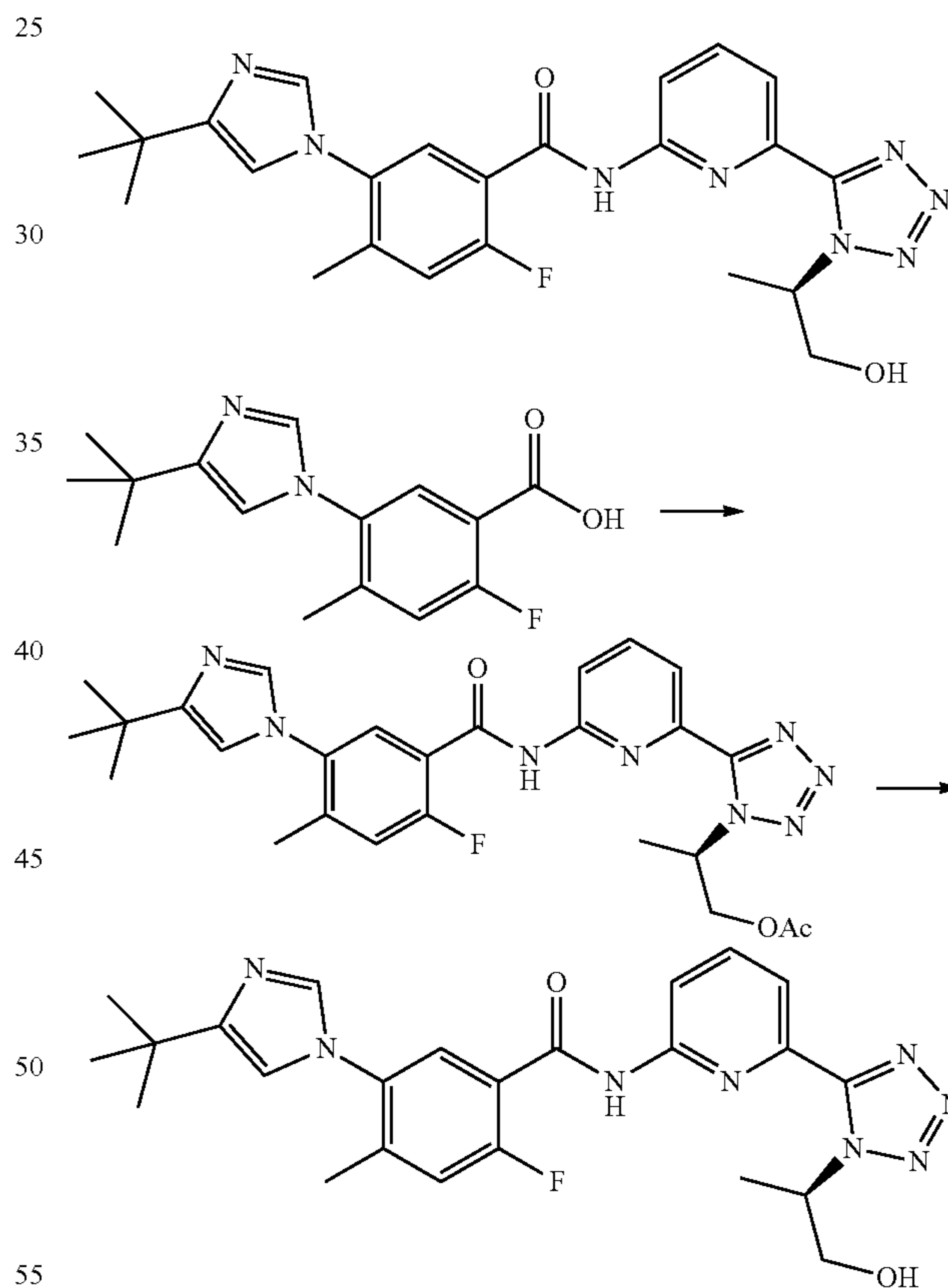
Example 30a
