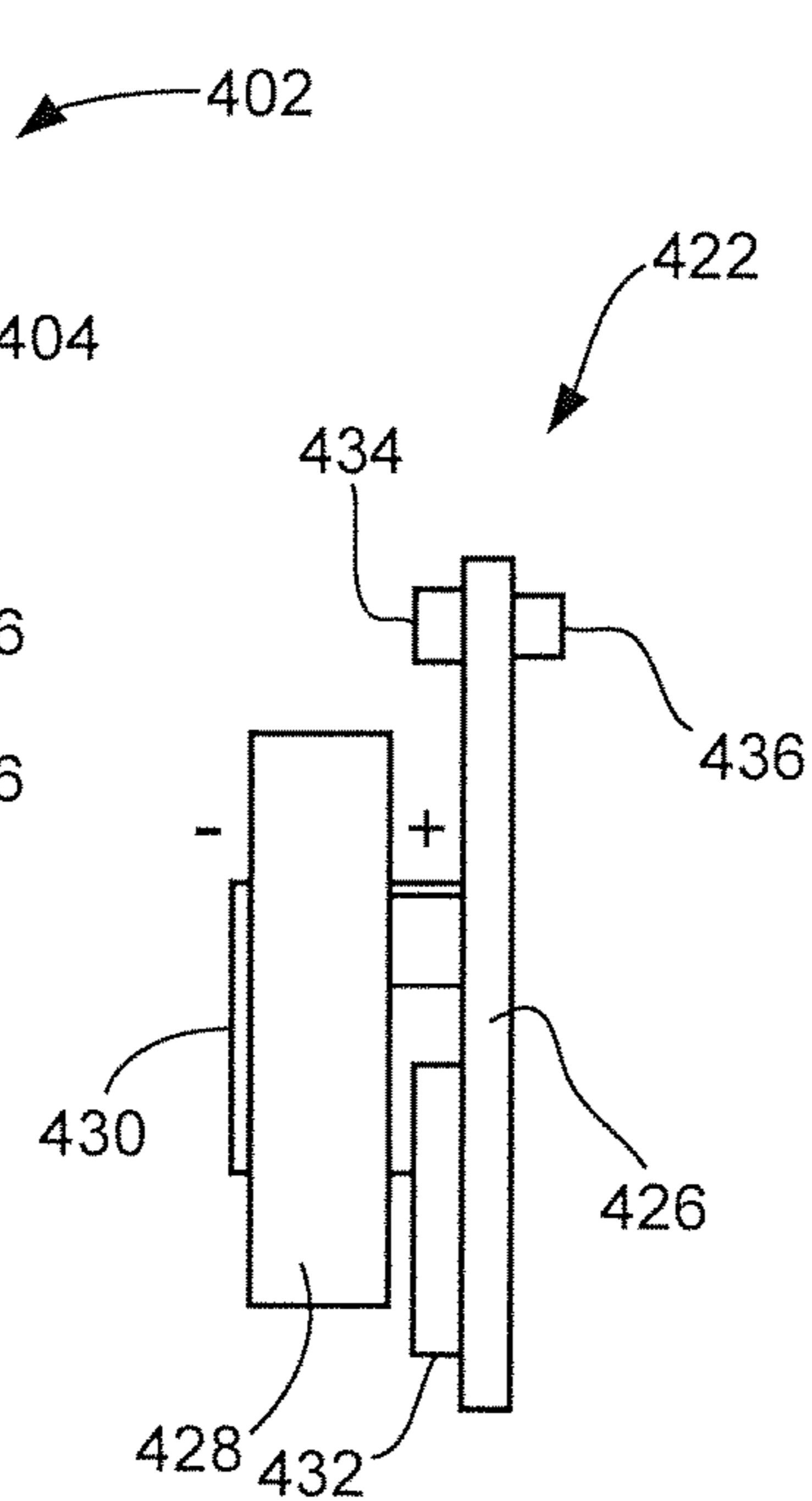
FIG. 28
