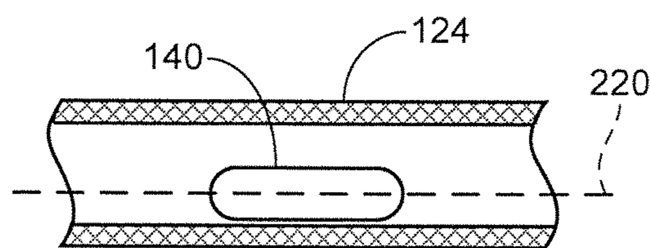
FIG. 10
