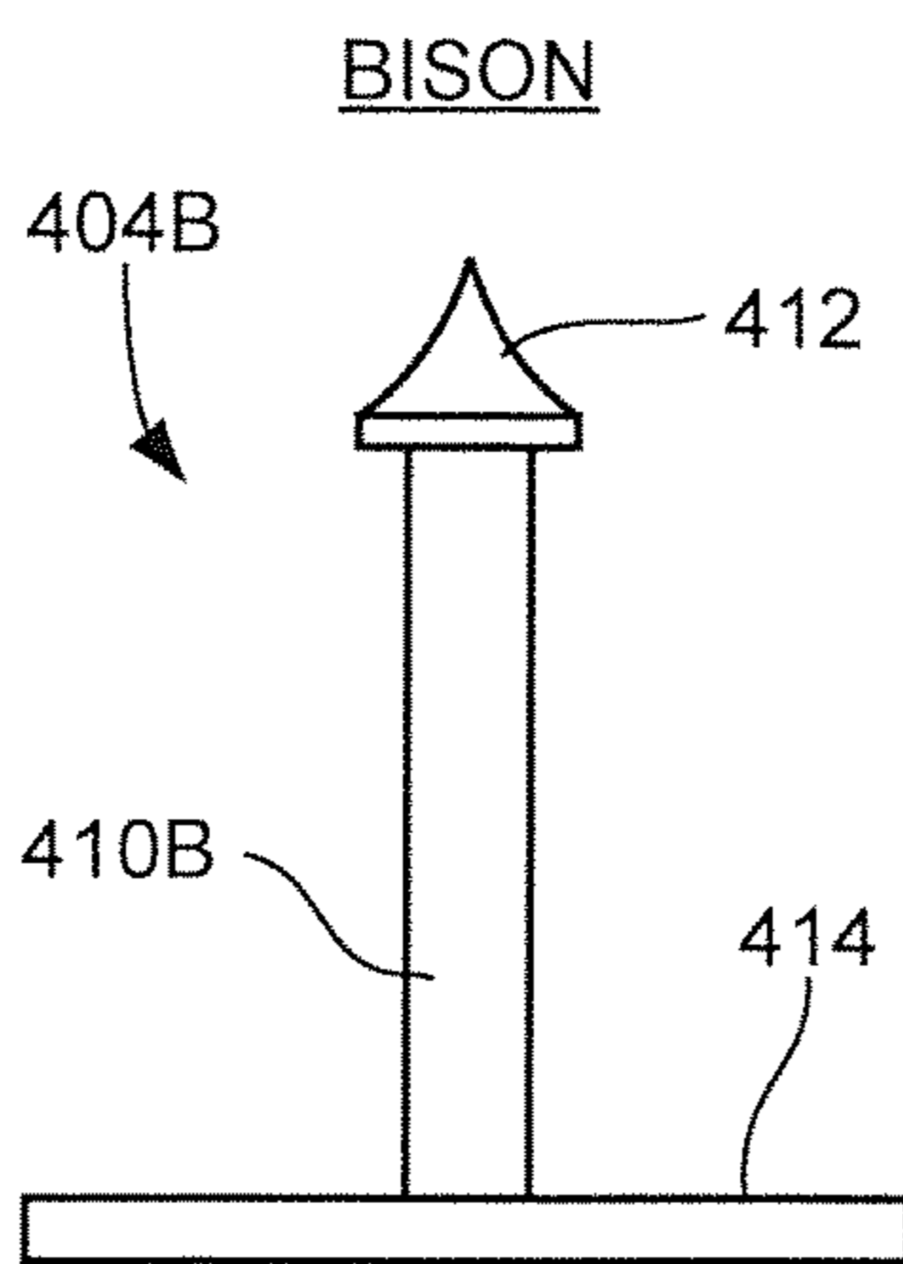
FIG. 30B
