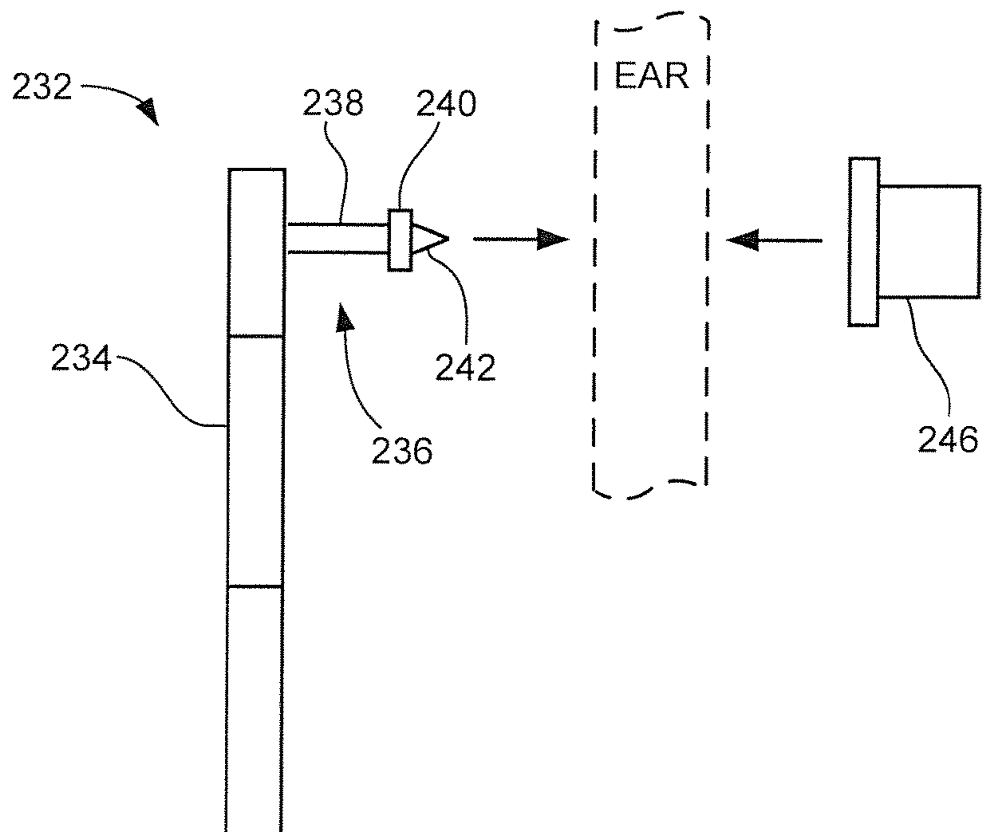
FIG. 14B
