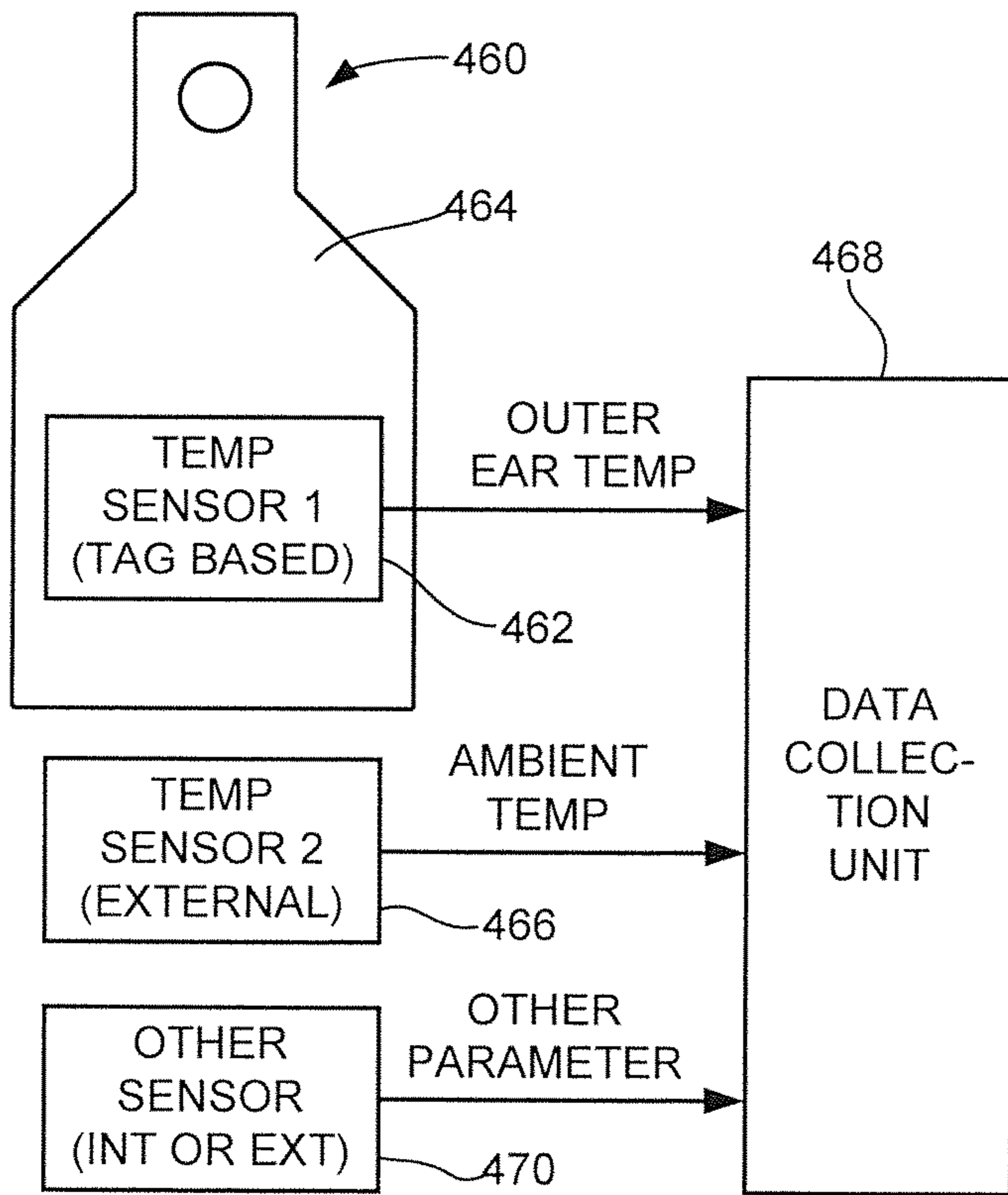
FIG. 33
