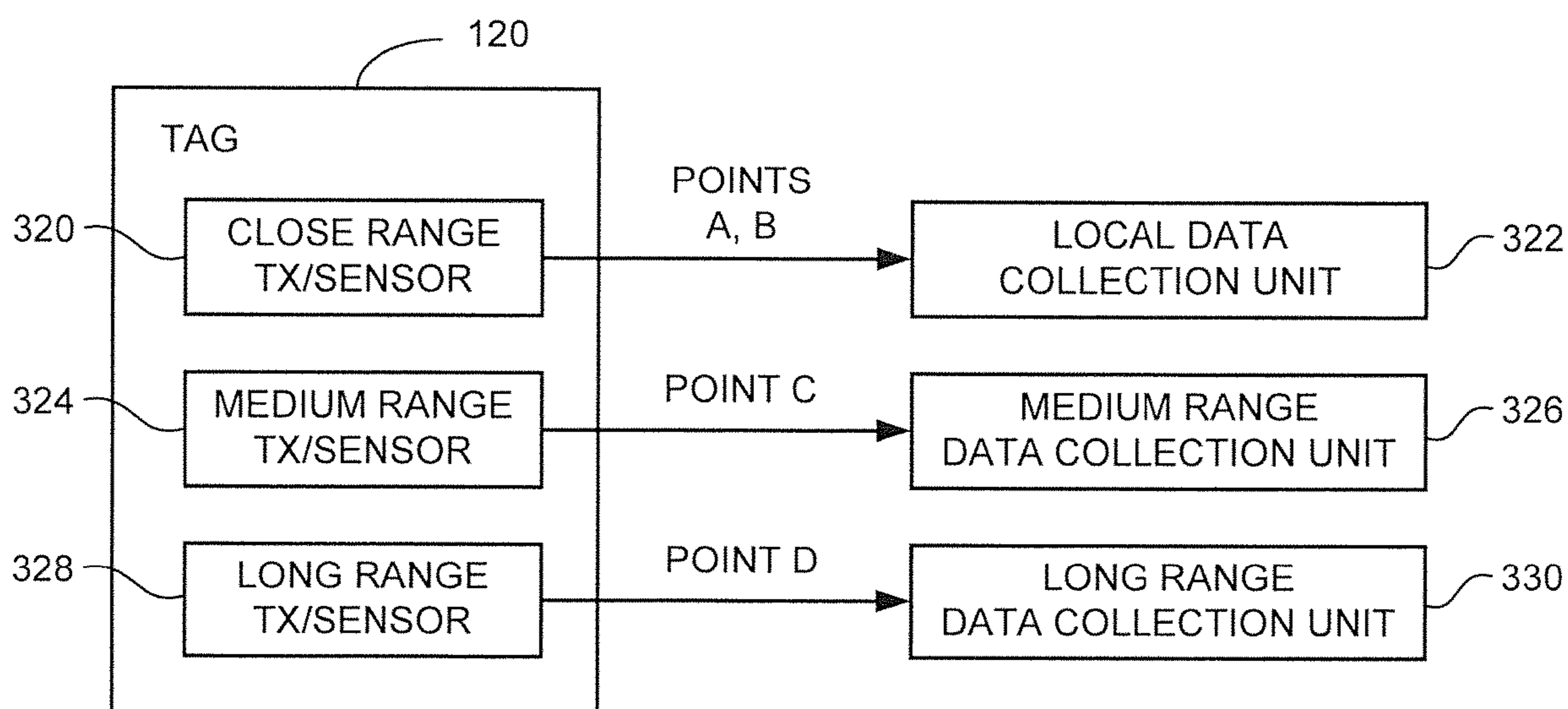
FIG. 23
