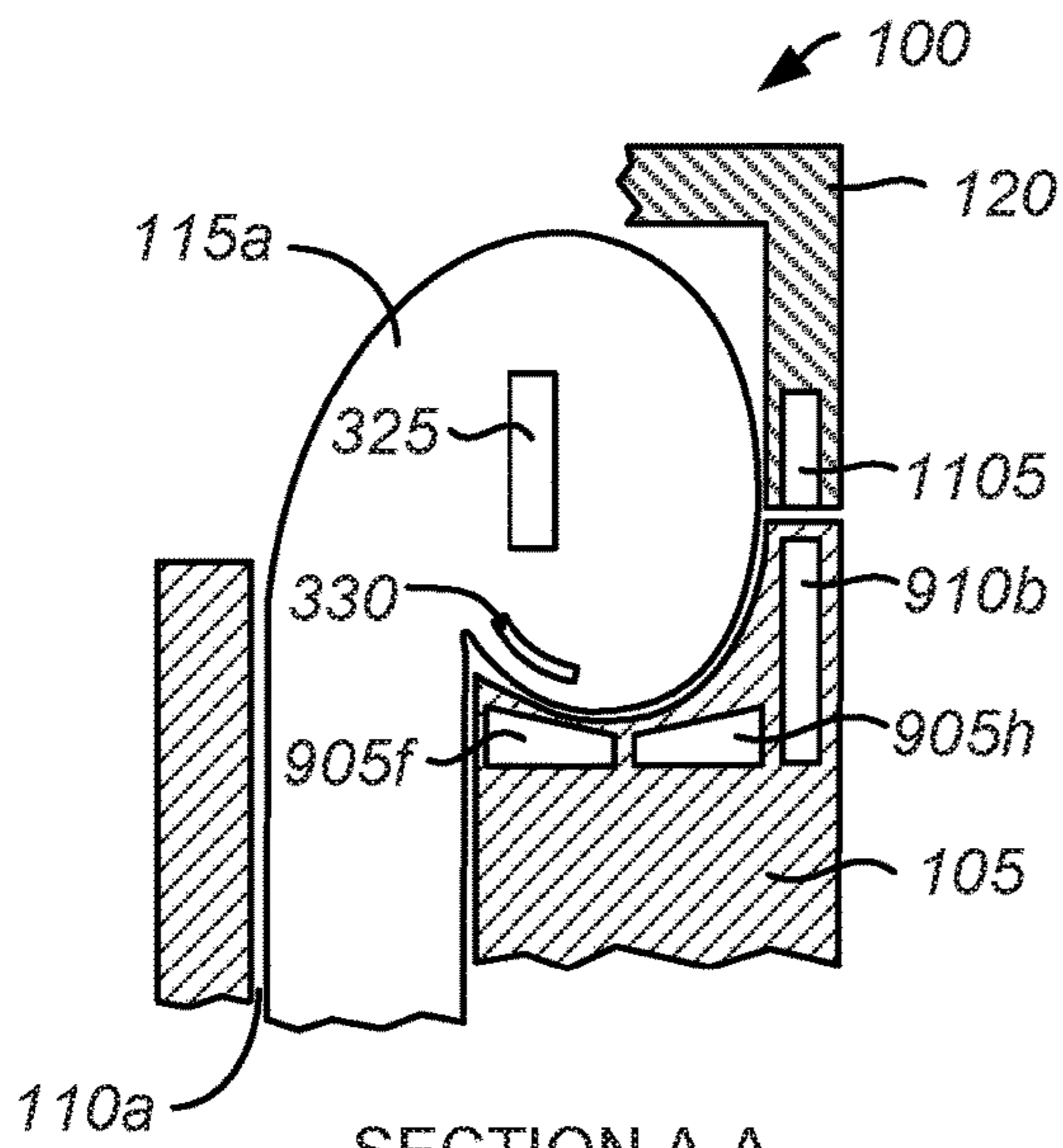
SECTION A-A
