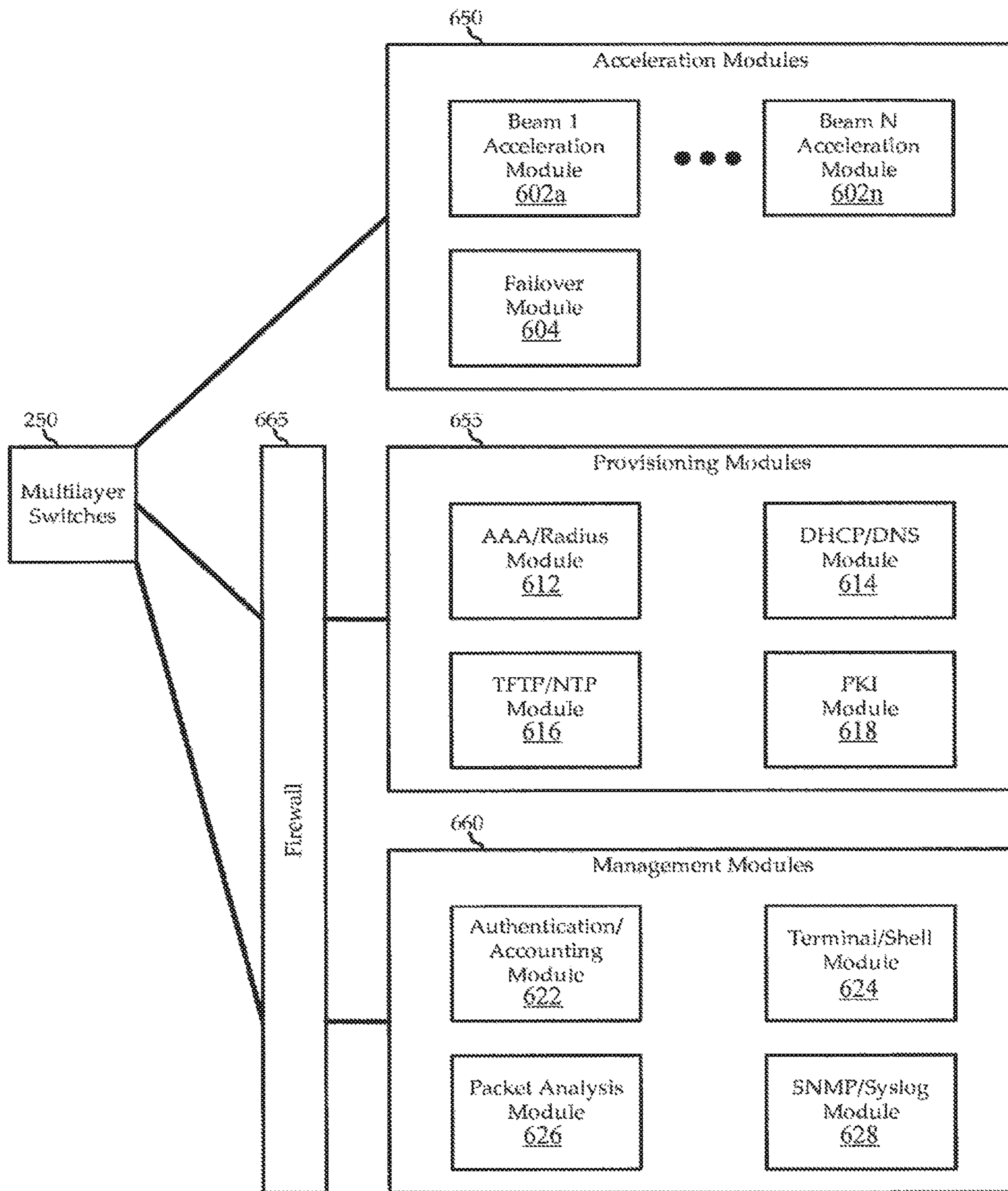
FIG. 6B
