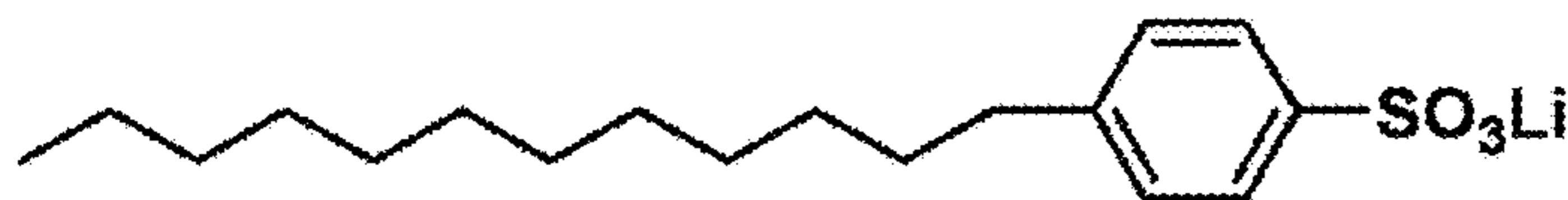
lithium 4-dodecylbenzenesulfonate
