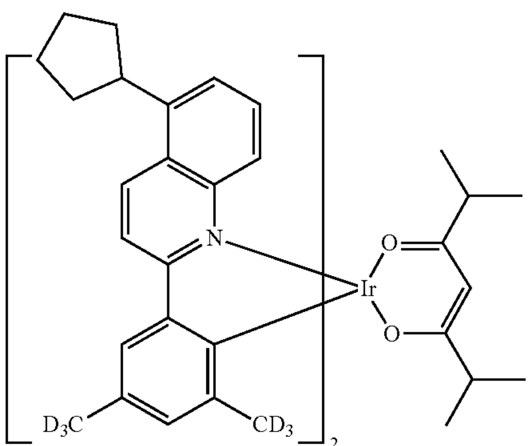
Compound II-43
