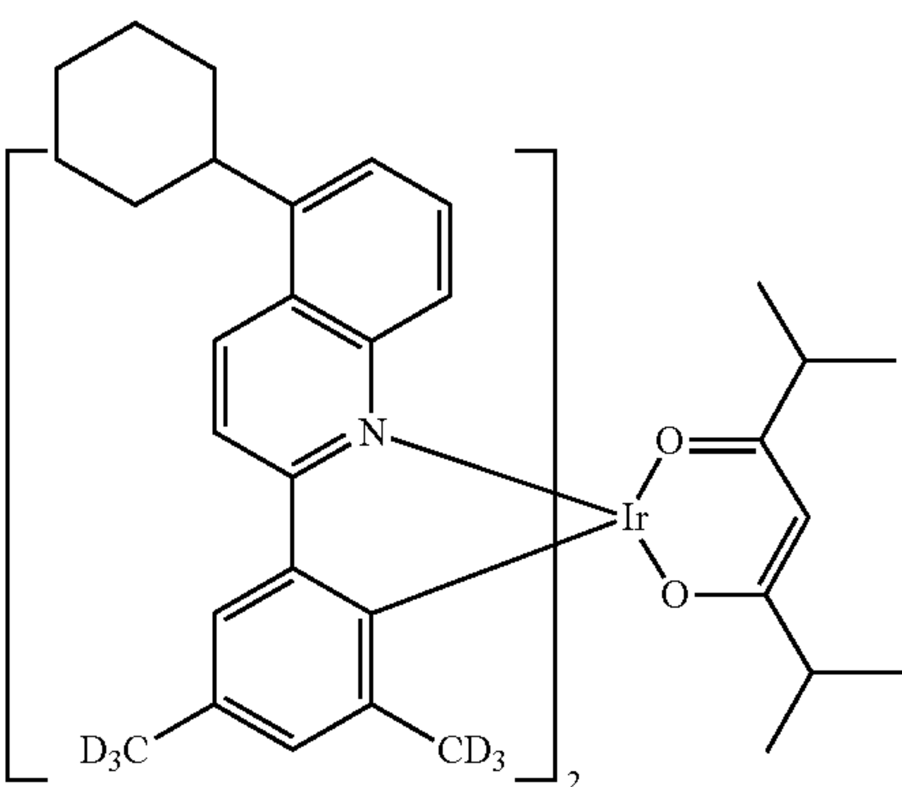
Compound II-43
