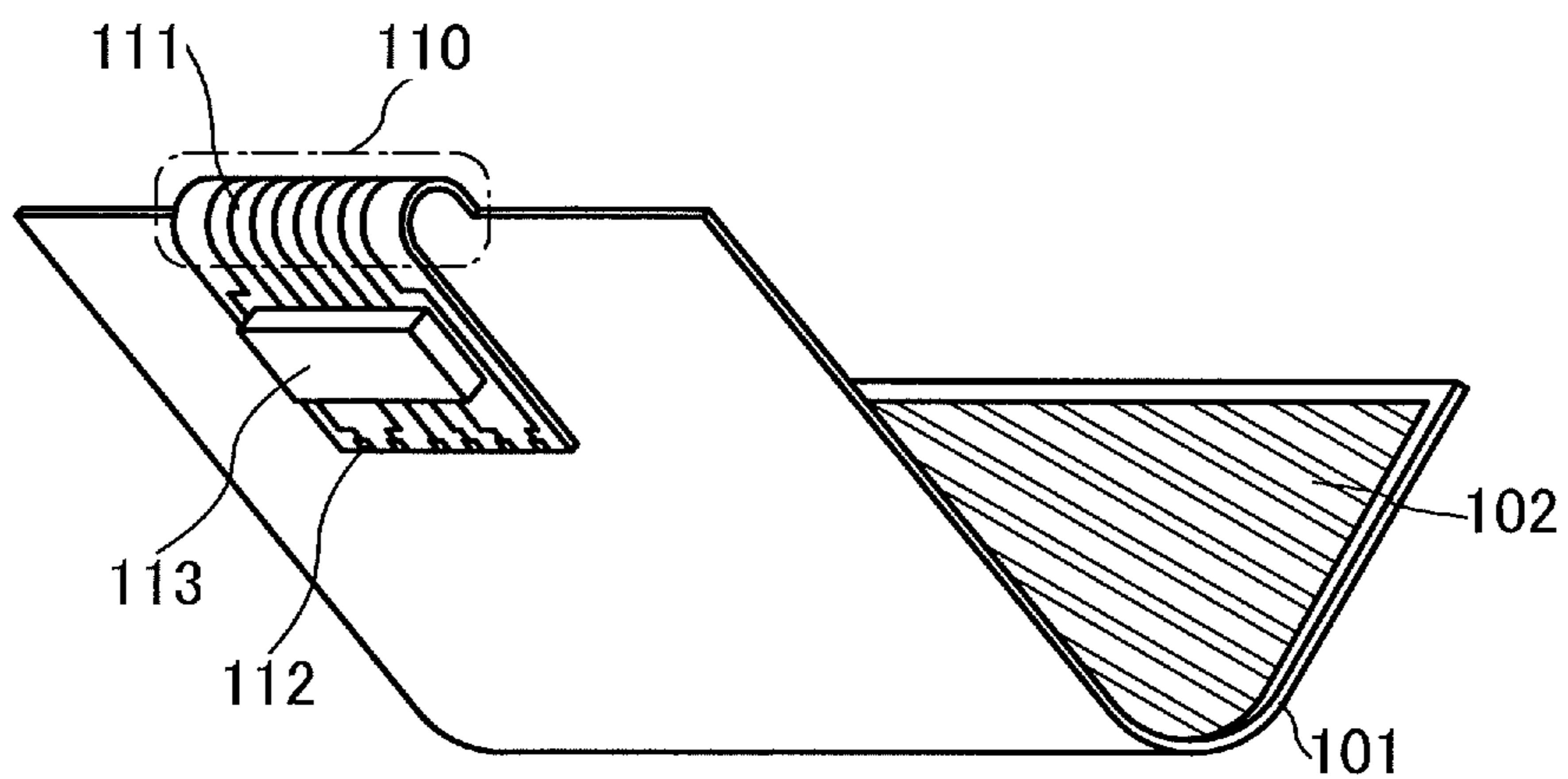
FIG. 1B
