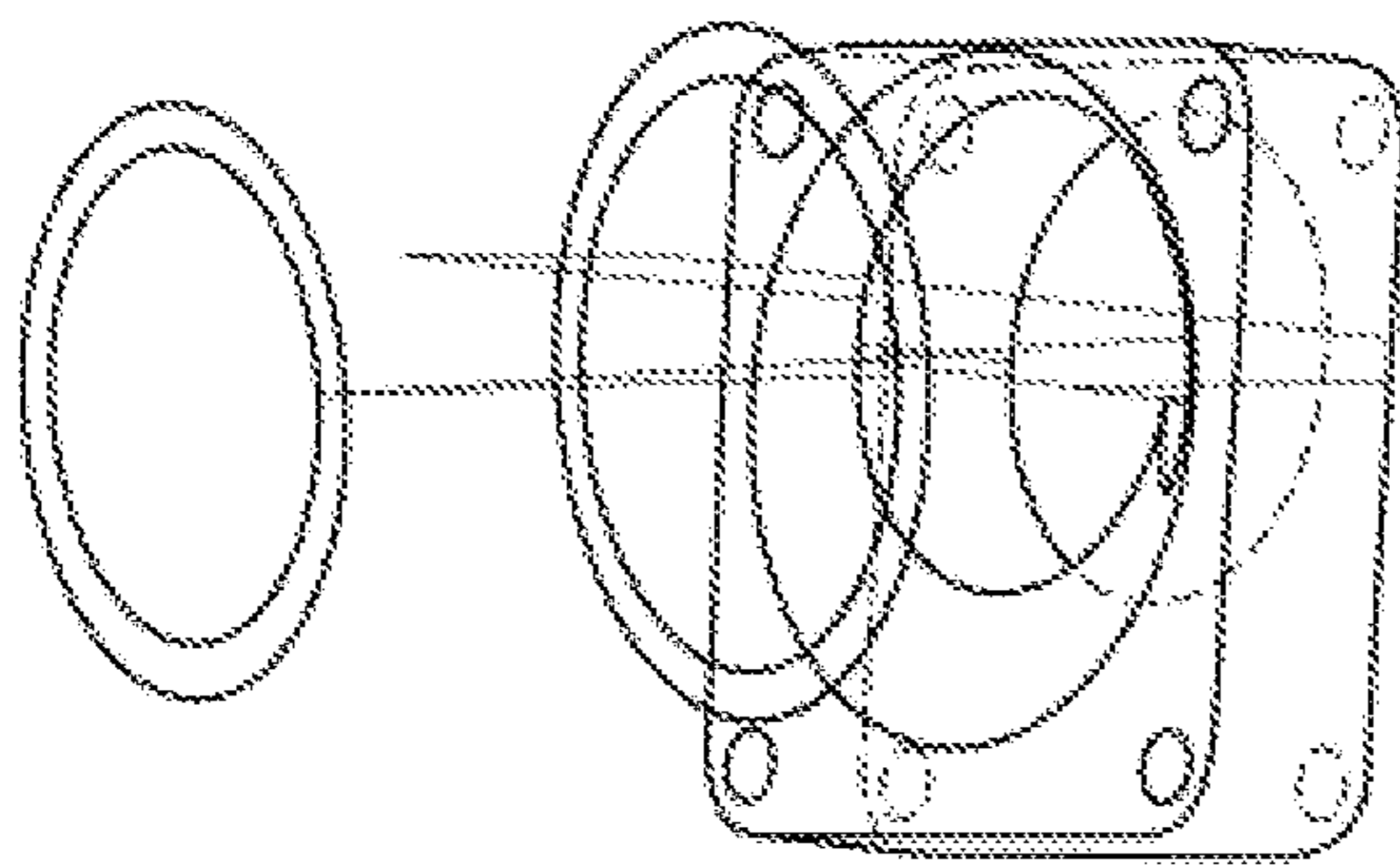
FIG. 18C
