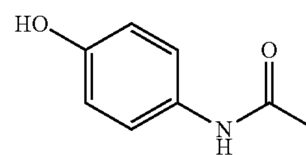
Acet
