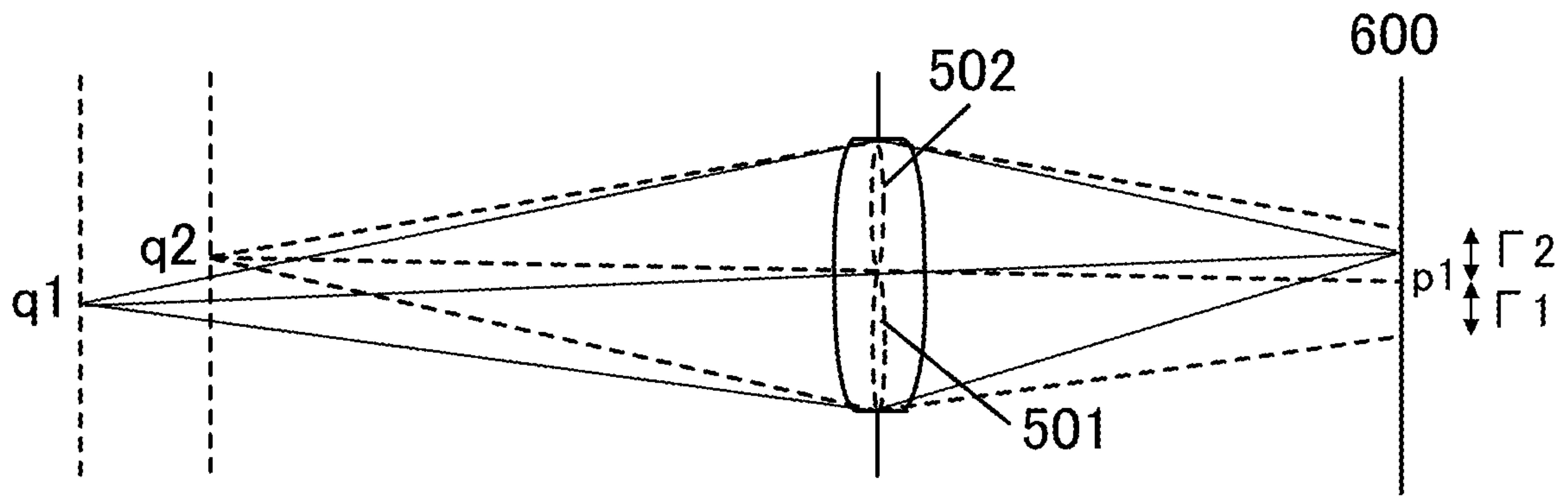
FIG. 8A
