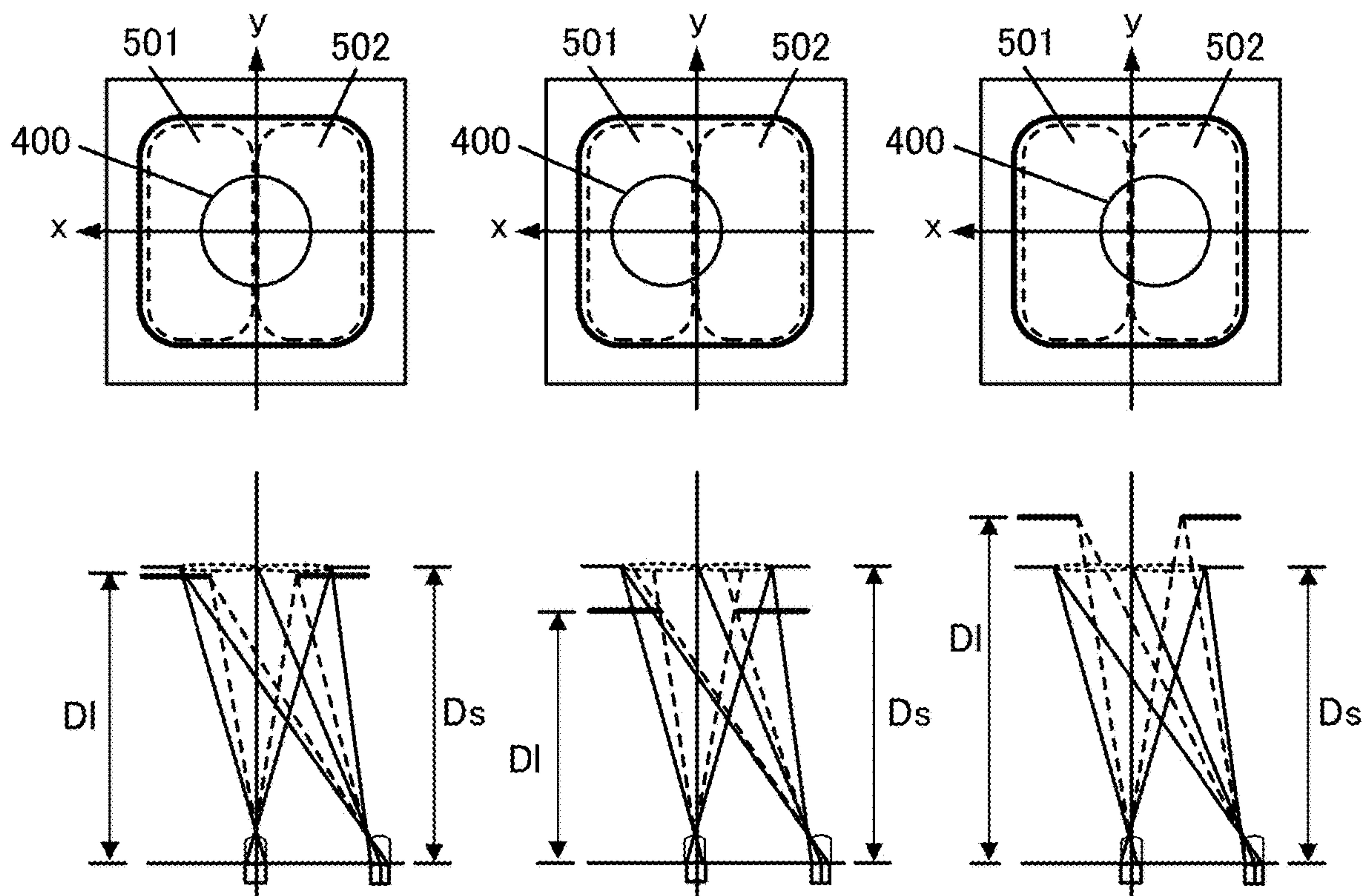
FIG. 10A
