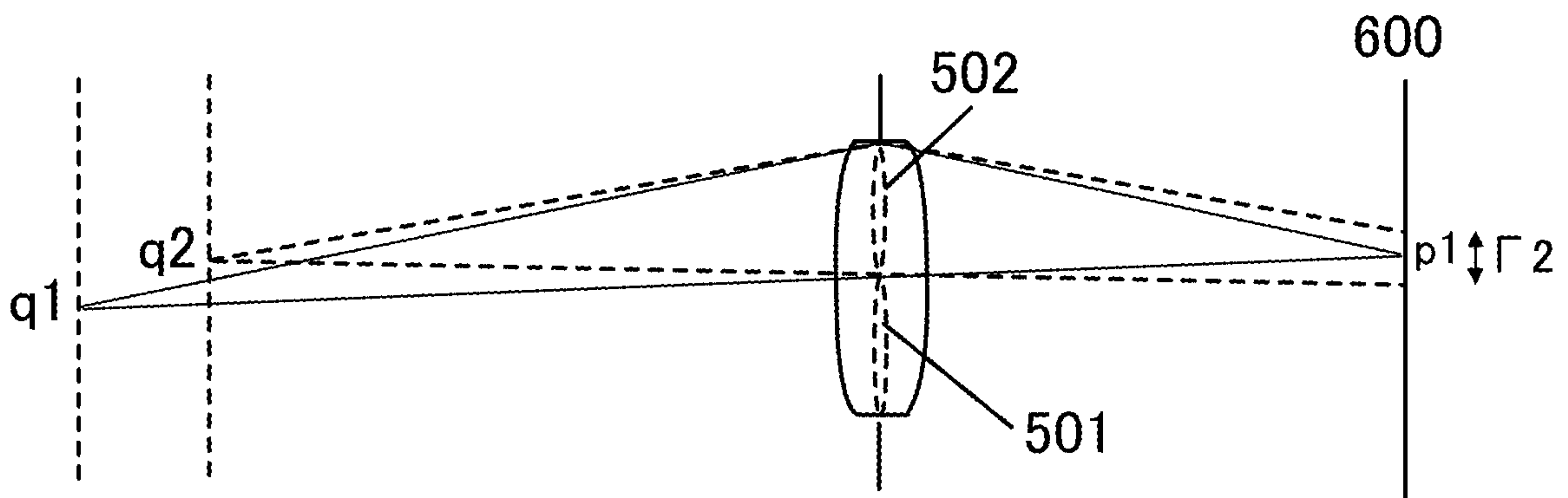
FIG. 8C
