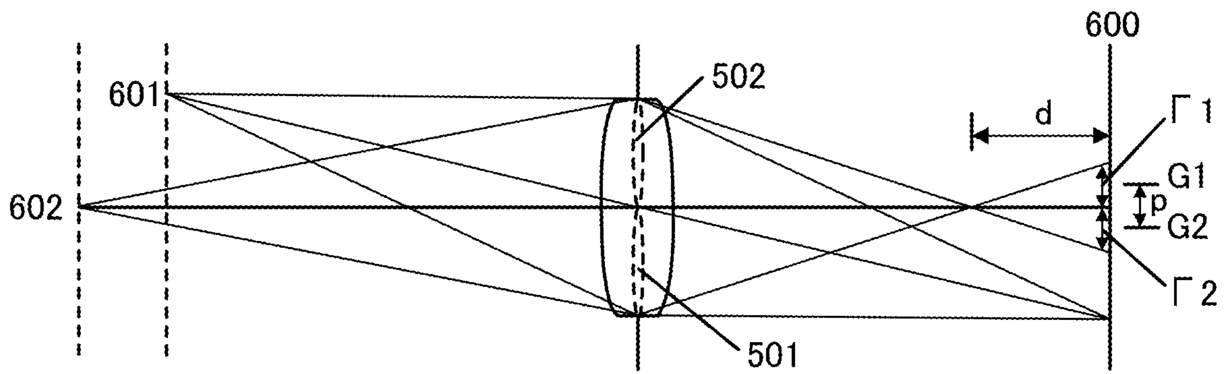
FIG. 6
