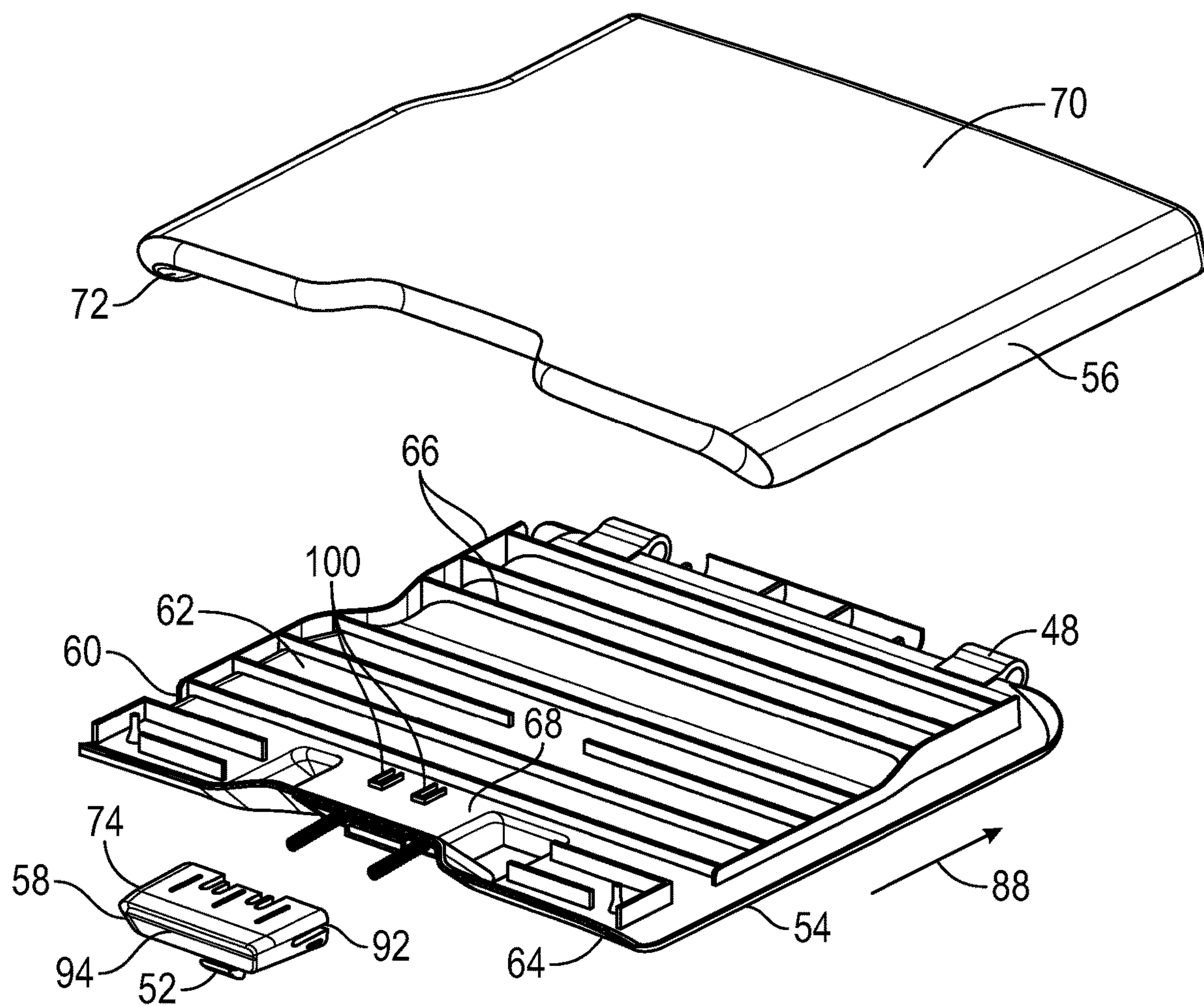
FIG. 7
