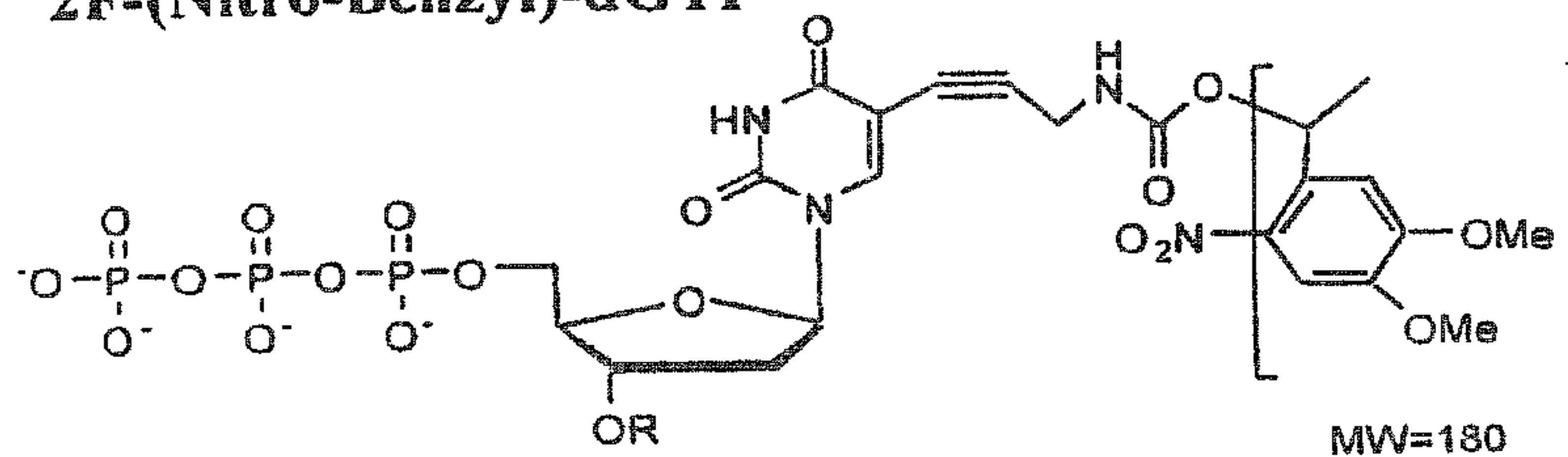
2(Meo)-(Nitro-Benzyl)-dTTP
