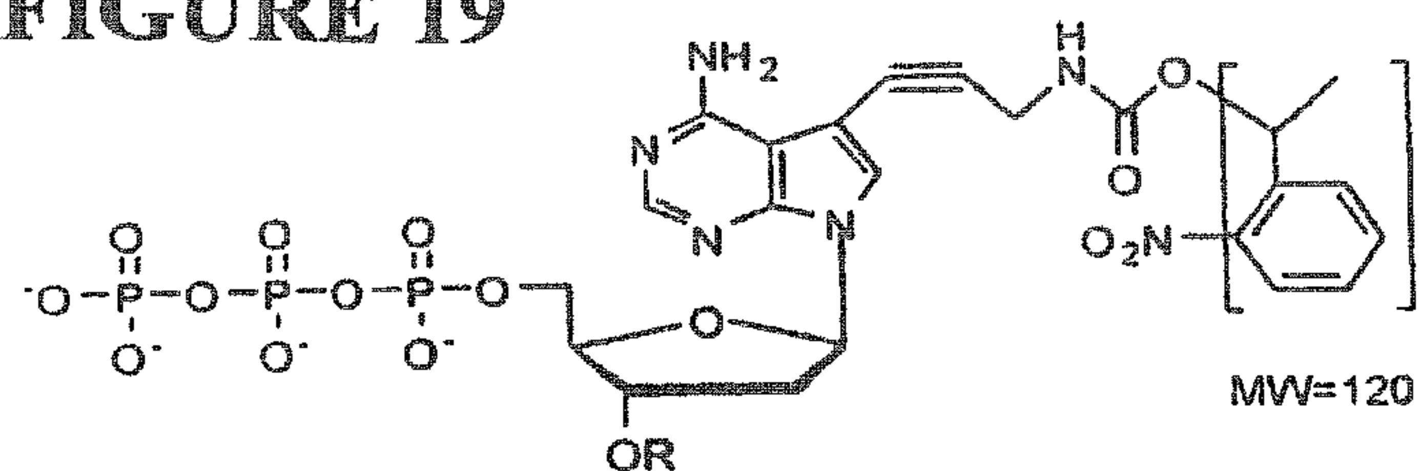
(Nitro-Benzyl)-dATP
