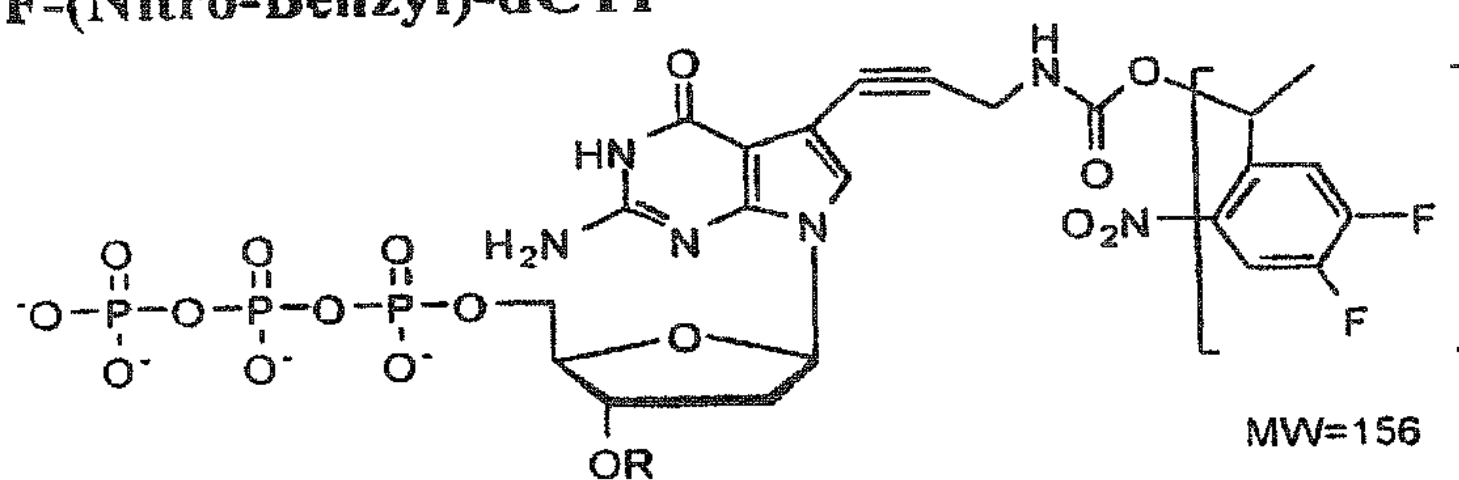
2F-(Nitro-Benzyl)-dGTP
