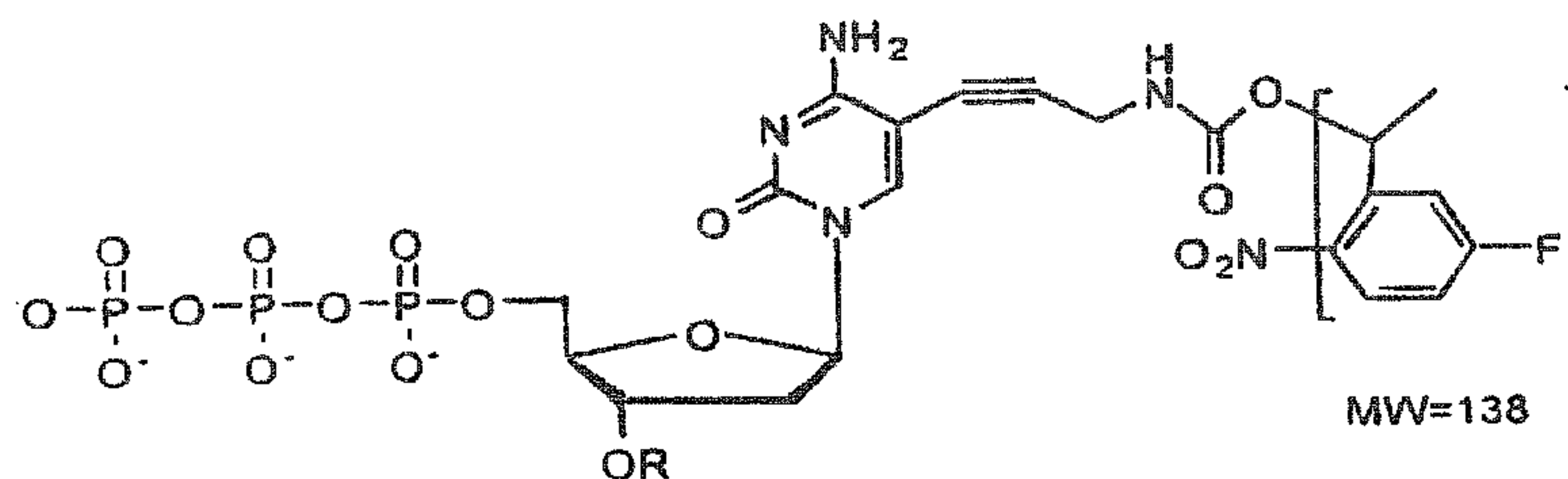
F-(Nitro-Benzyl)-dCTP
