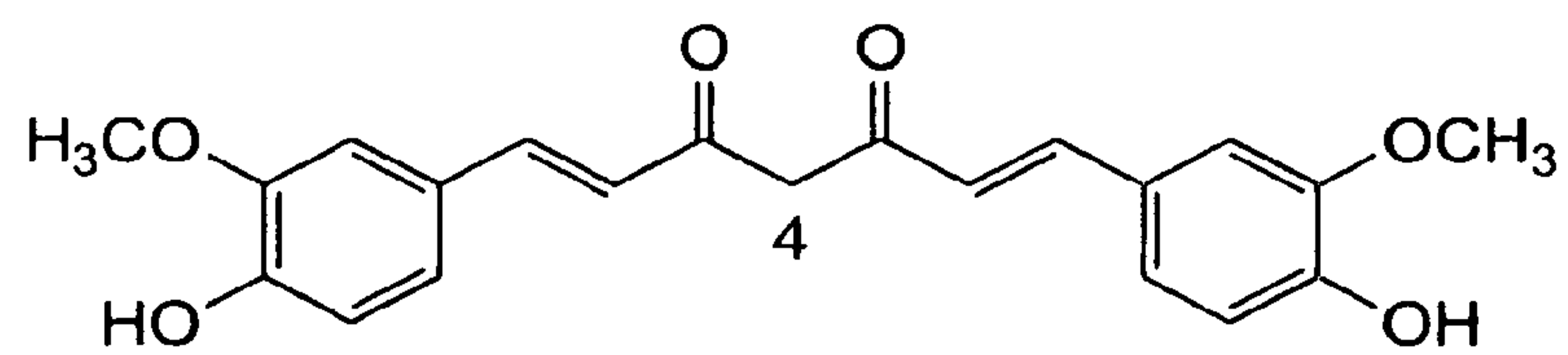
Curcumin
