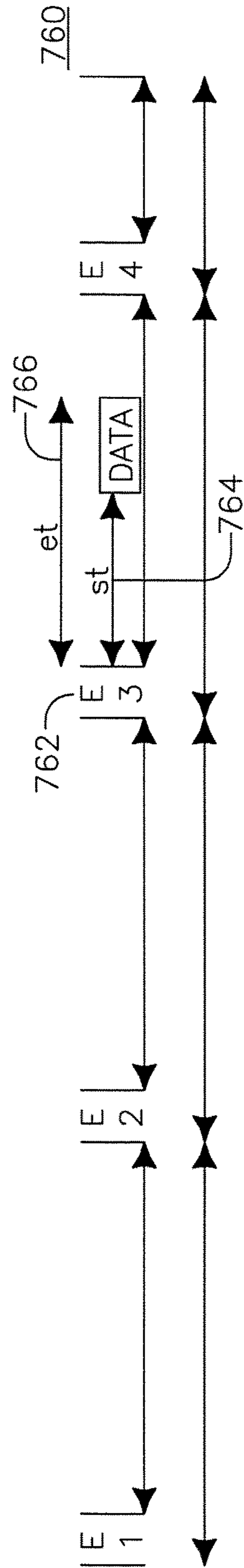
FIG. 7C
