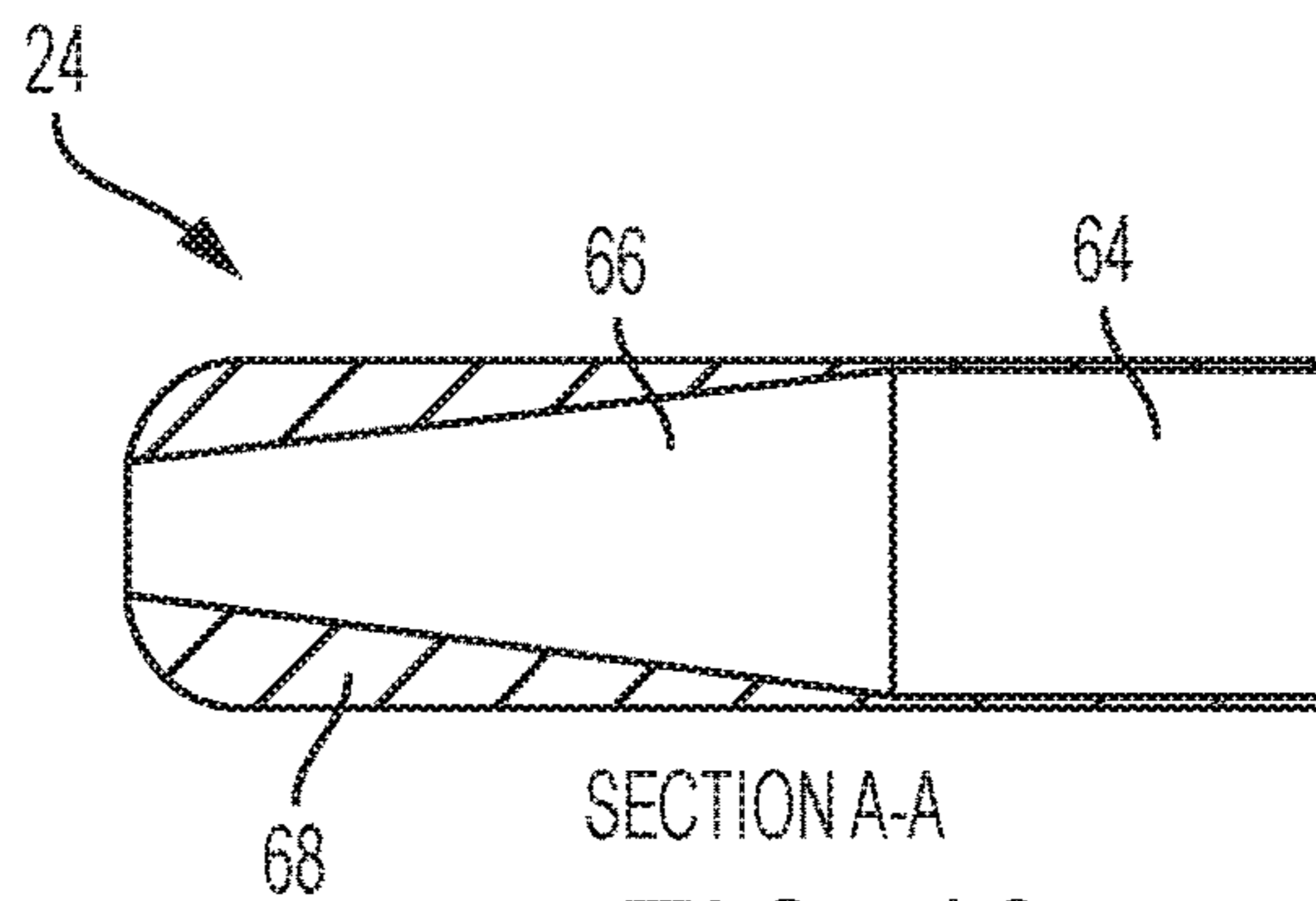
SECTION A-A FIG. 13
