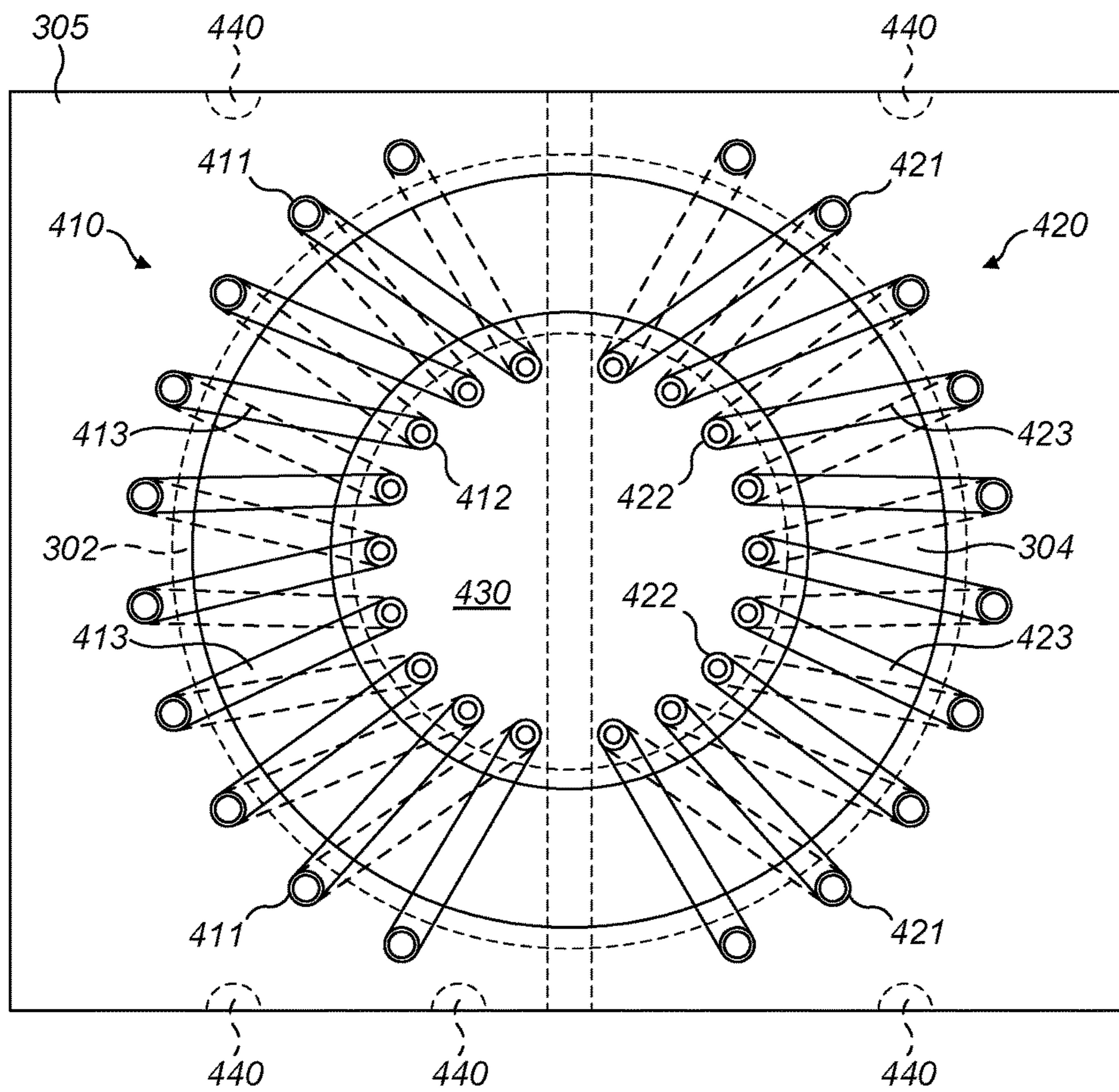
FIG. 4C
