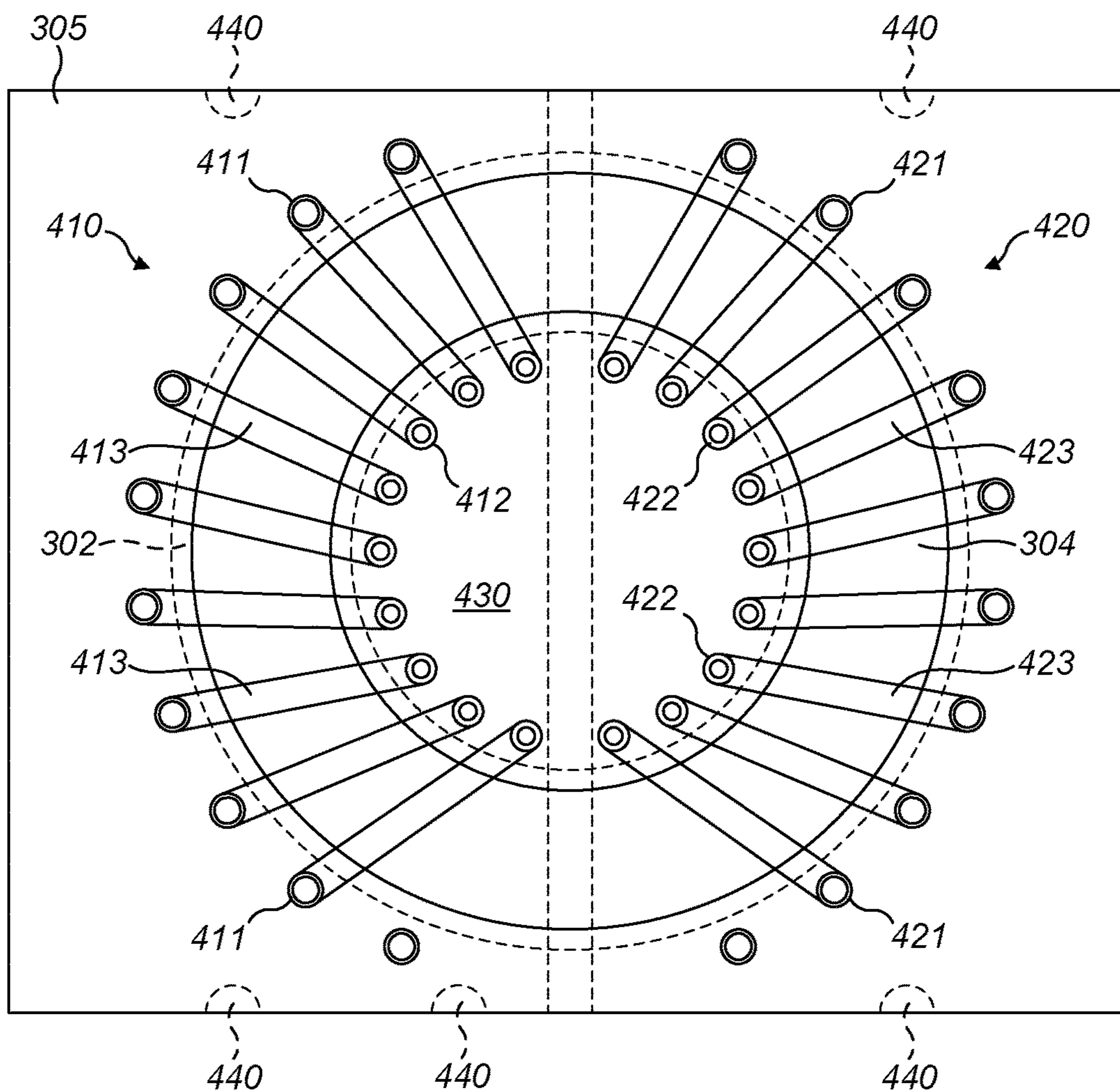
FIG. 4B
