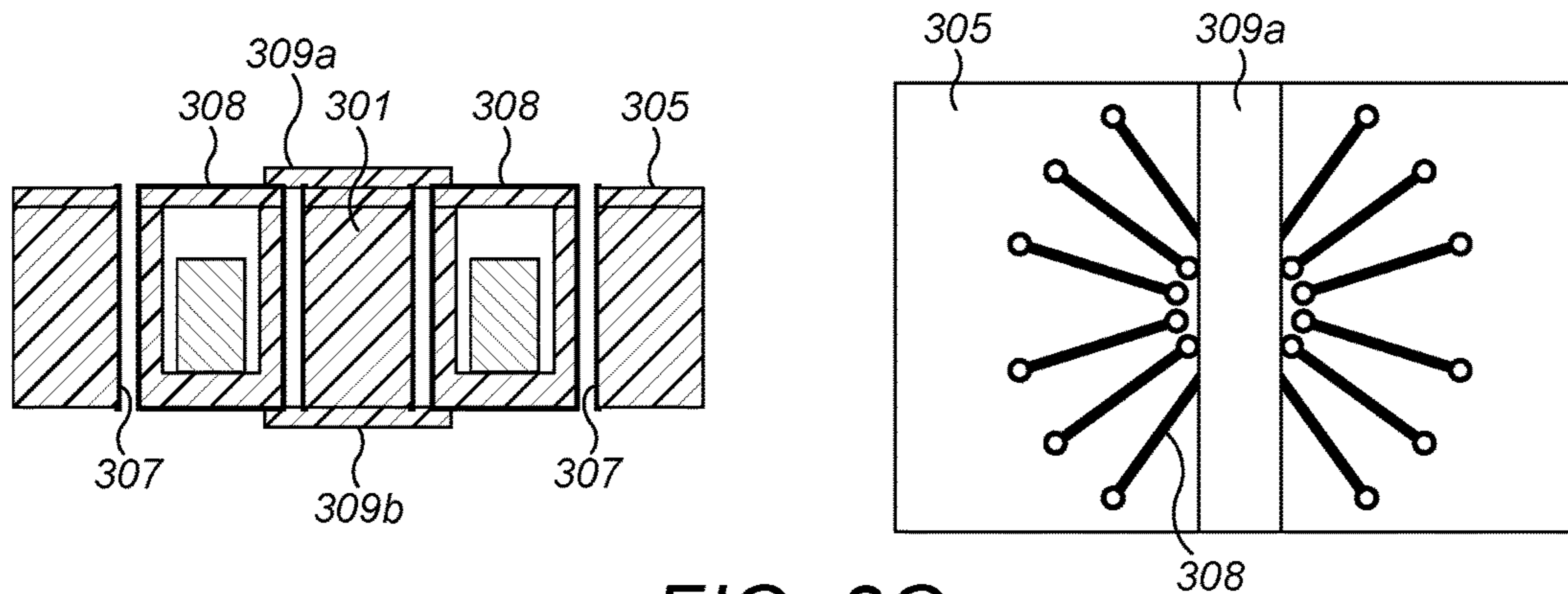
FIG. 3G
