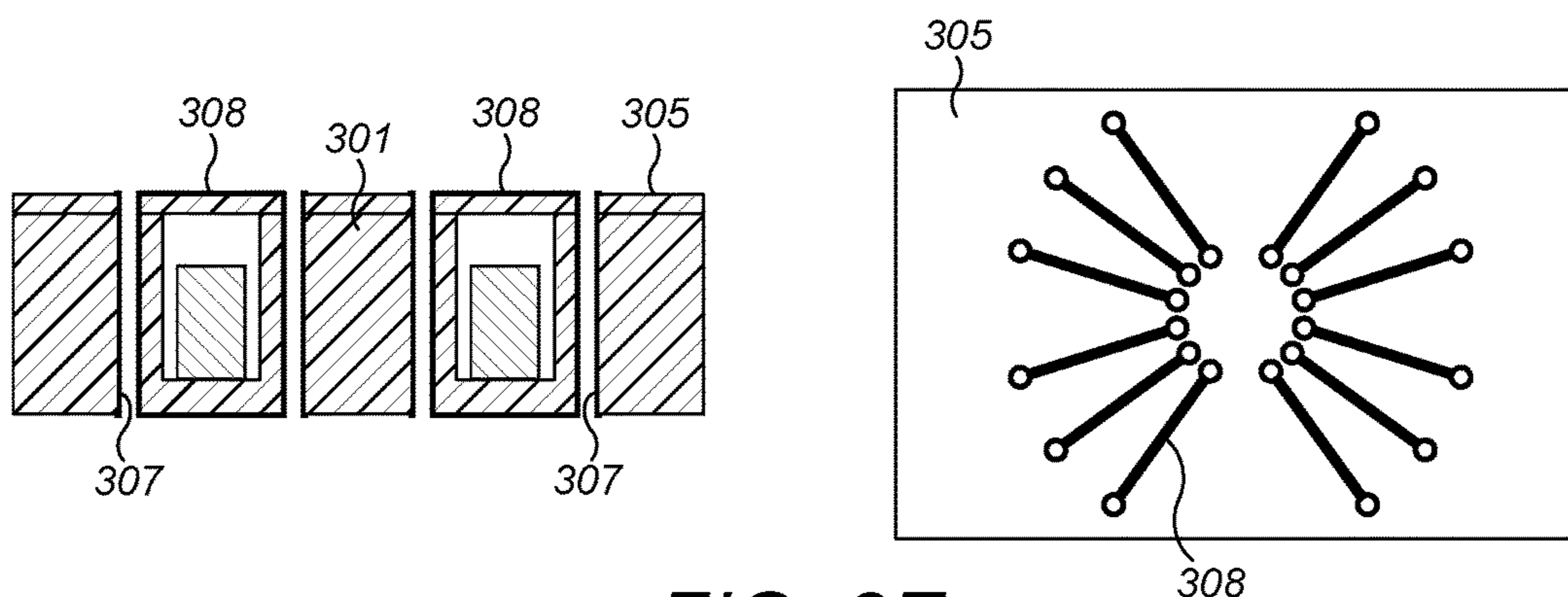
FIG. 3E
