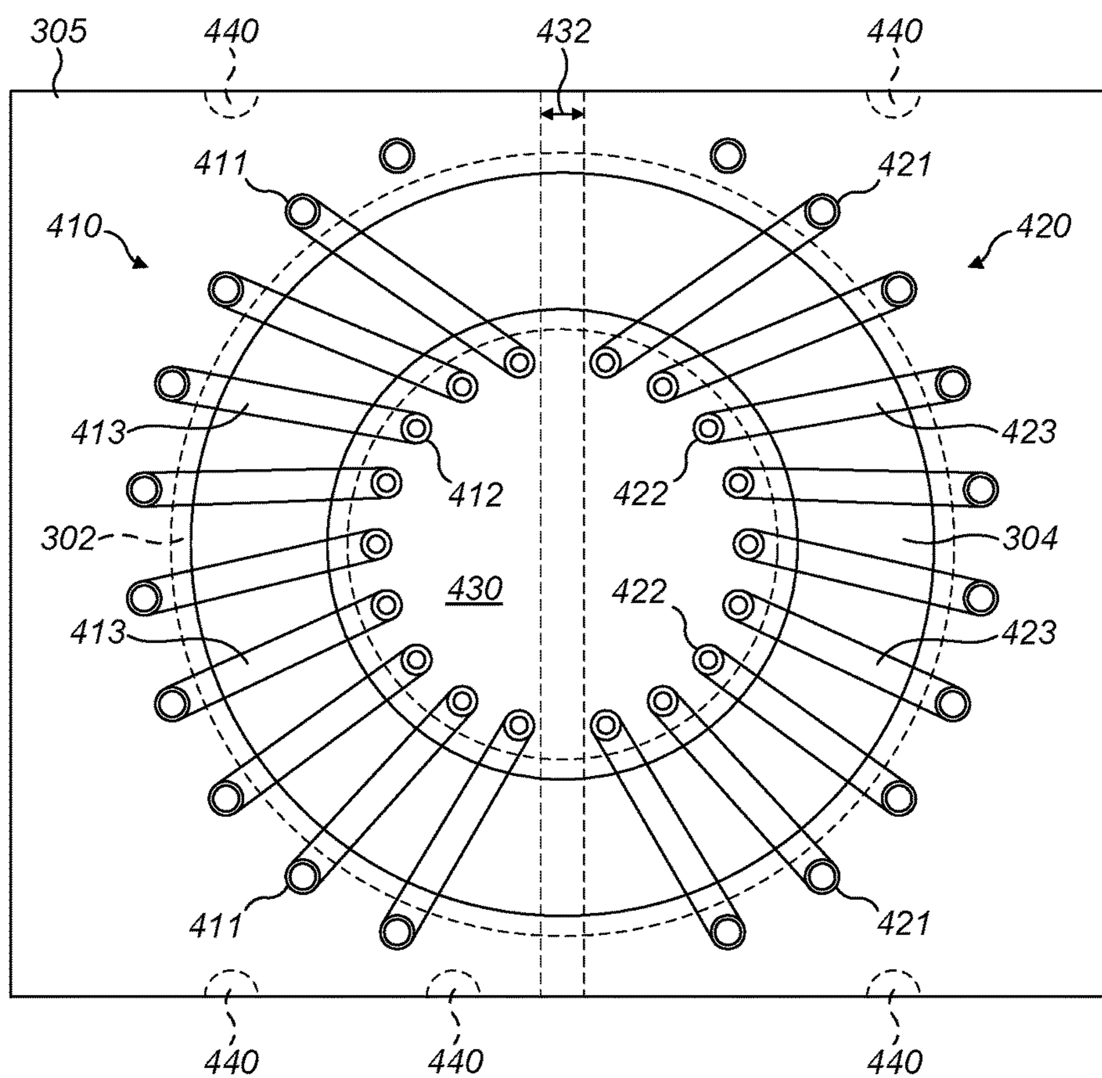
FIG. 4A
