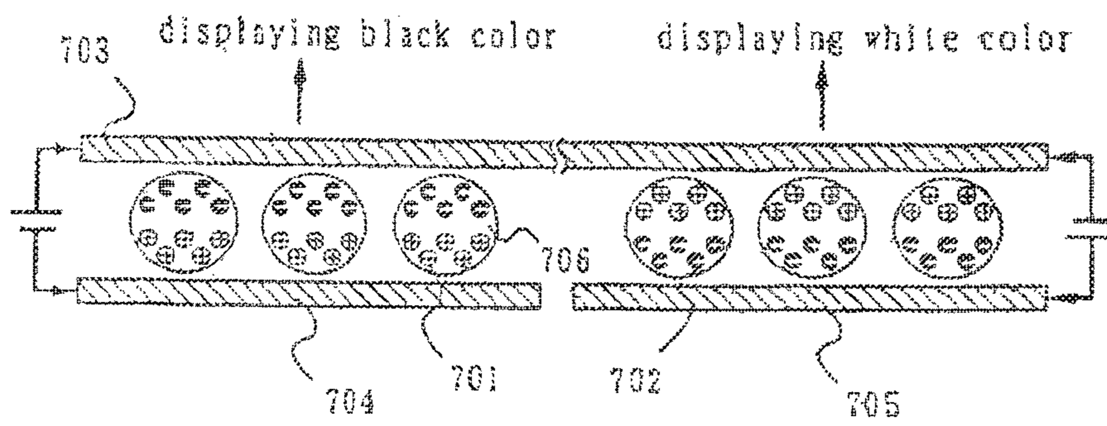
Fig. 10
