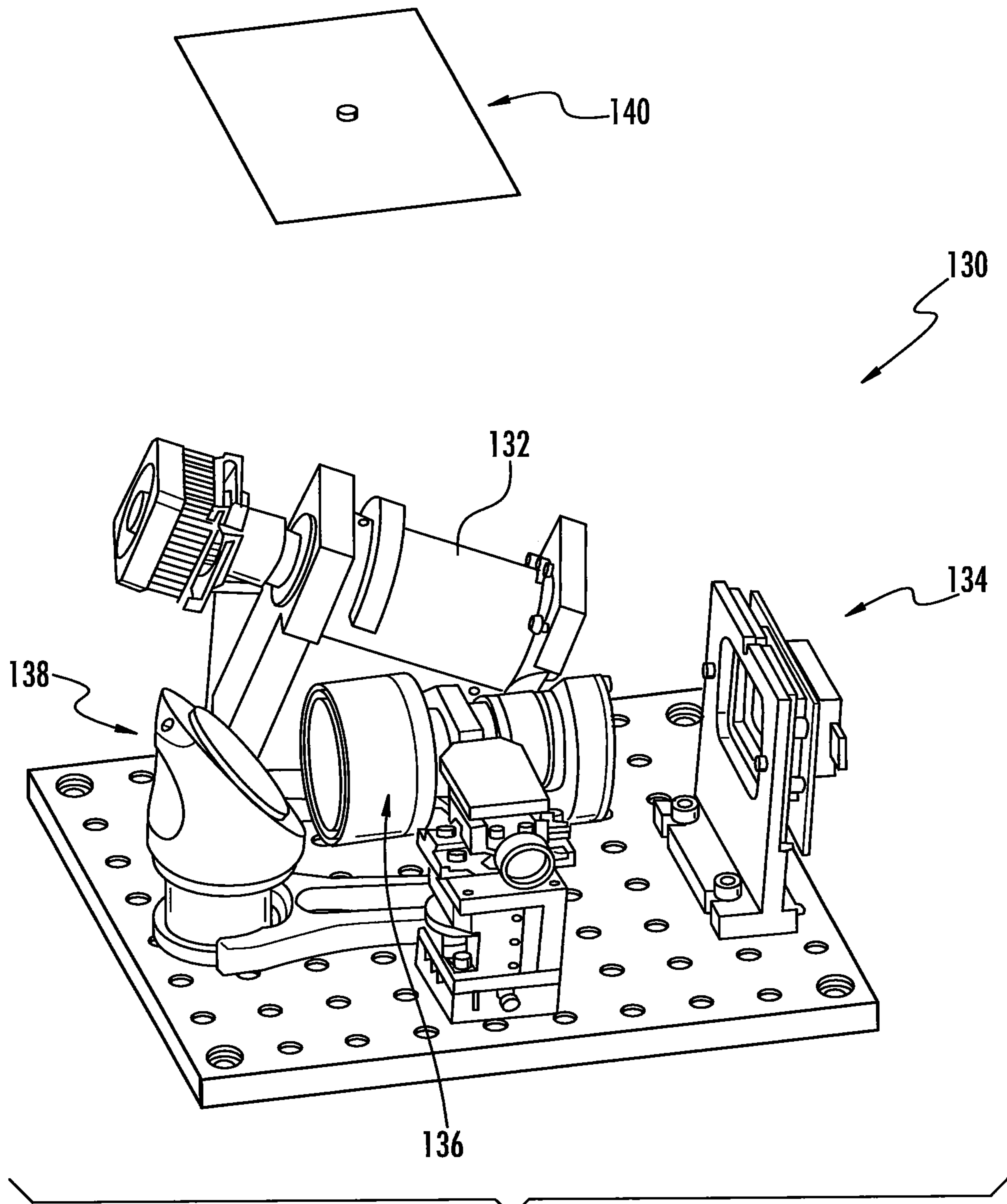
FIG. 15
