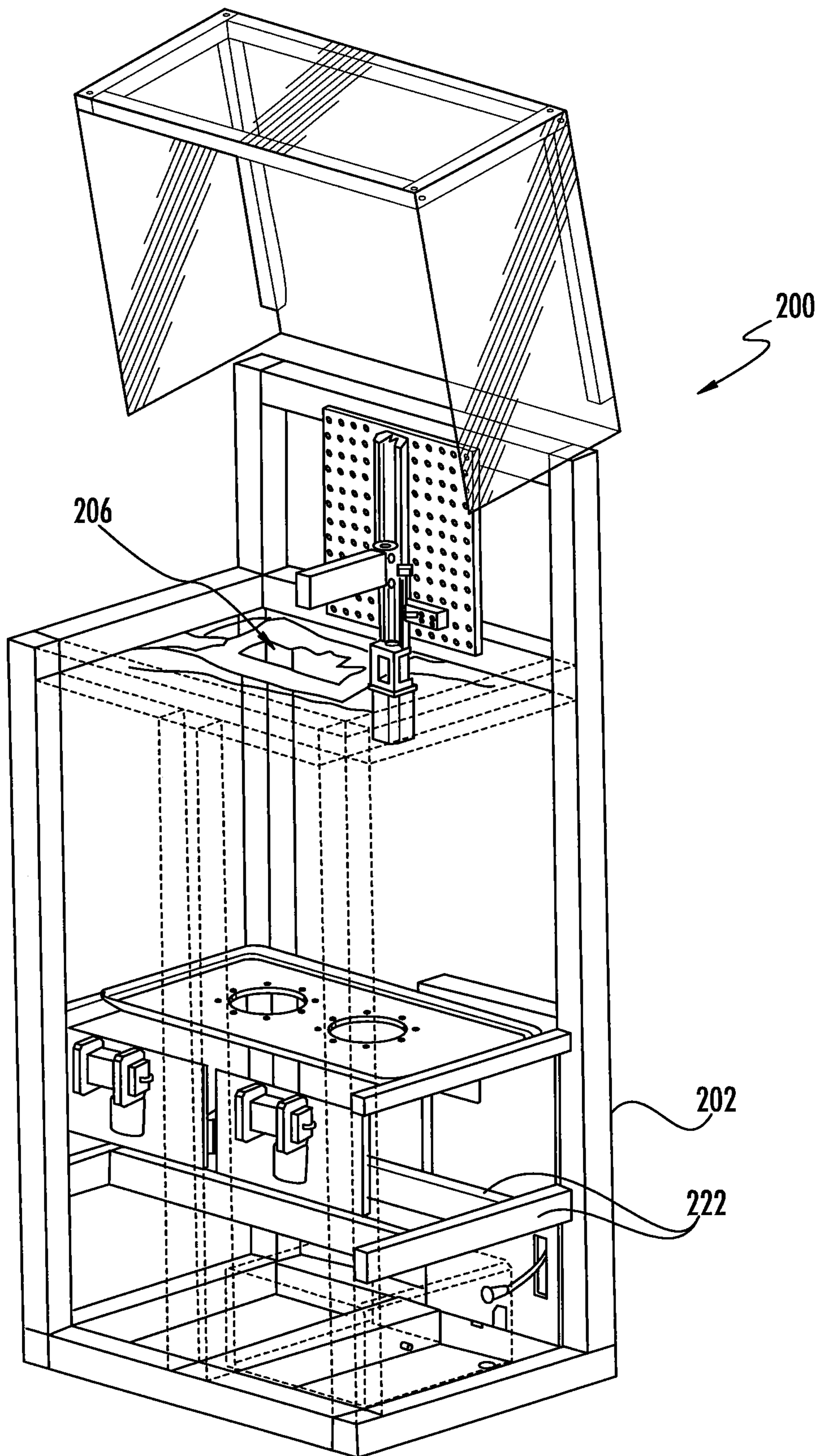
FIG. 16
