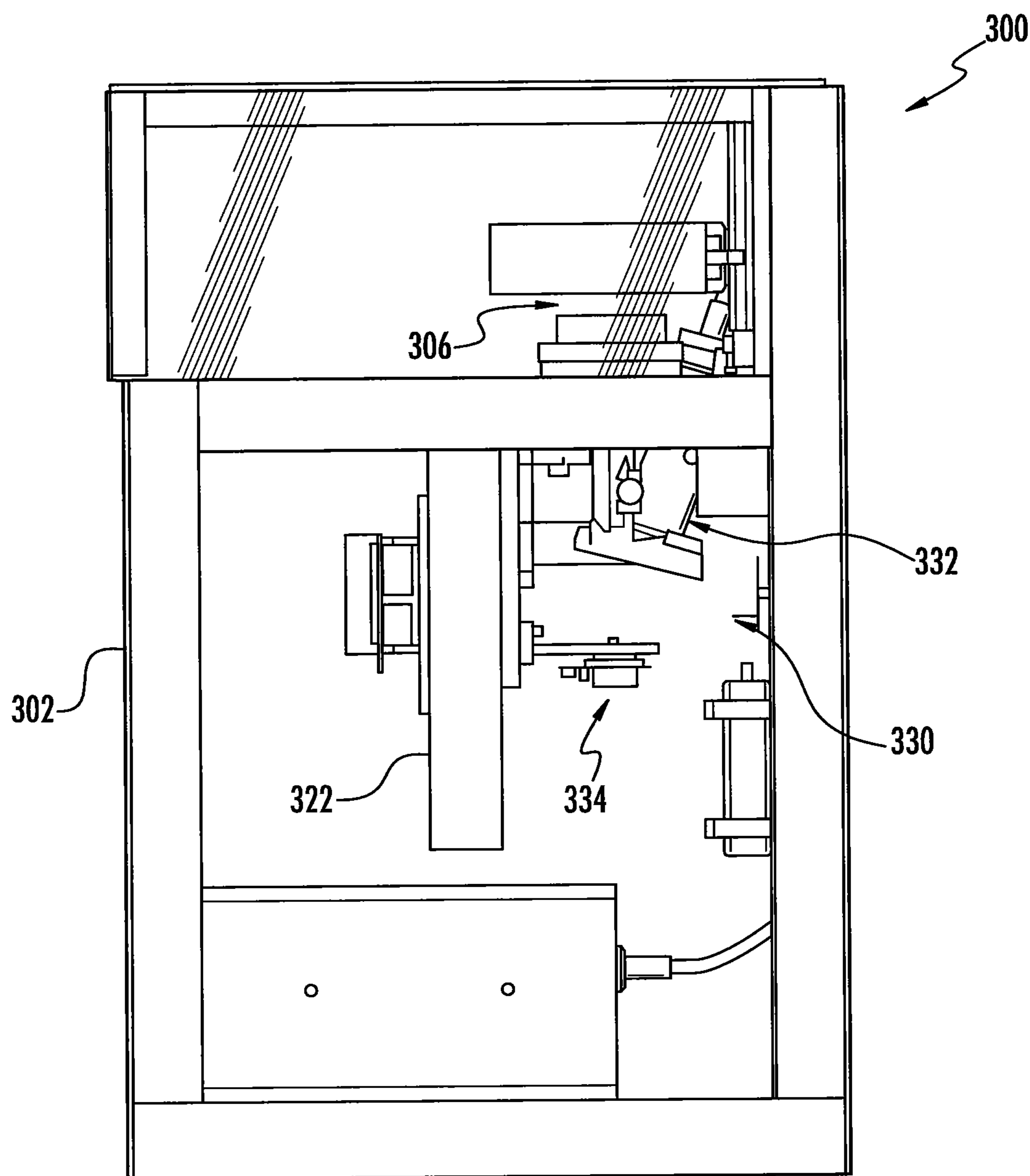
FIG. 19
