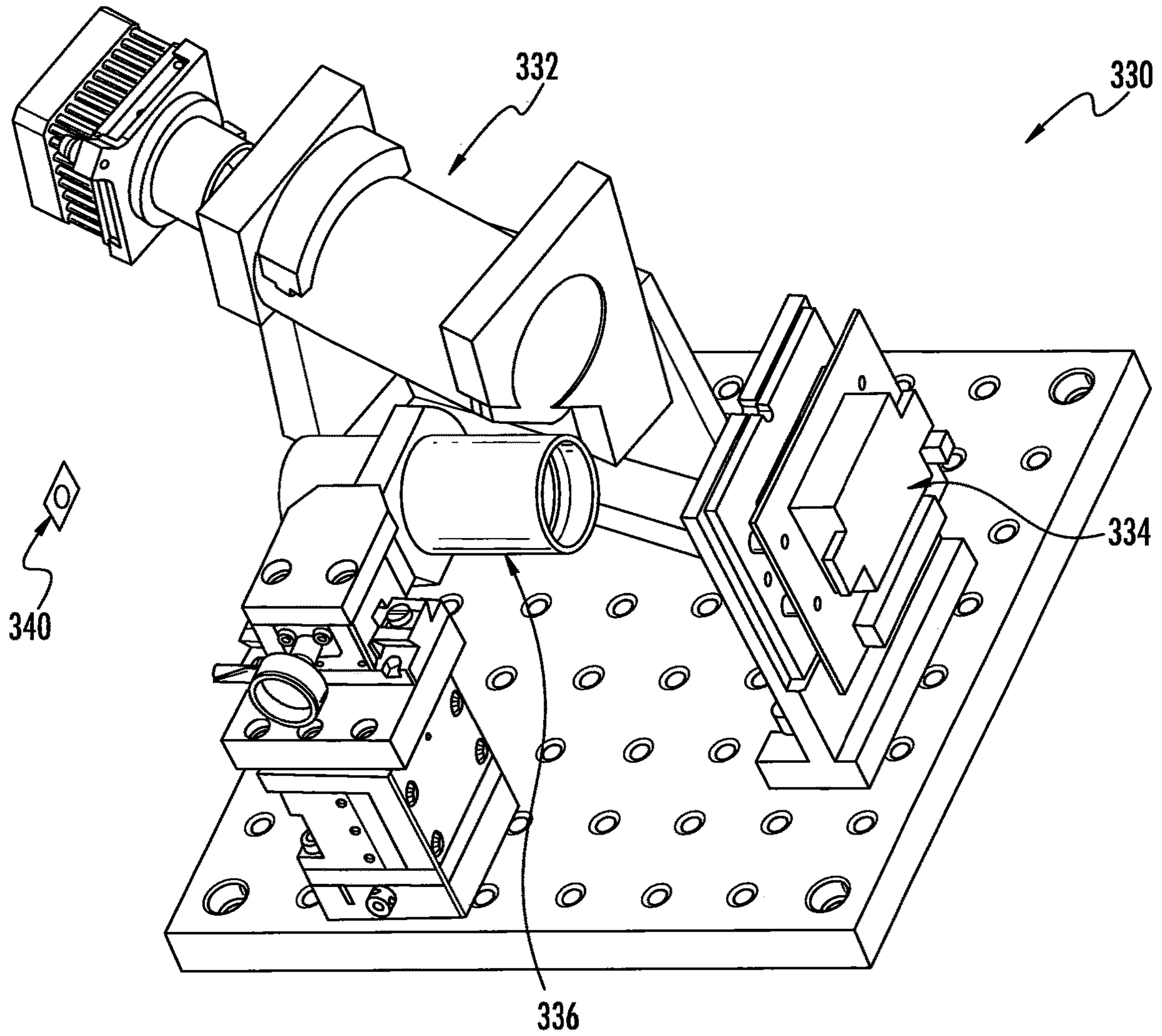
FIG. 20
