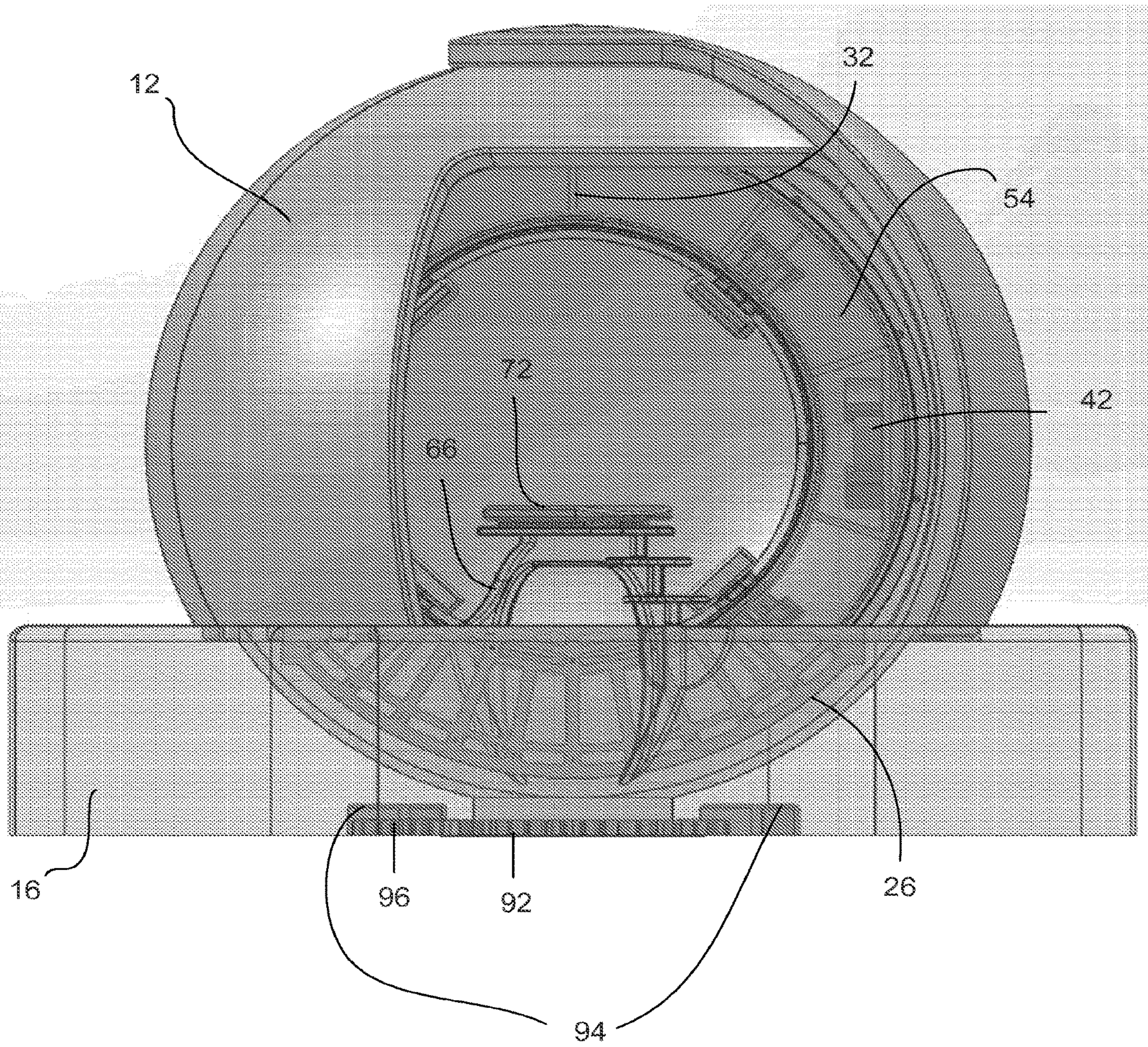
FIG. 14C
