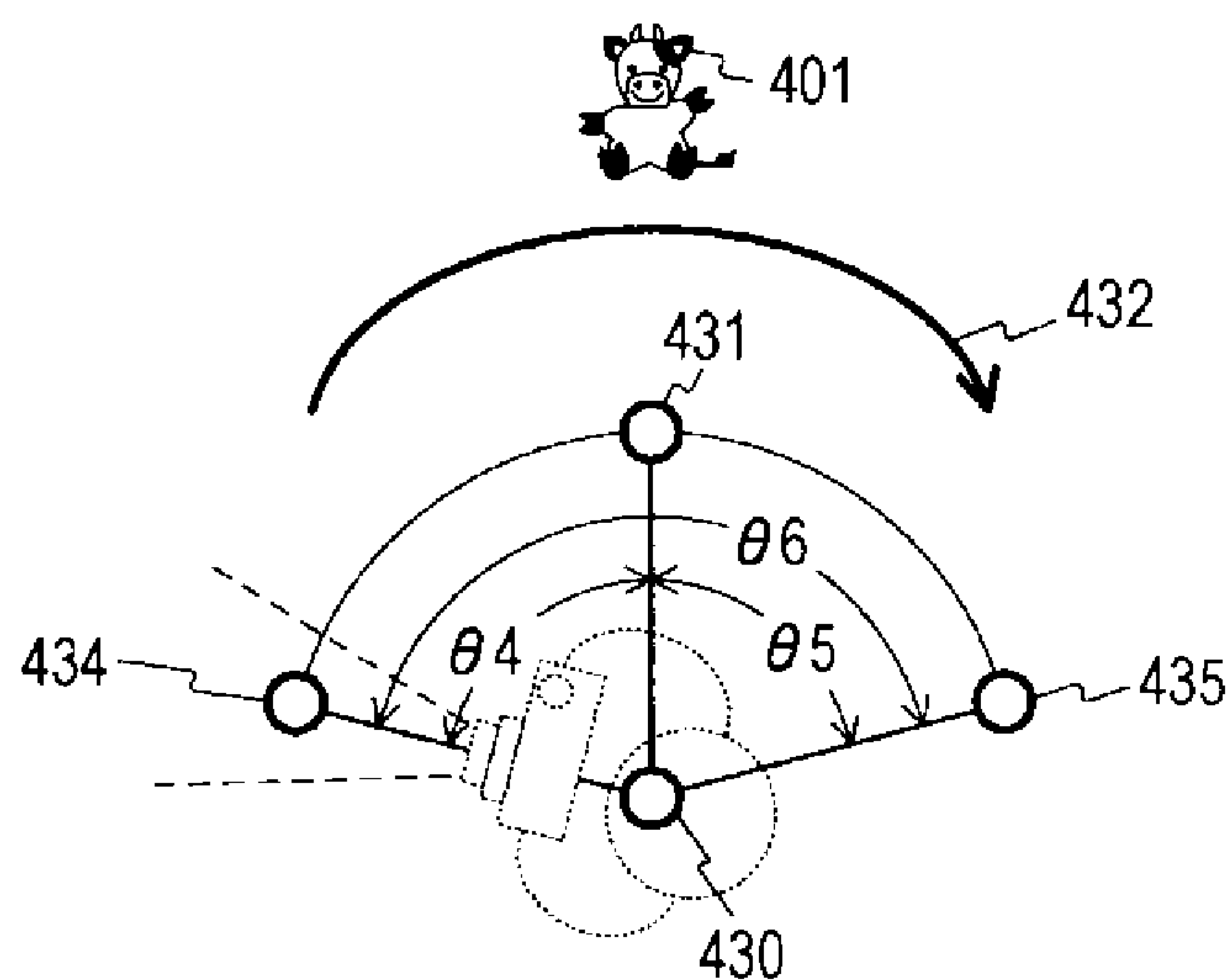
FIG. 18B
