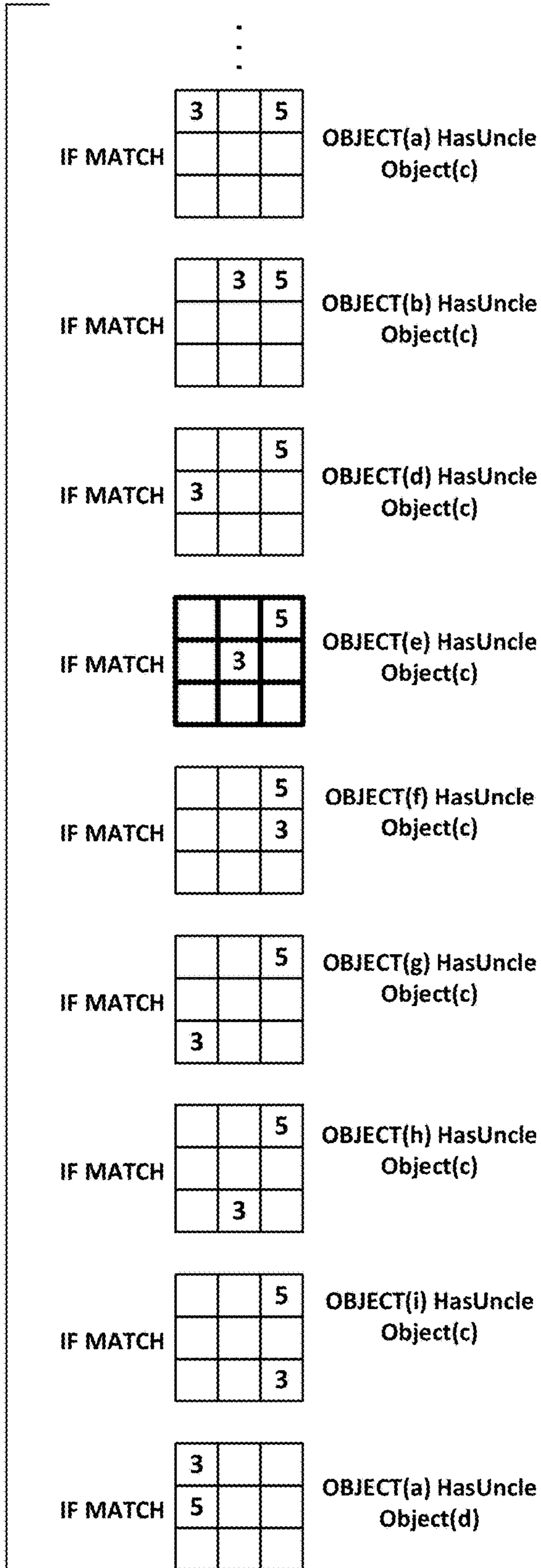
FIG. 26 – PREDICATE TEMPLATES
