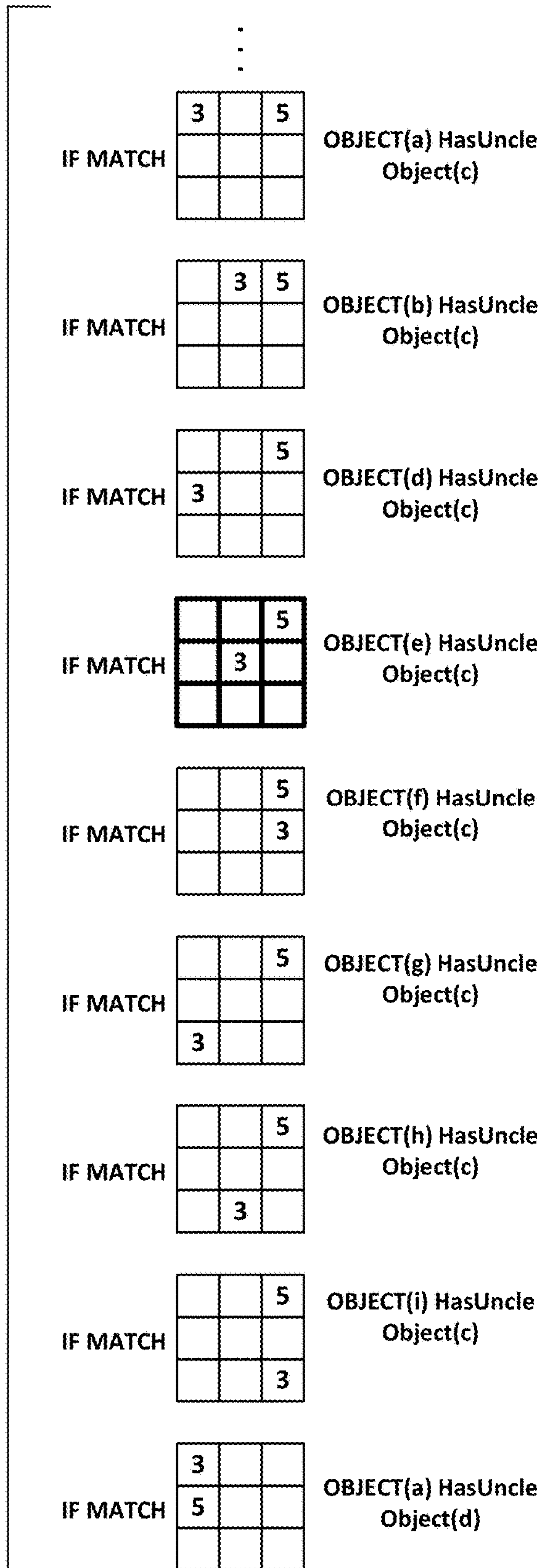
FIG. 26 – PREDICATE TEMPLATES
