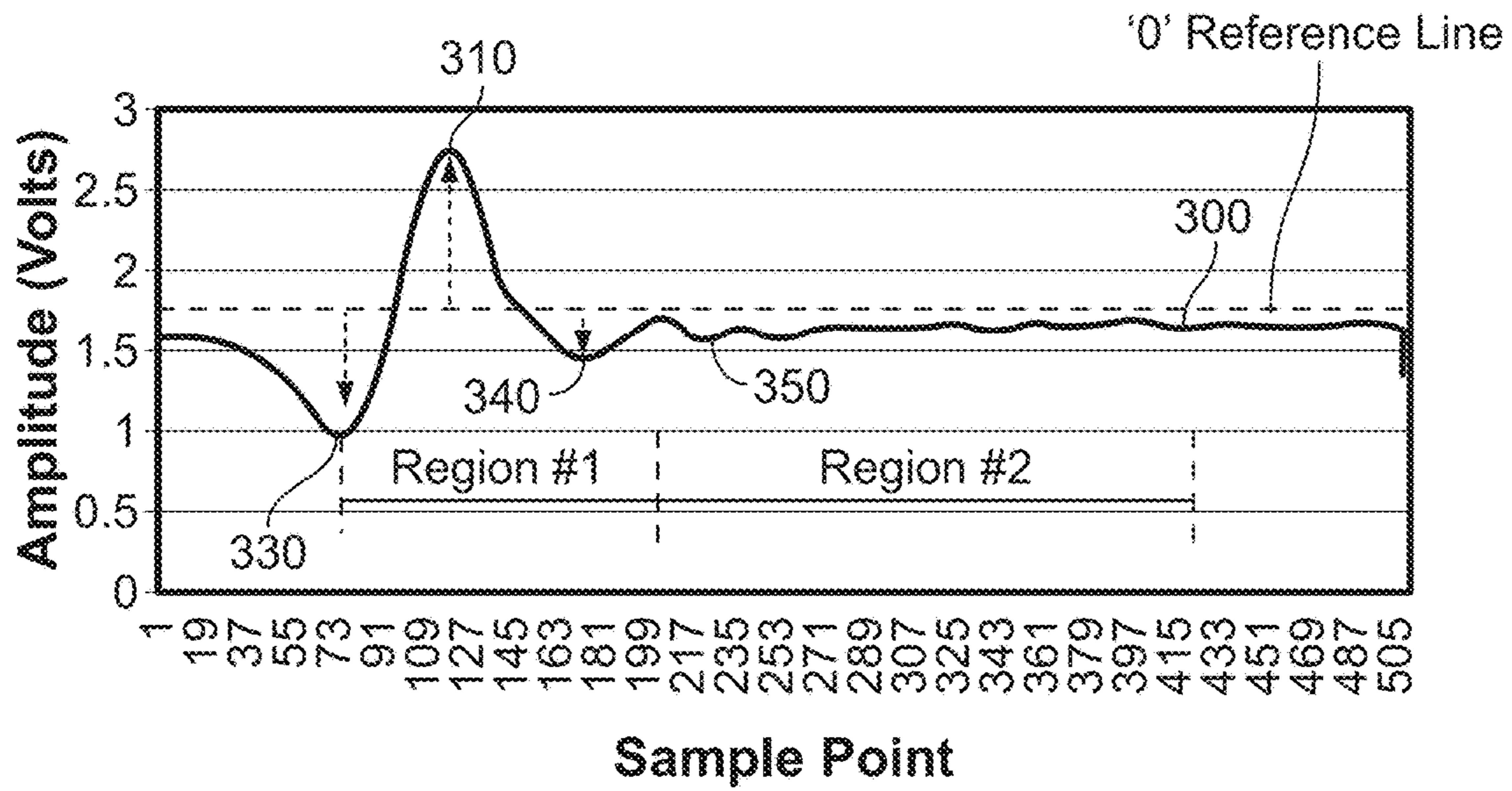
FIG. 15
