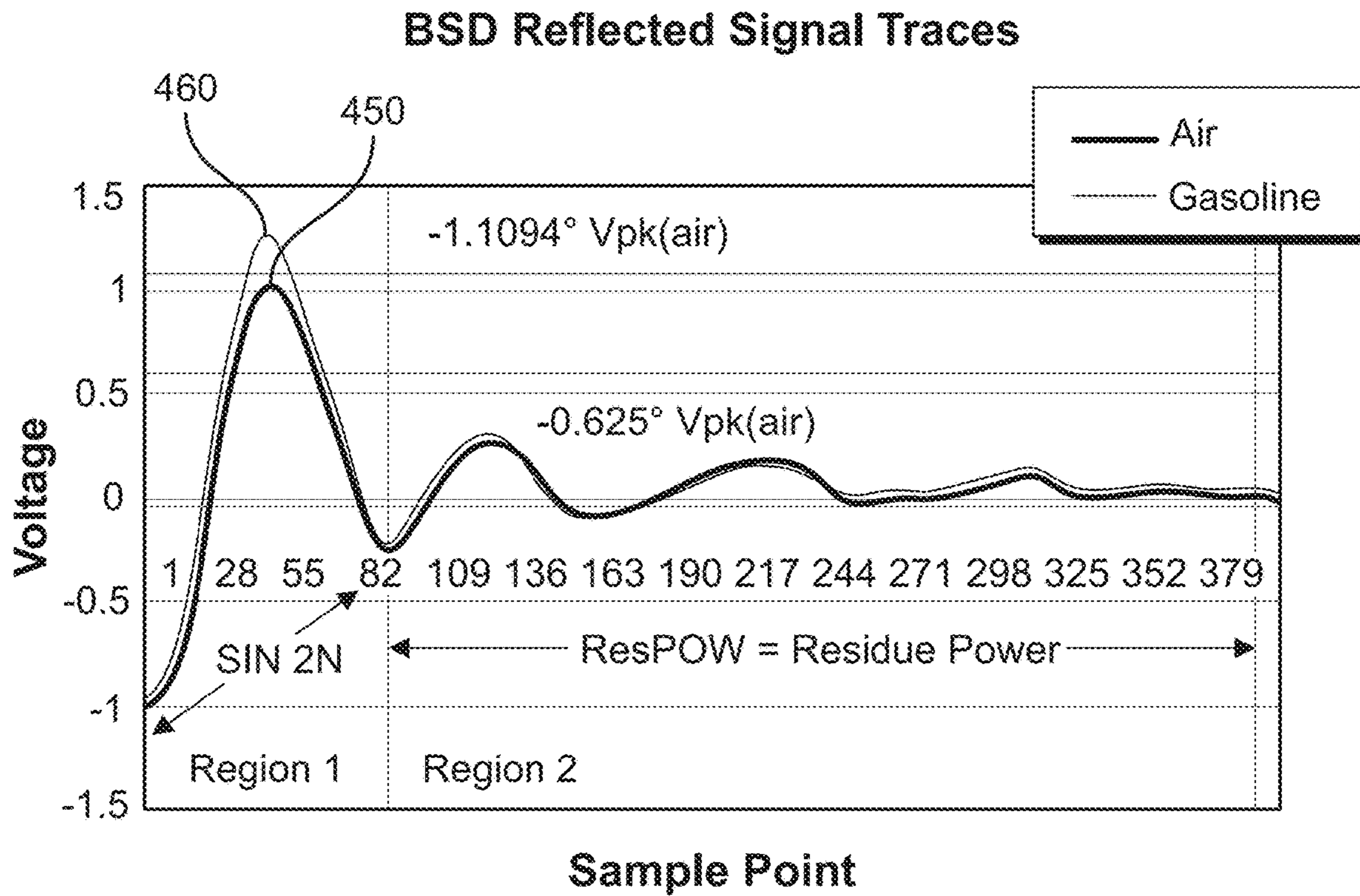
FIG. 16
