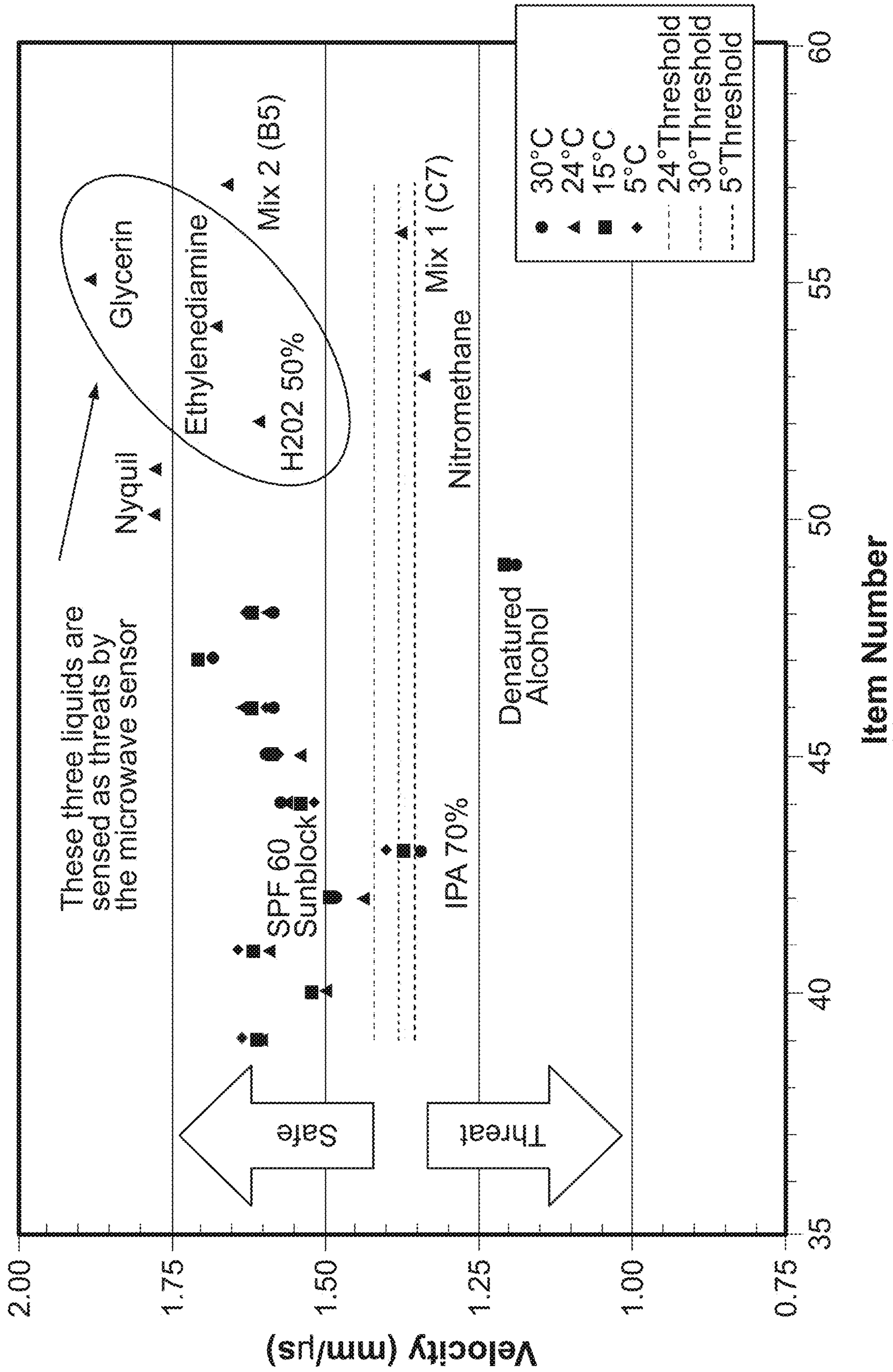
FIG. 21
