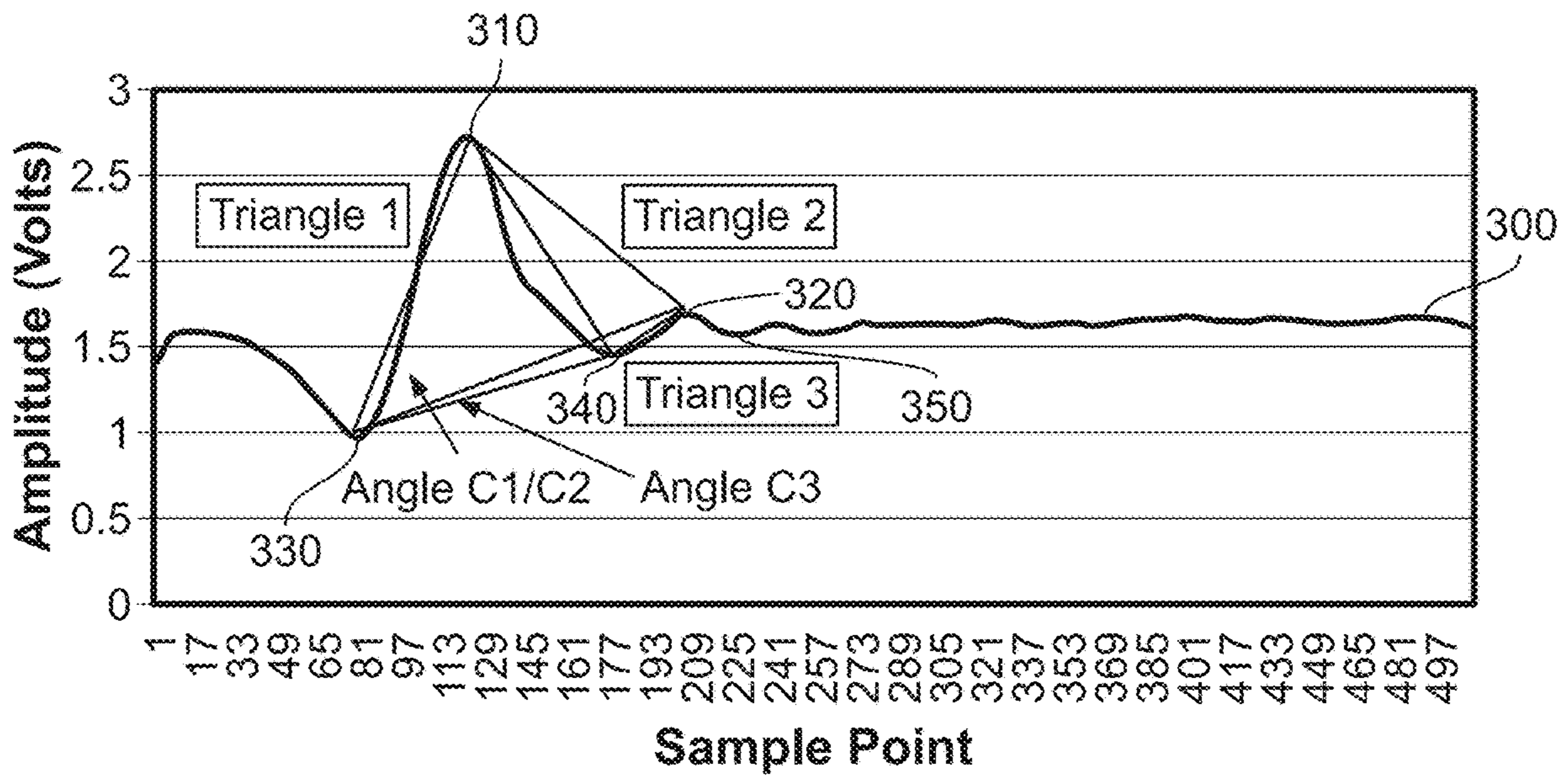
FIG. 14
