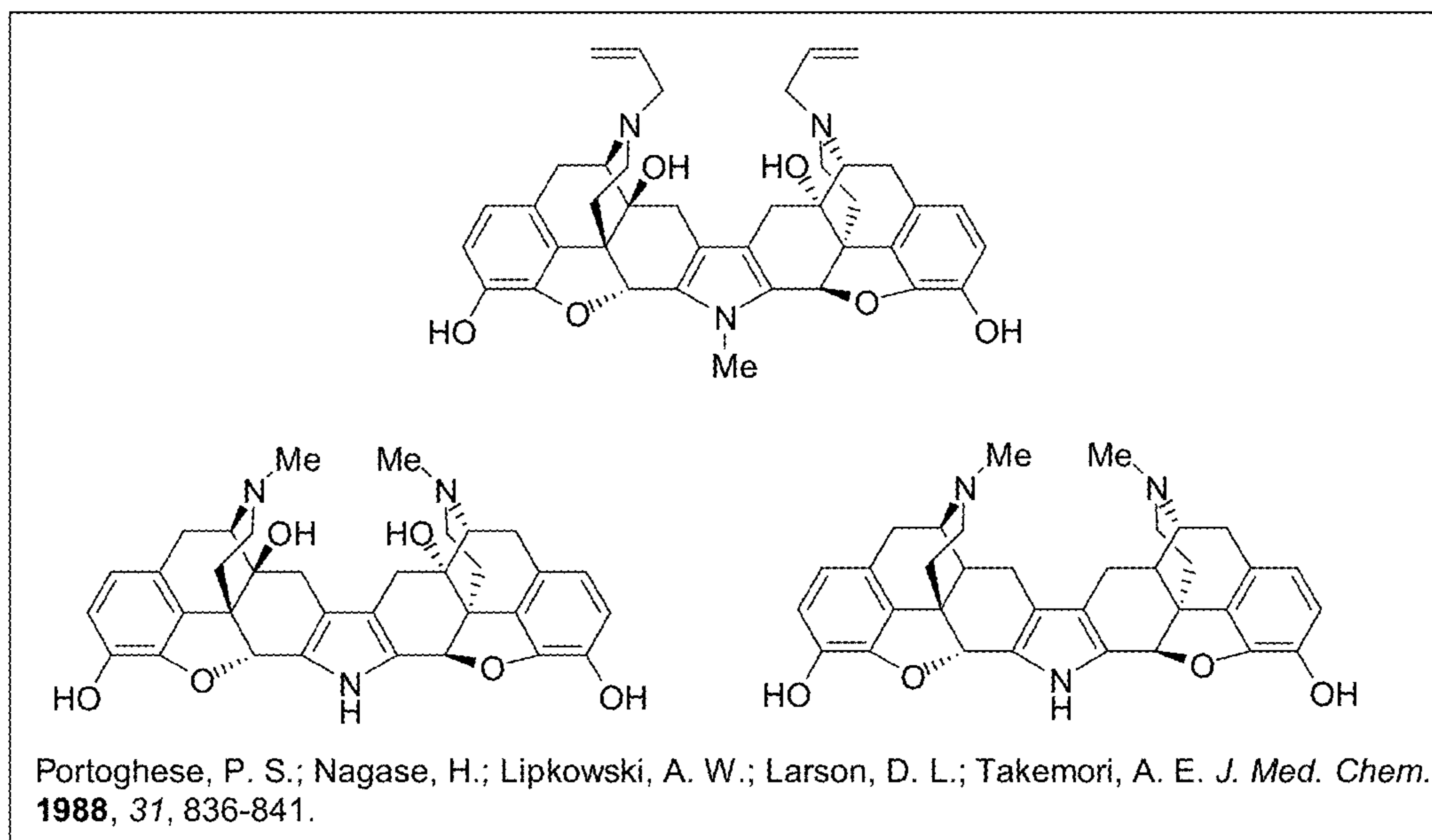
norBNI enantiomer
