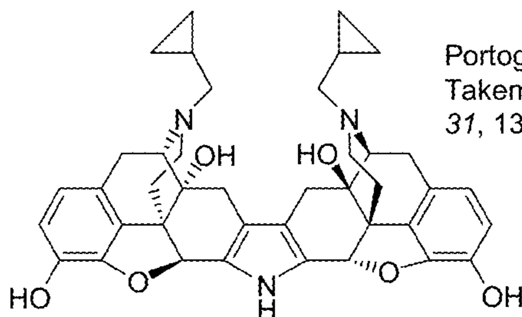
norBNI enantiomer
