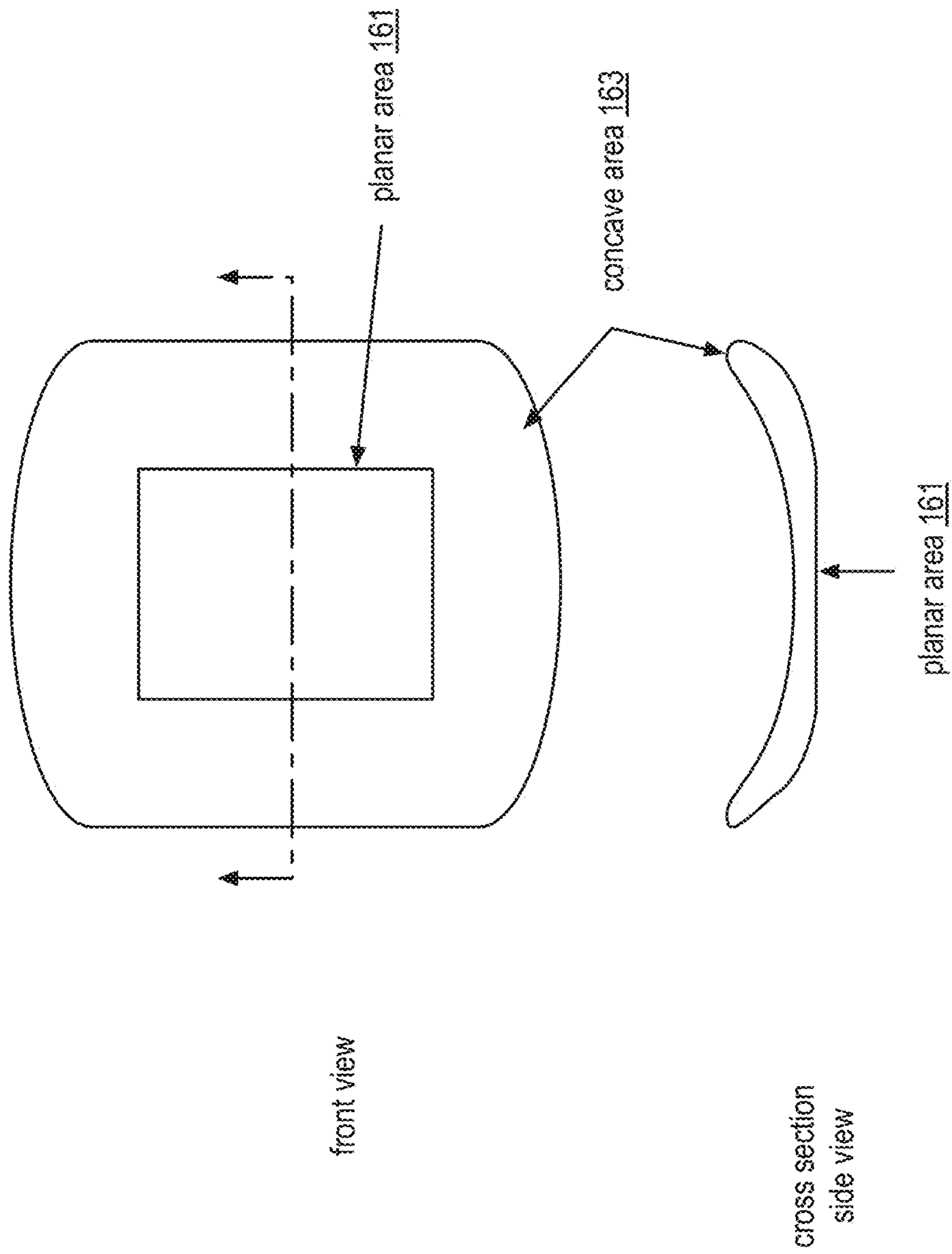
FIG. 27 outer layer 153
