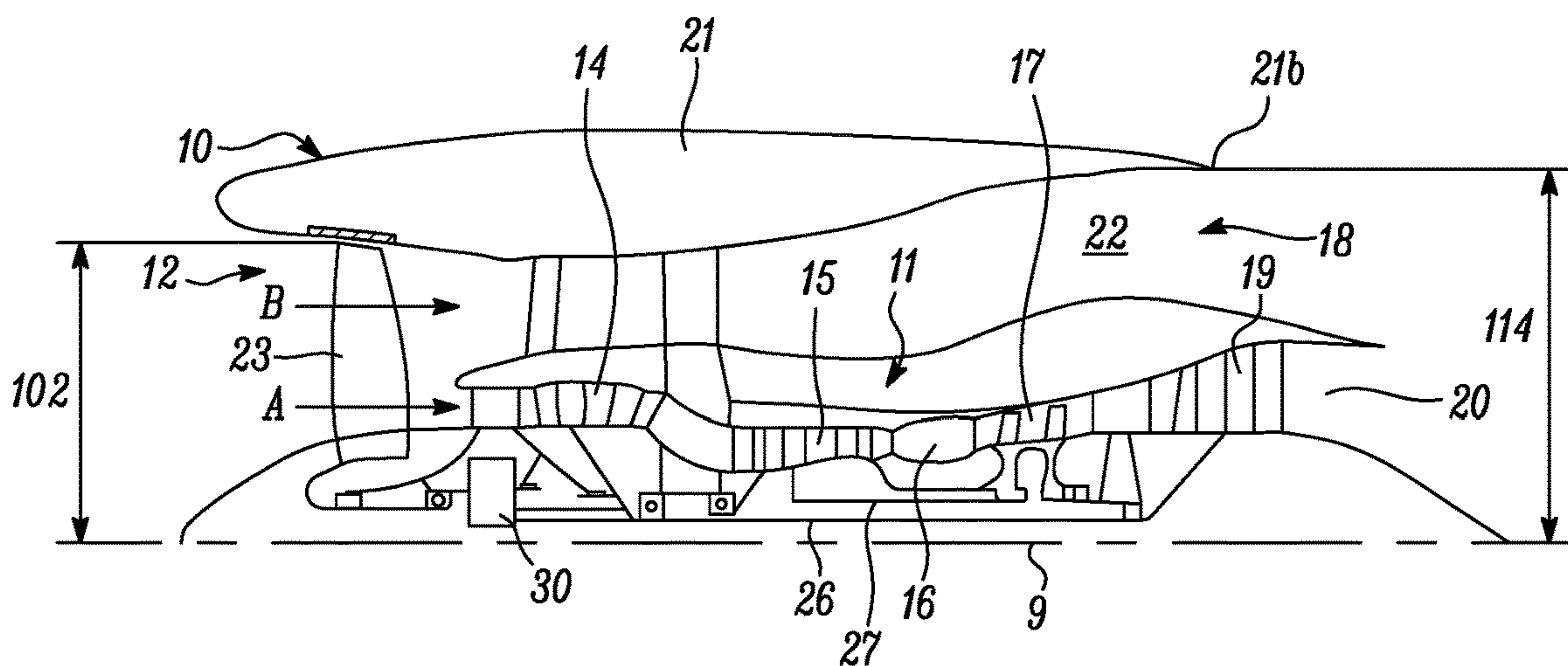
FIG. 7A
