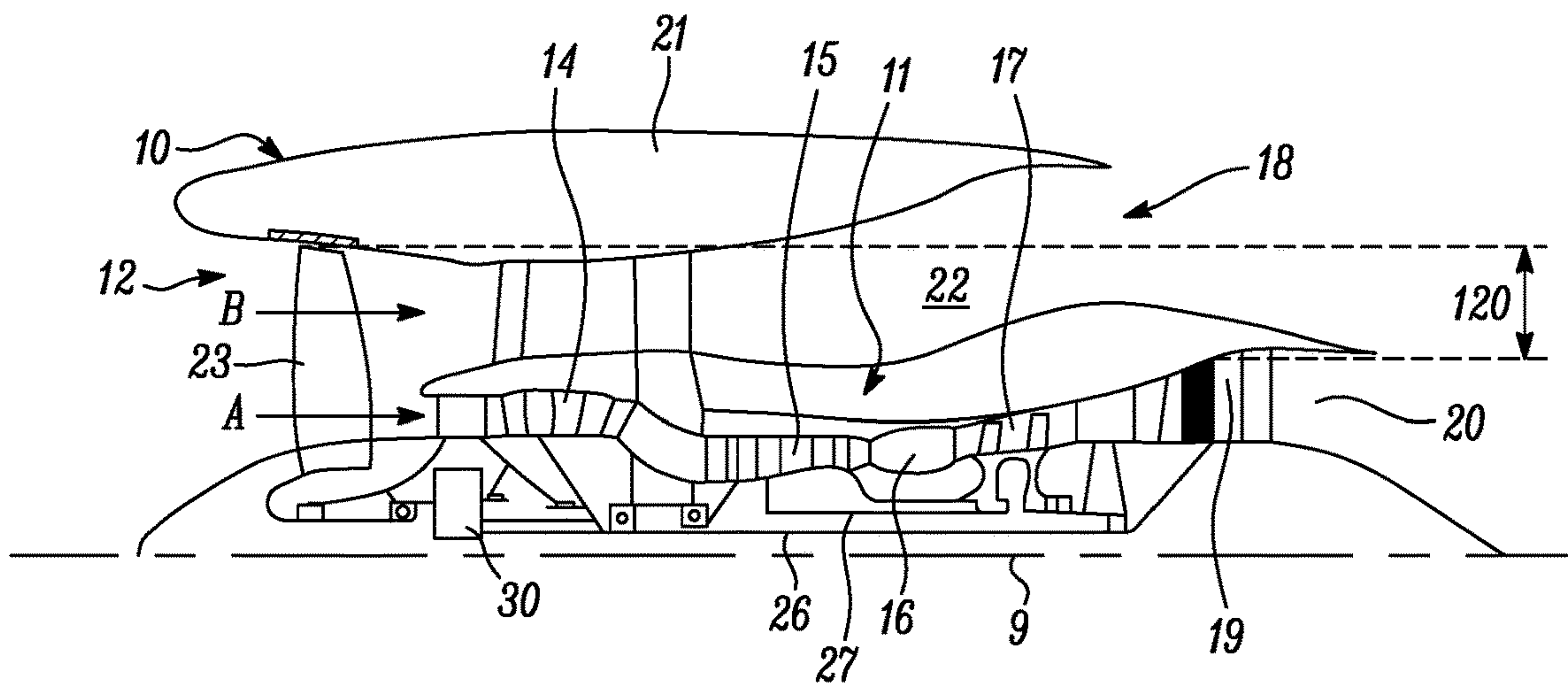
FIG. 10A
