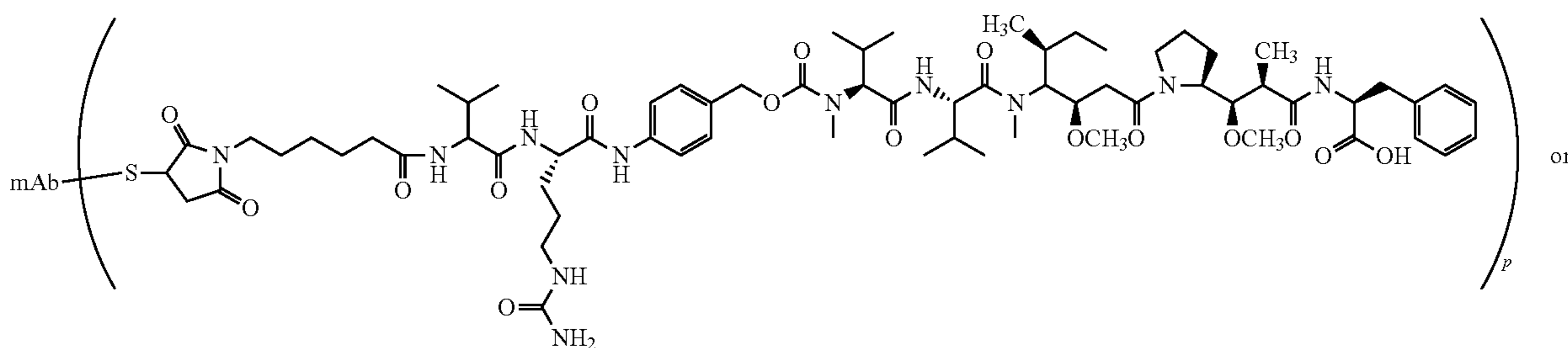
L-MC-vc-PAB-MMAP
