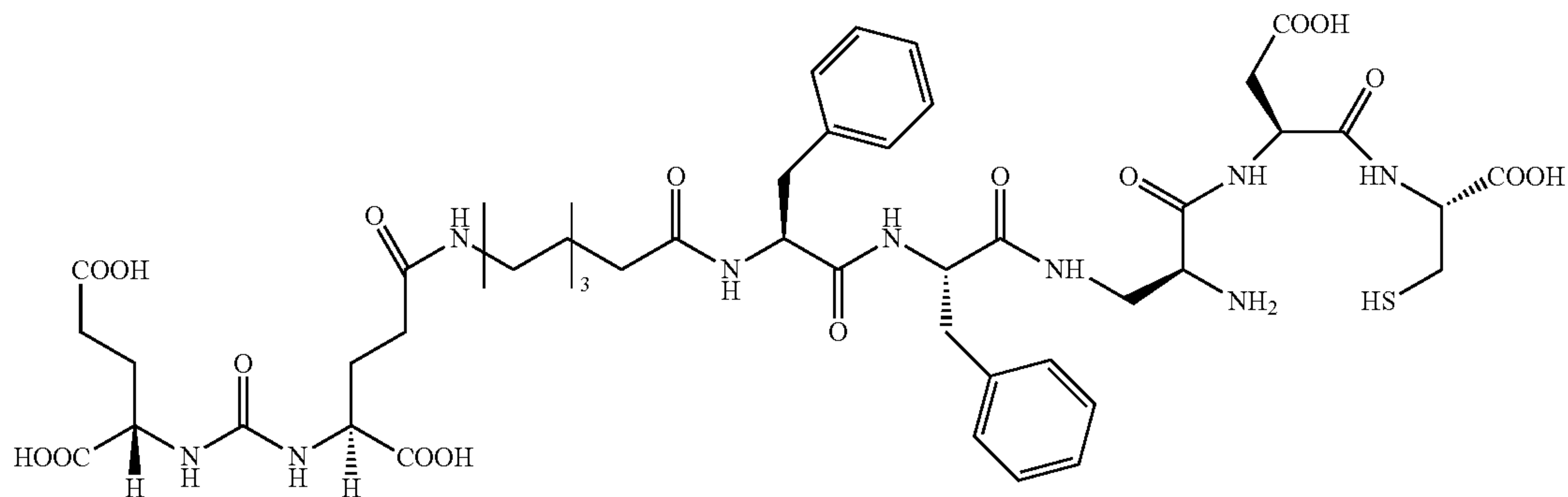
PC01SK28 \text{C}_{47}\text{H}_{65}\text{N}_9\text{O}_{17}\text{S} Mol. Wt.: 1060.13
