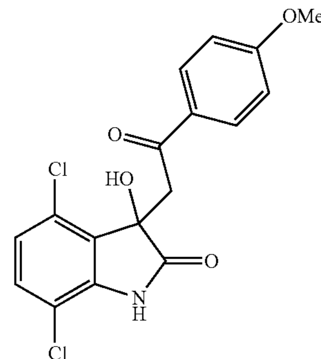
4,7-dichloro-3-hydroxy-3-(2-(4-methoxyphenyl)-2-oxoethyl)indolin-2-one
