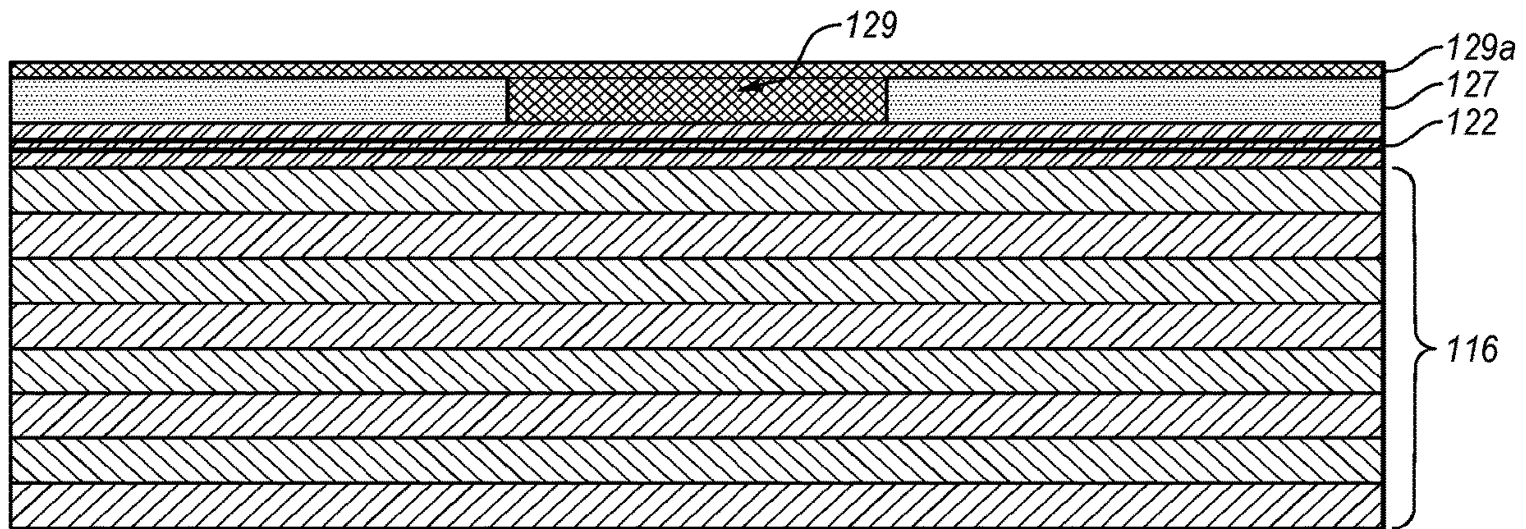
FIG. 5A
