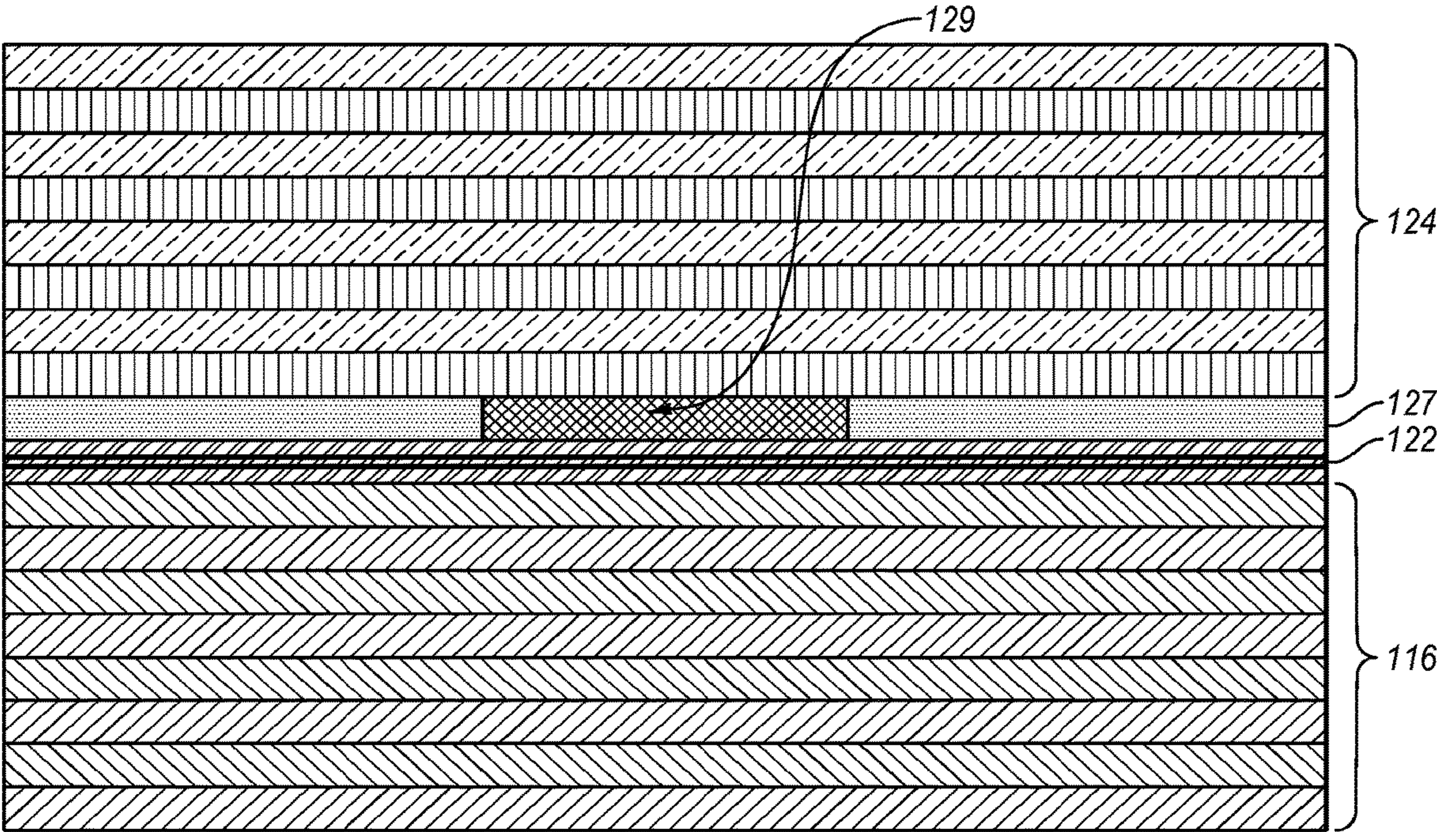
FIG. 6A
