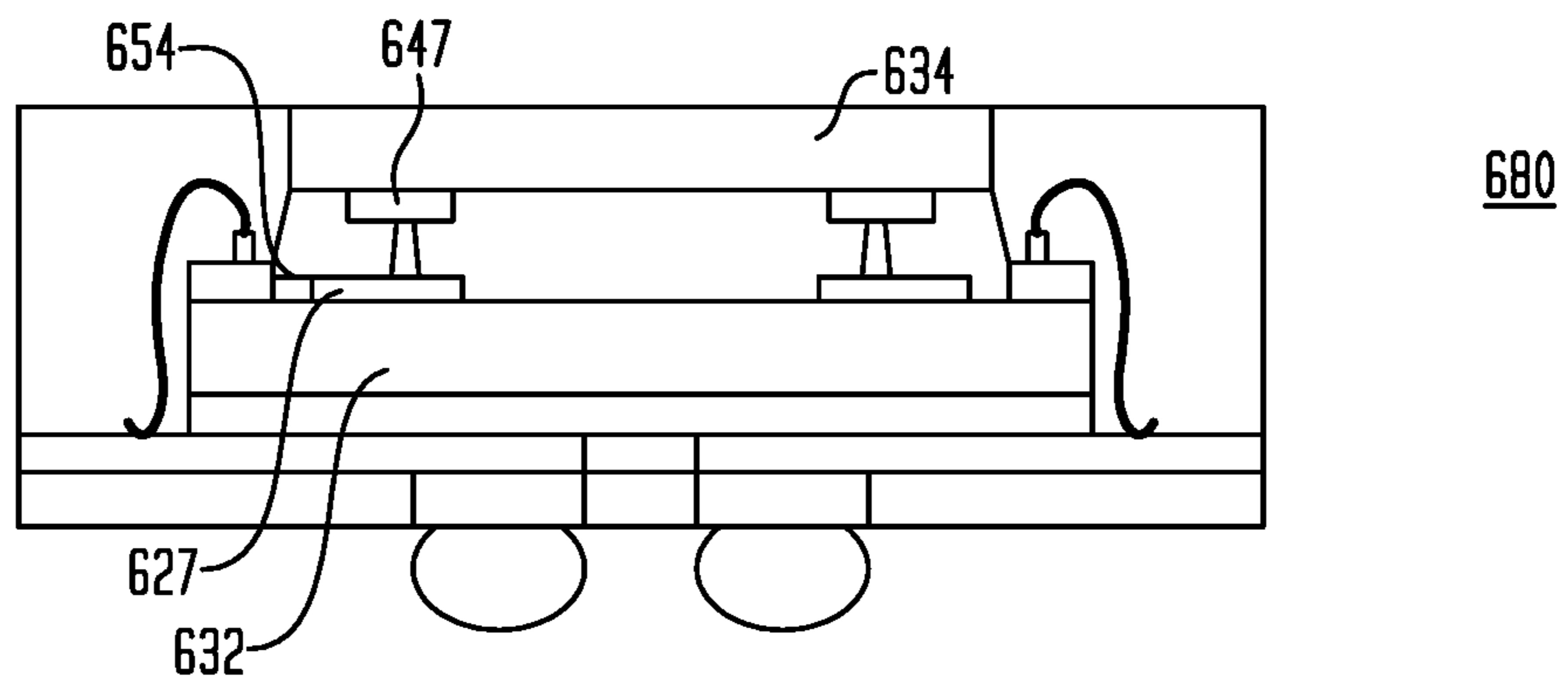
FIG. 15A
