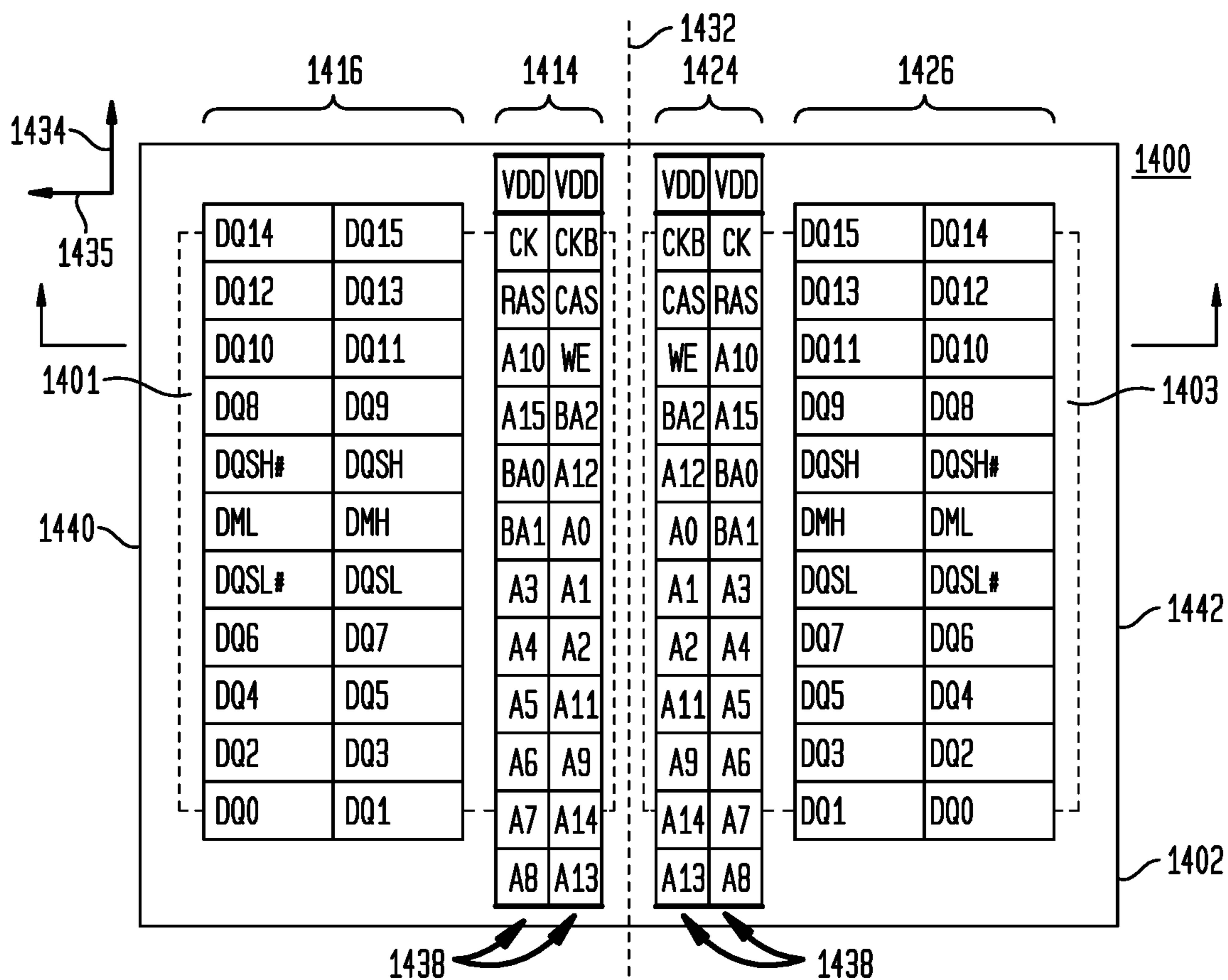
FIG. 16
