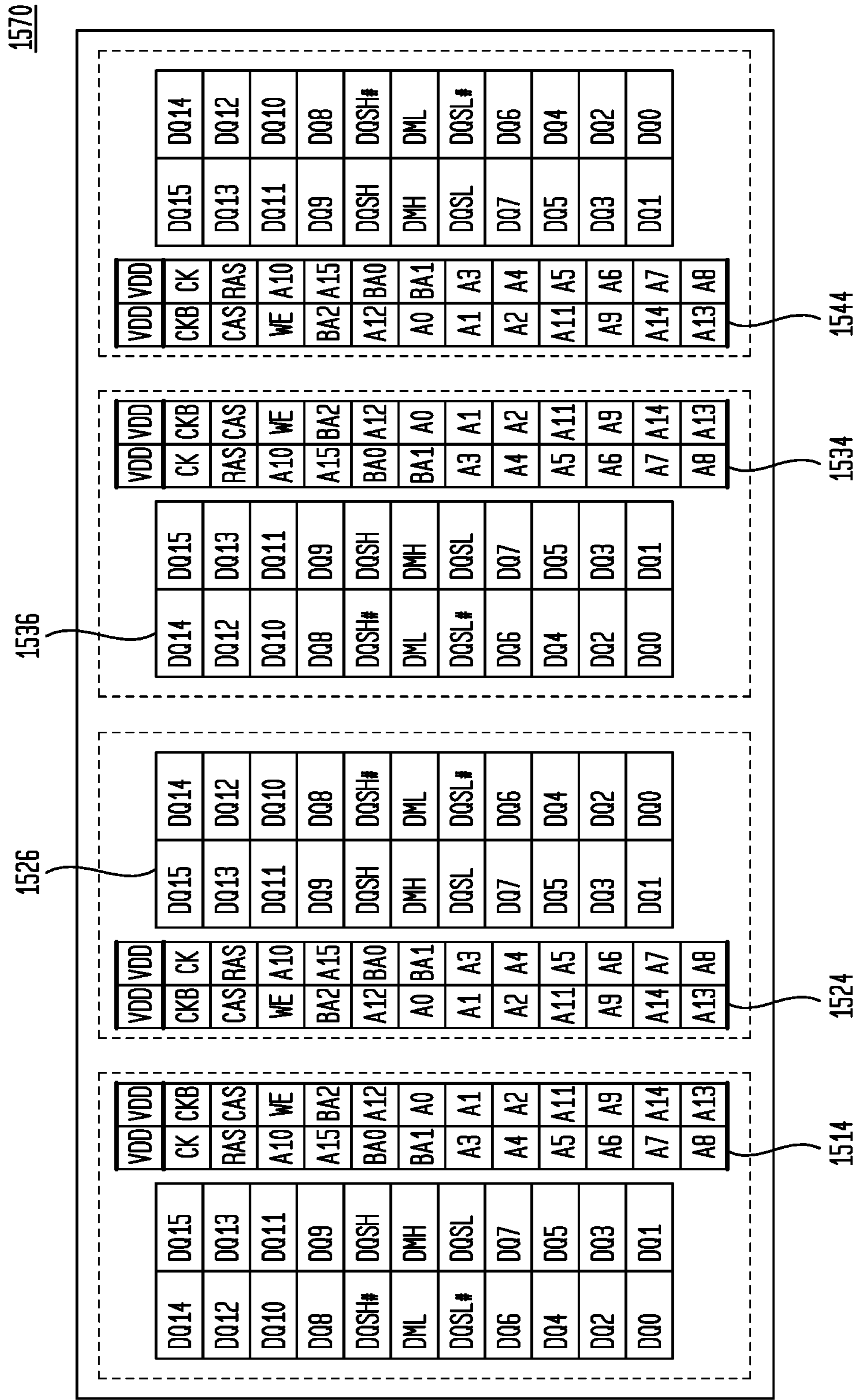
FIG. 25
