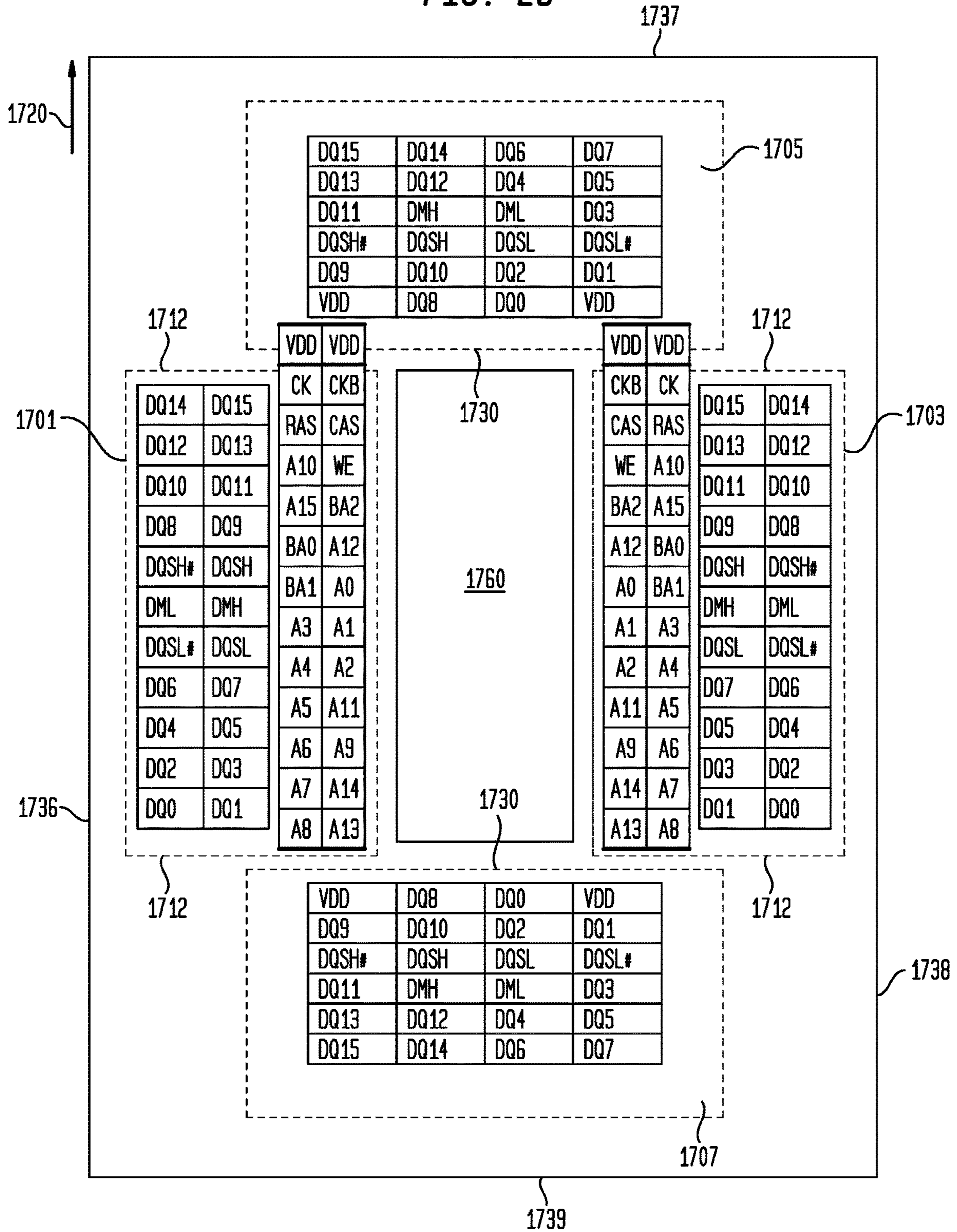
FIG. 28
