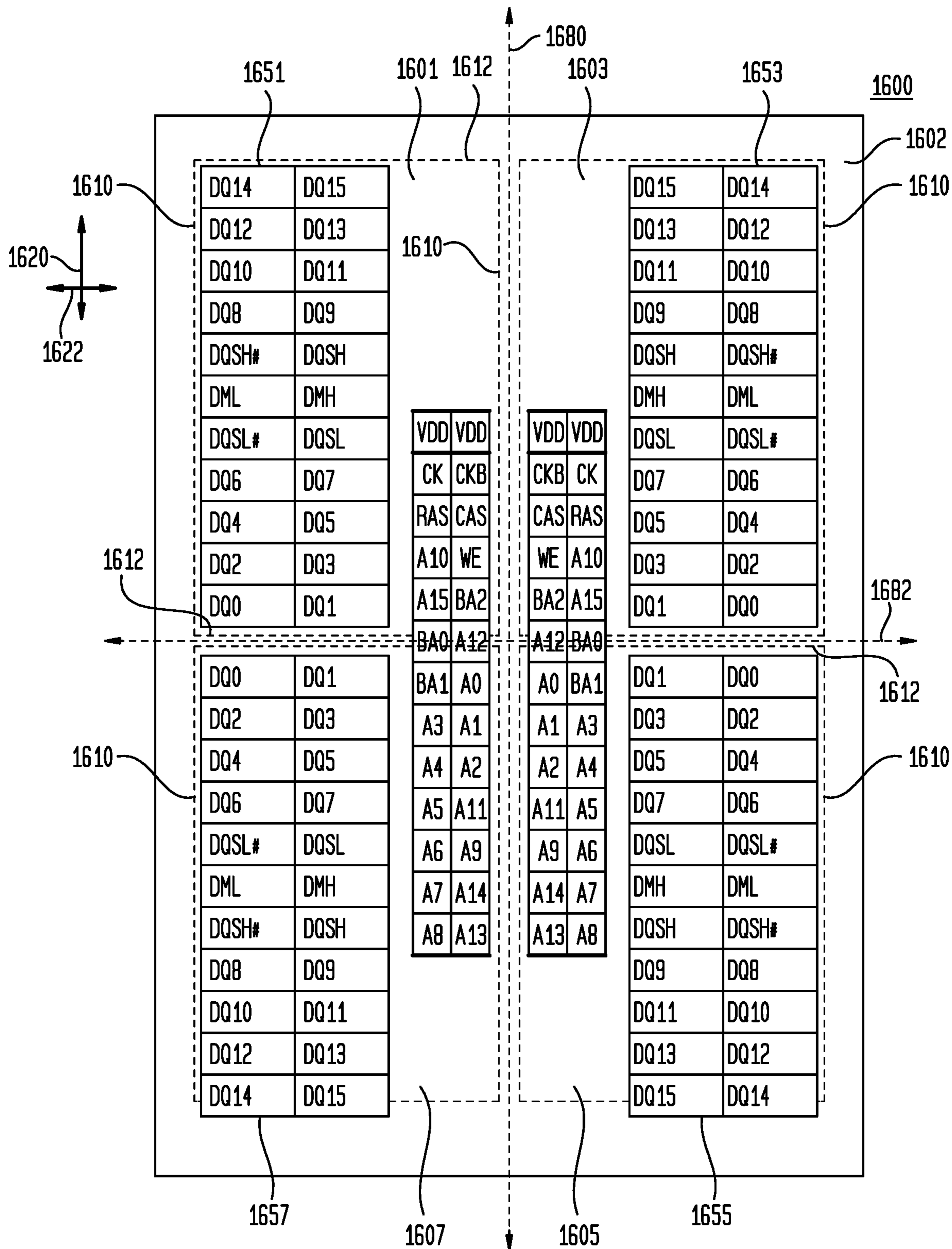
FIG. 26
