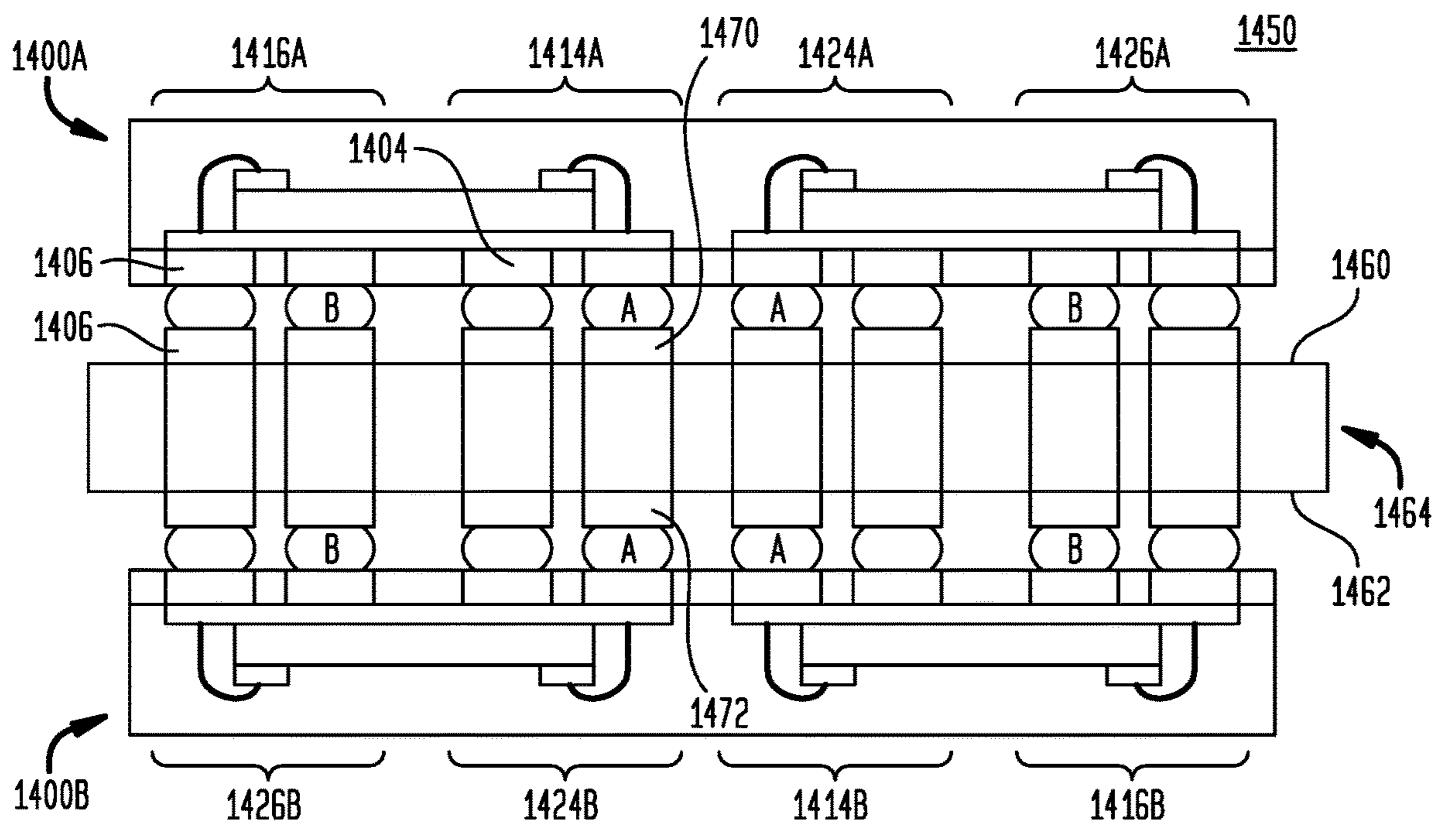
FIG. 19
