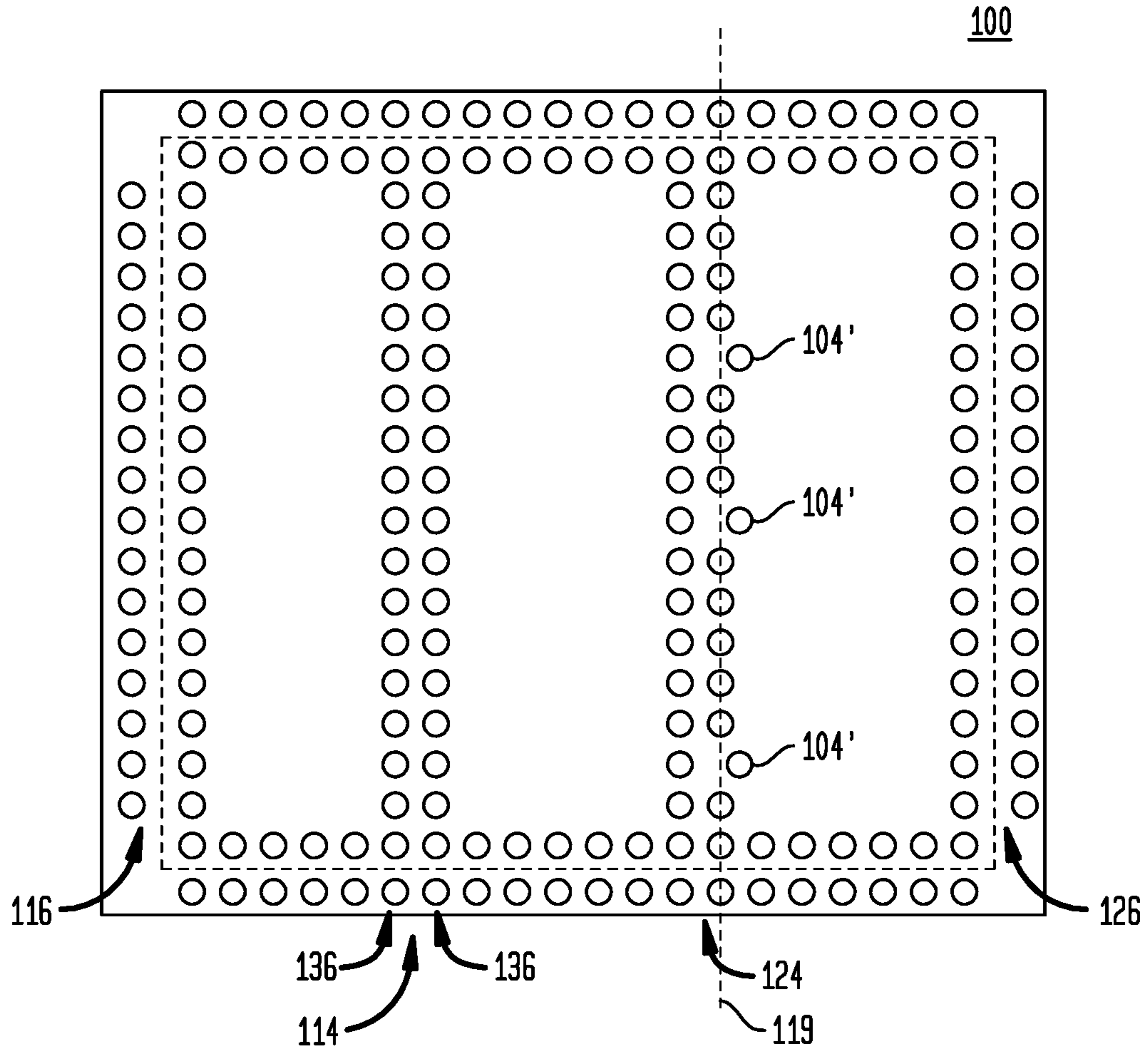
FIG. 5B
