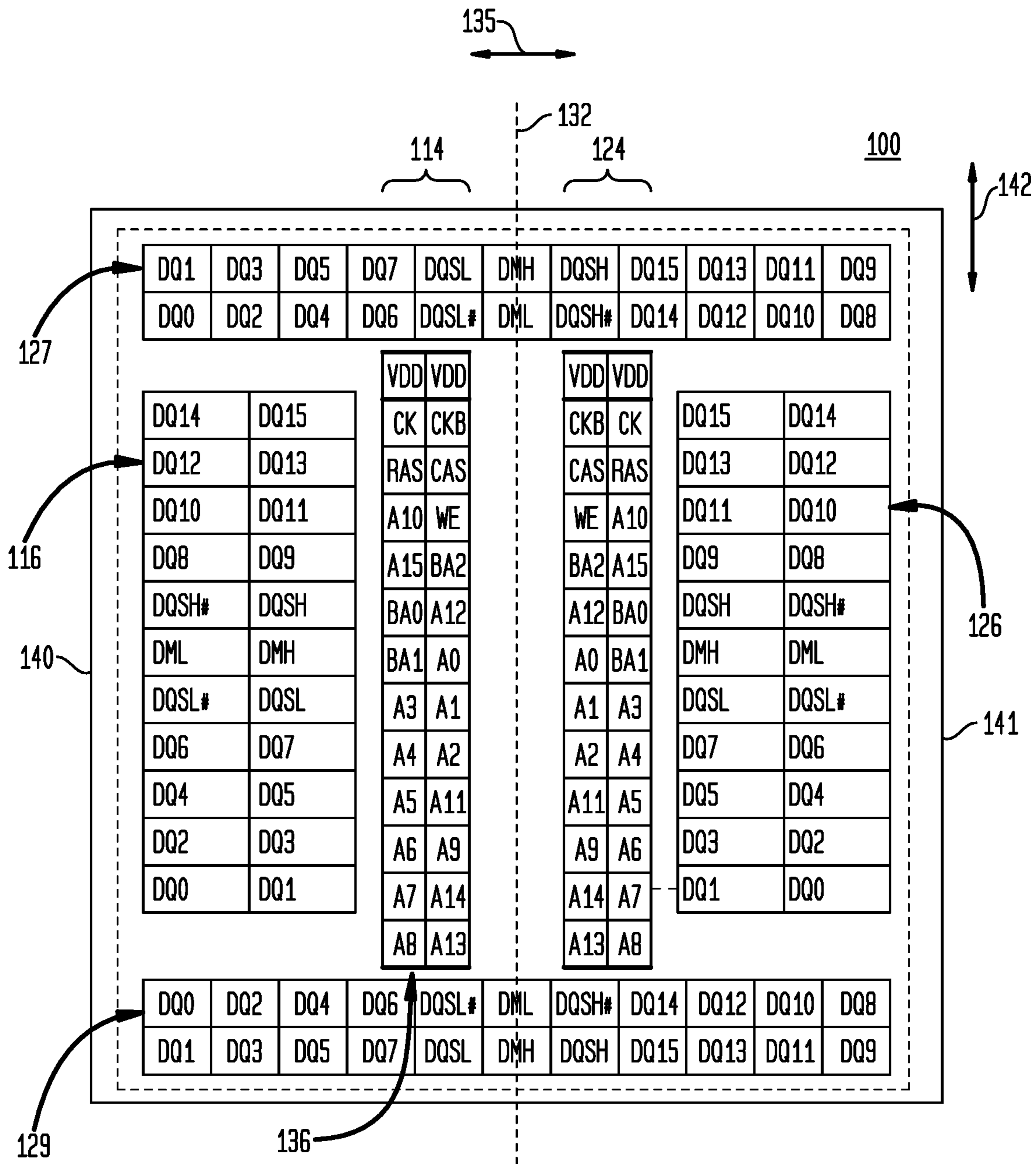
FIG. 5A
