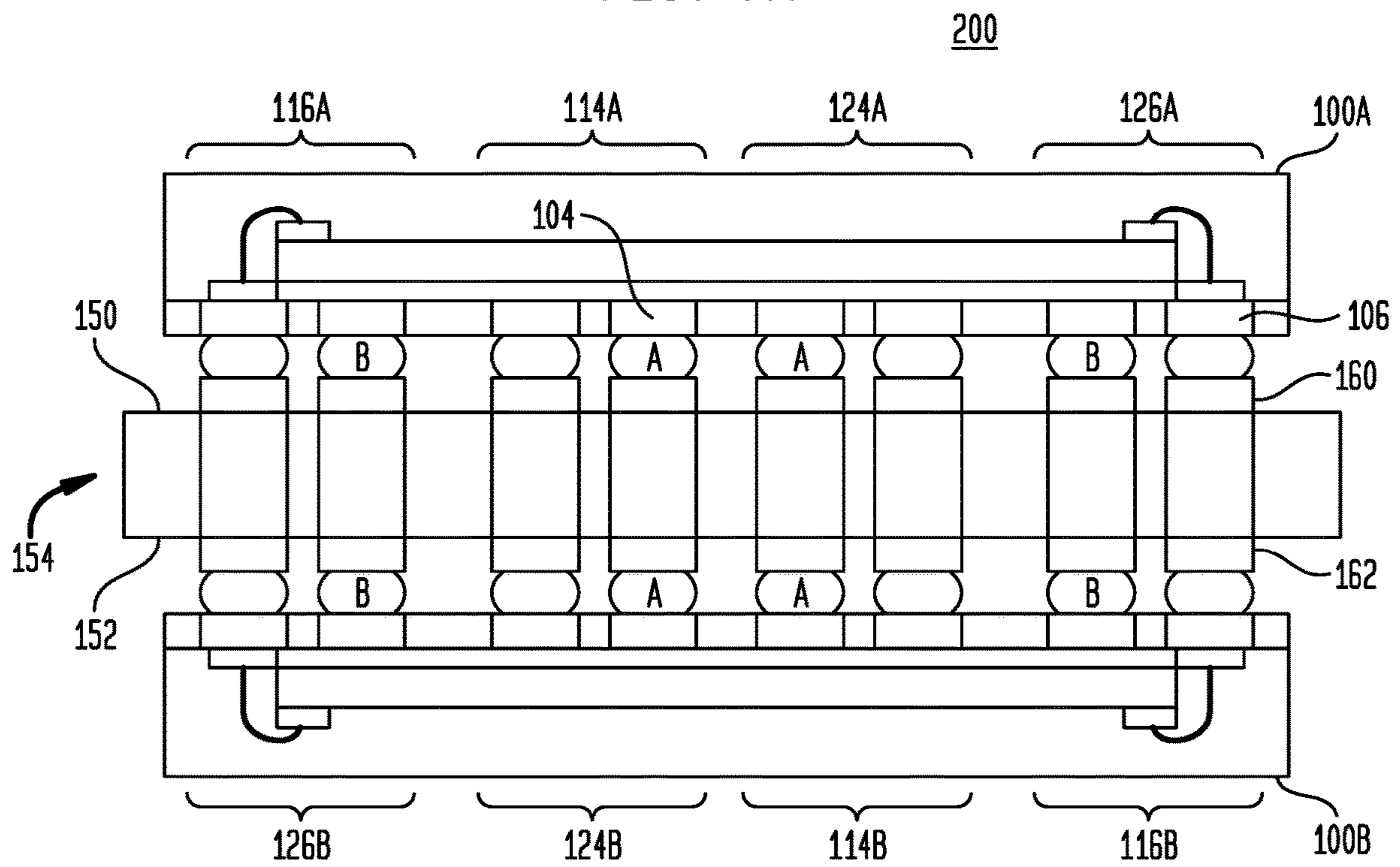
FIG. 7A
