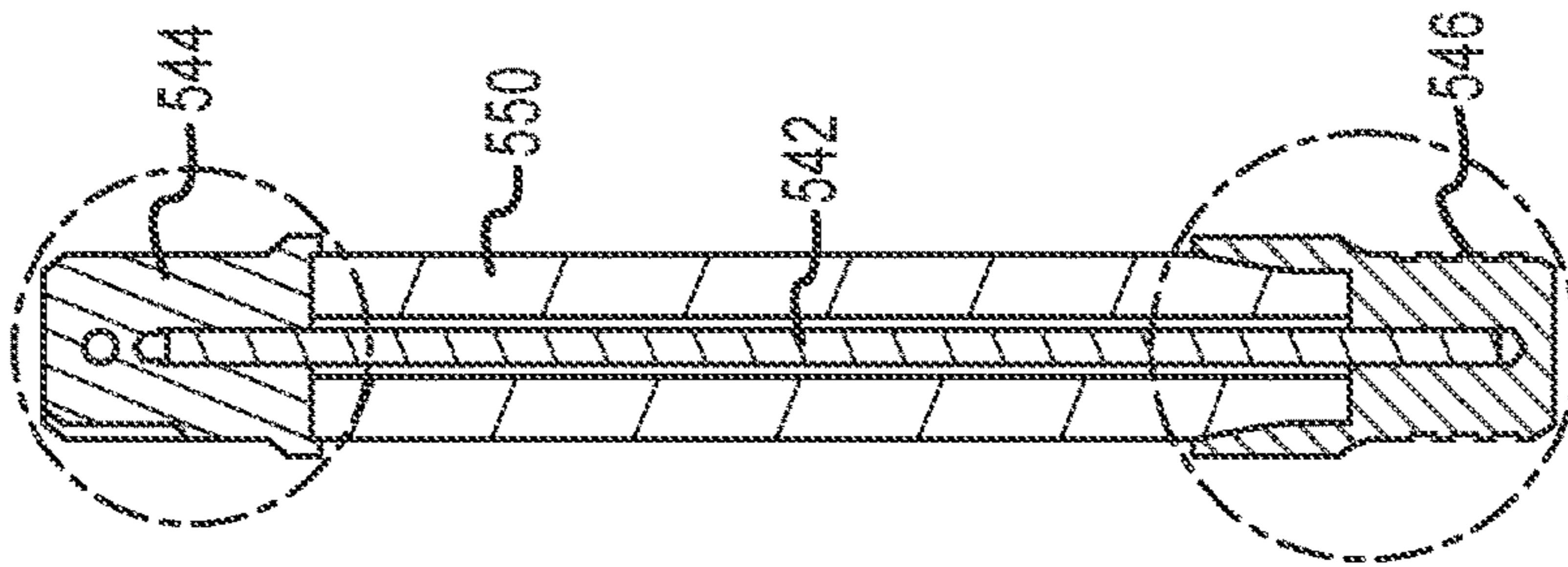
SECTION A-A
