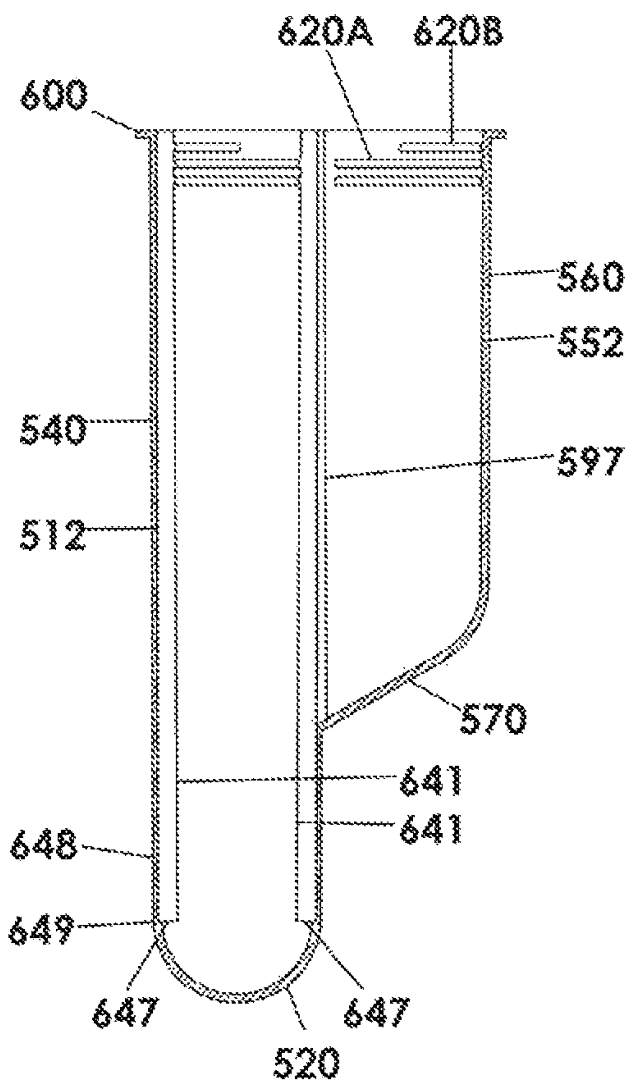
SECTION A-A
