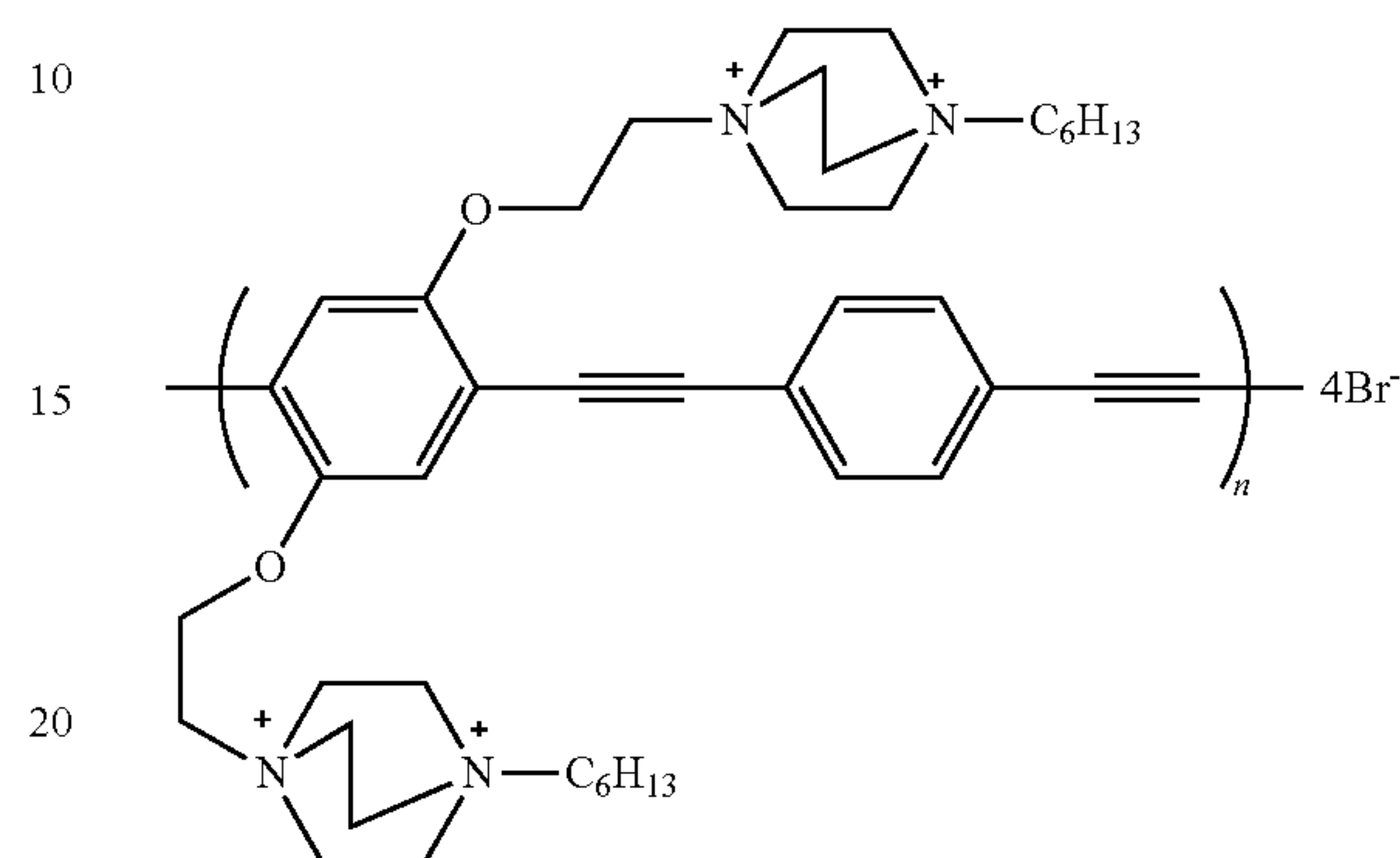
PPE-DABCO
