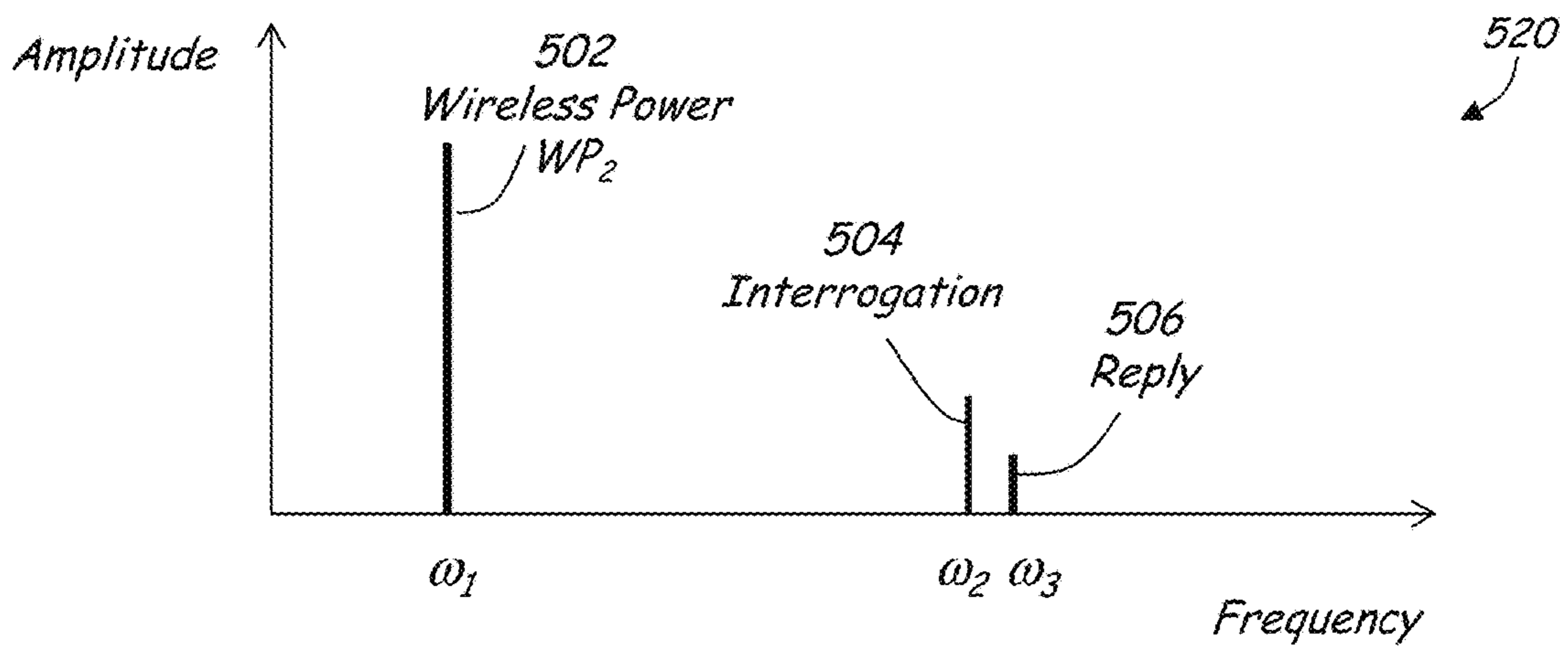
FIG. 5C
