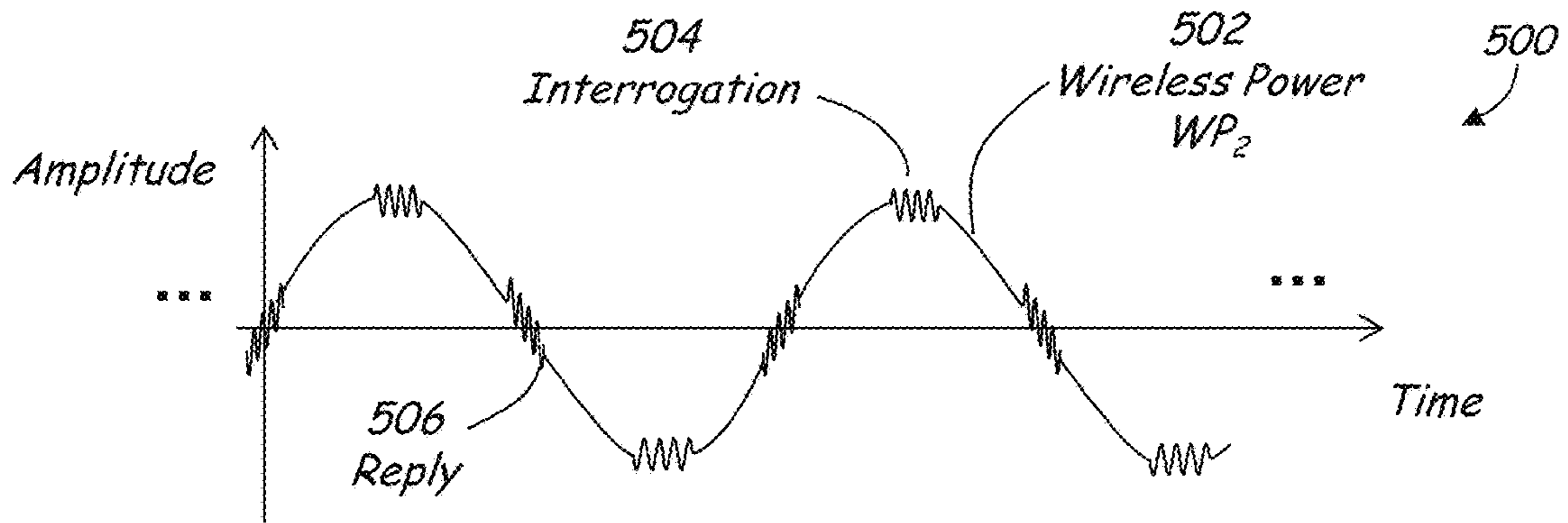
FIG. 5A
