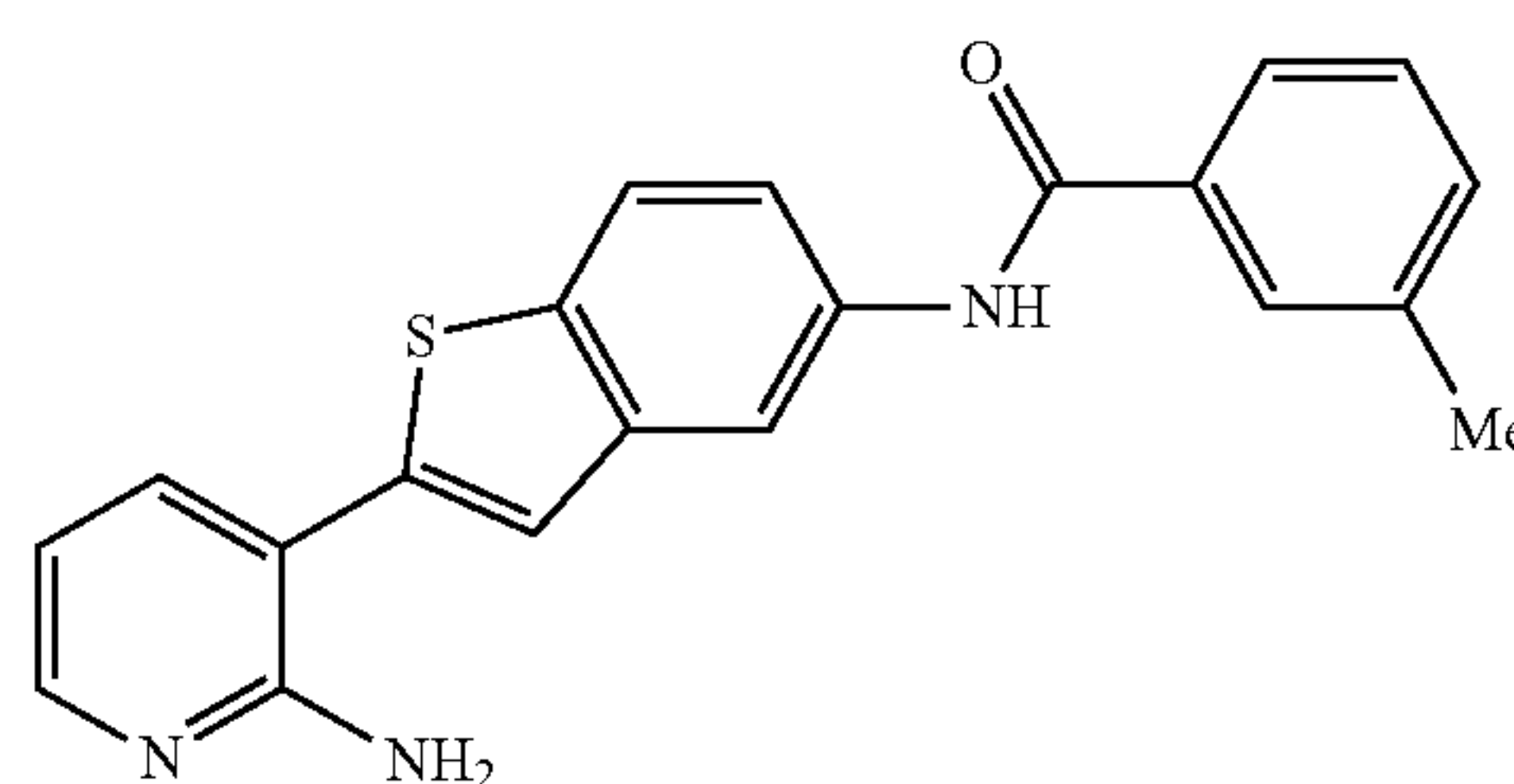
N-[2-(2-aminopyridin-3-yl)-1-benzothien-5-yl]-3-methylbenzamide
