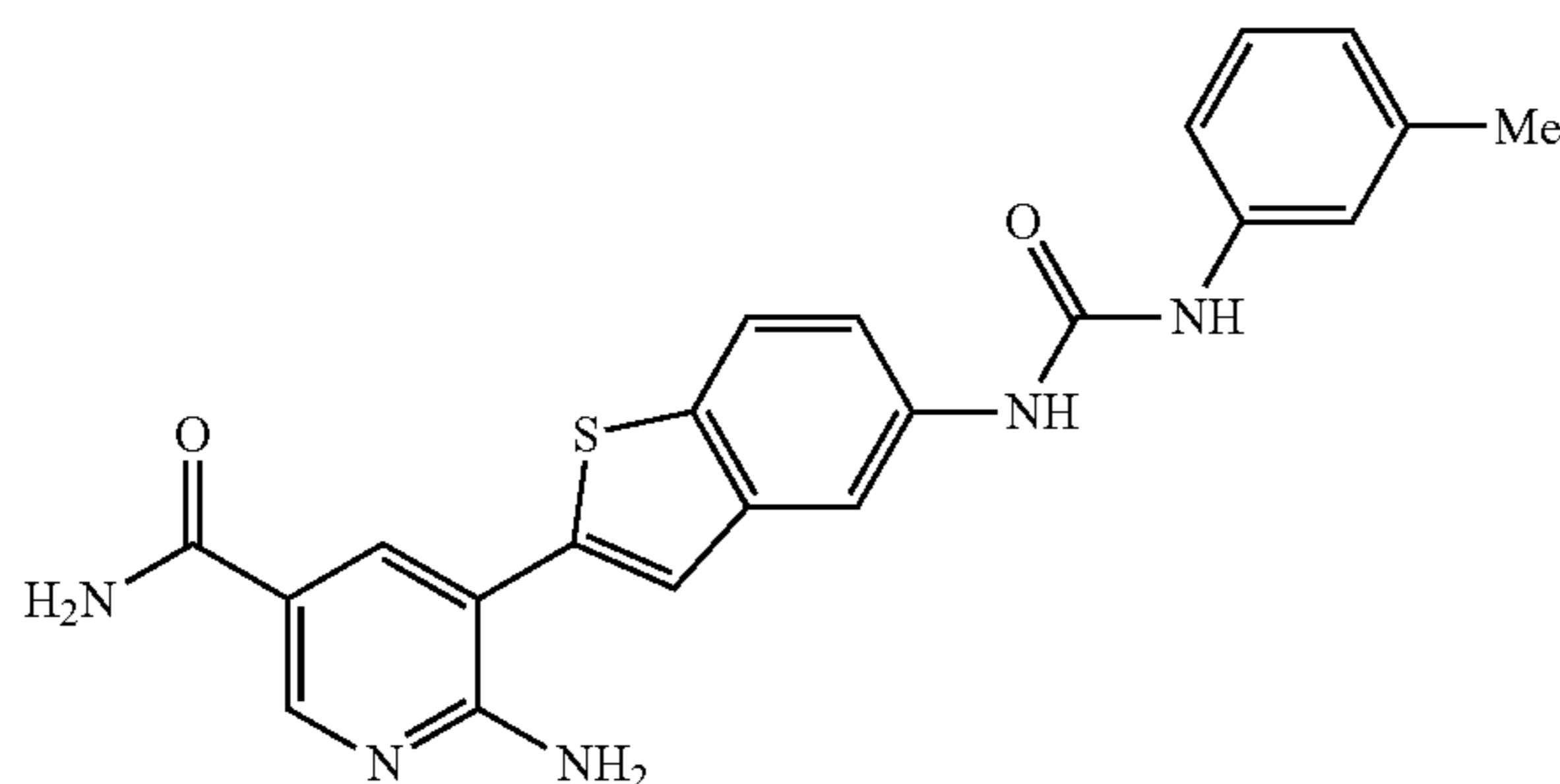
6-amino-5-[5-({[(3-methylphenyl)amino]carbonyl}amino)-1-benzothien-2-yl]nicotinamide
