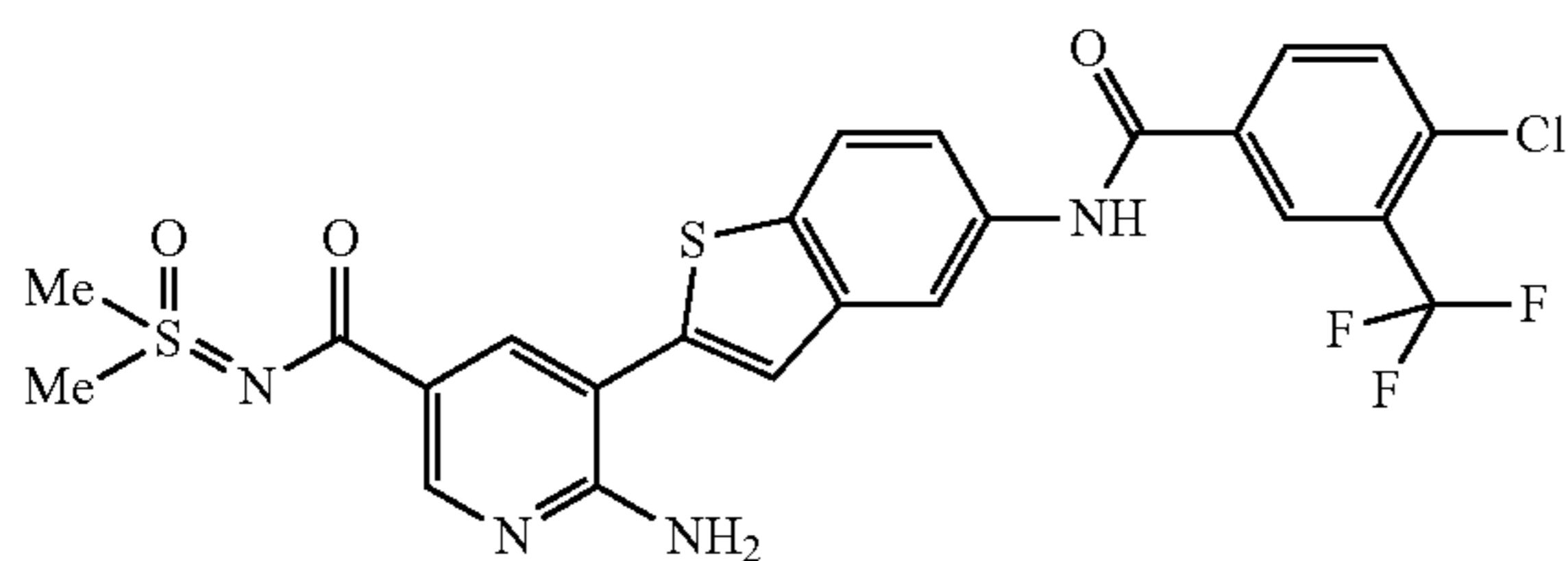
6-amino-5-(5-{4-chloro-3-(trifluoromethyl)benzoyl}amino)-1-benzothien-2-yl)-N-[dimethyl(oxido)-λ 4 -sulfanylidene]nicotinamide
