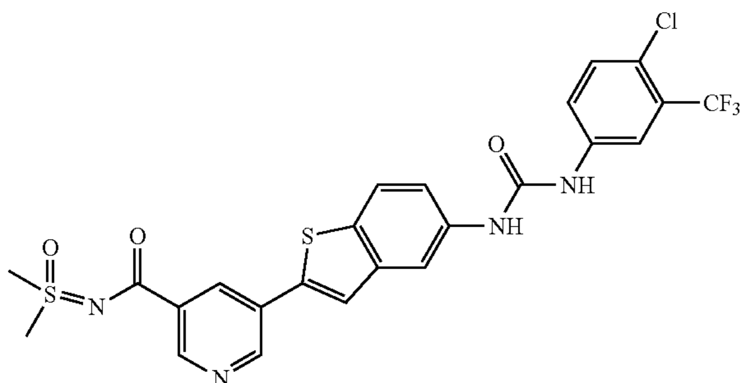
5-{5-[(4-chloro-3-(trifluoromethyl)phenyl)amino]carbonylamino}-1-benzothien-2-yl}-N-[dimethyl(oxido)- \lambda^4 -sulfanylidene]nicotinamide
