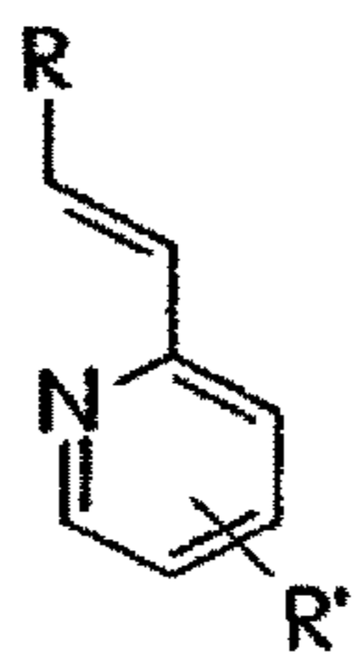
vinylpyridines
