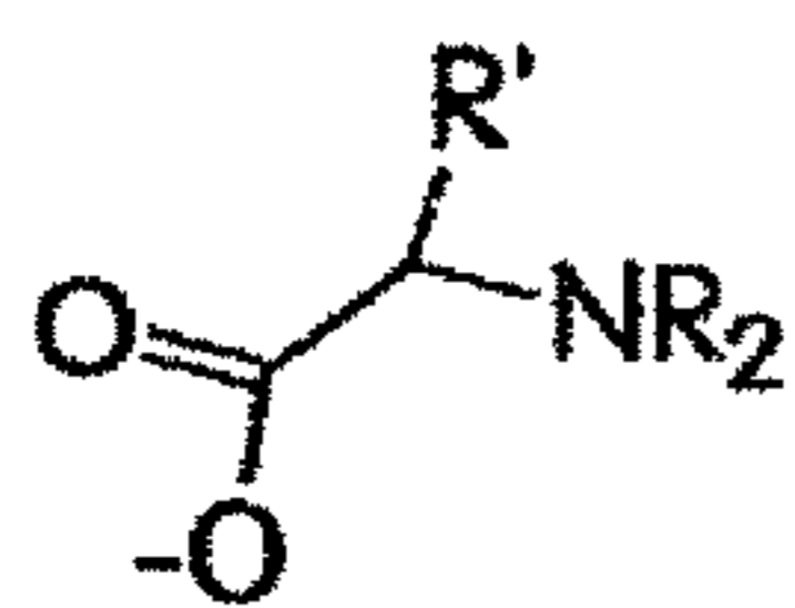
aminoacids
