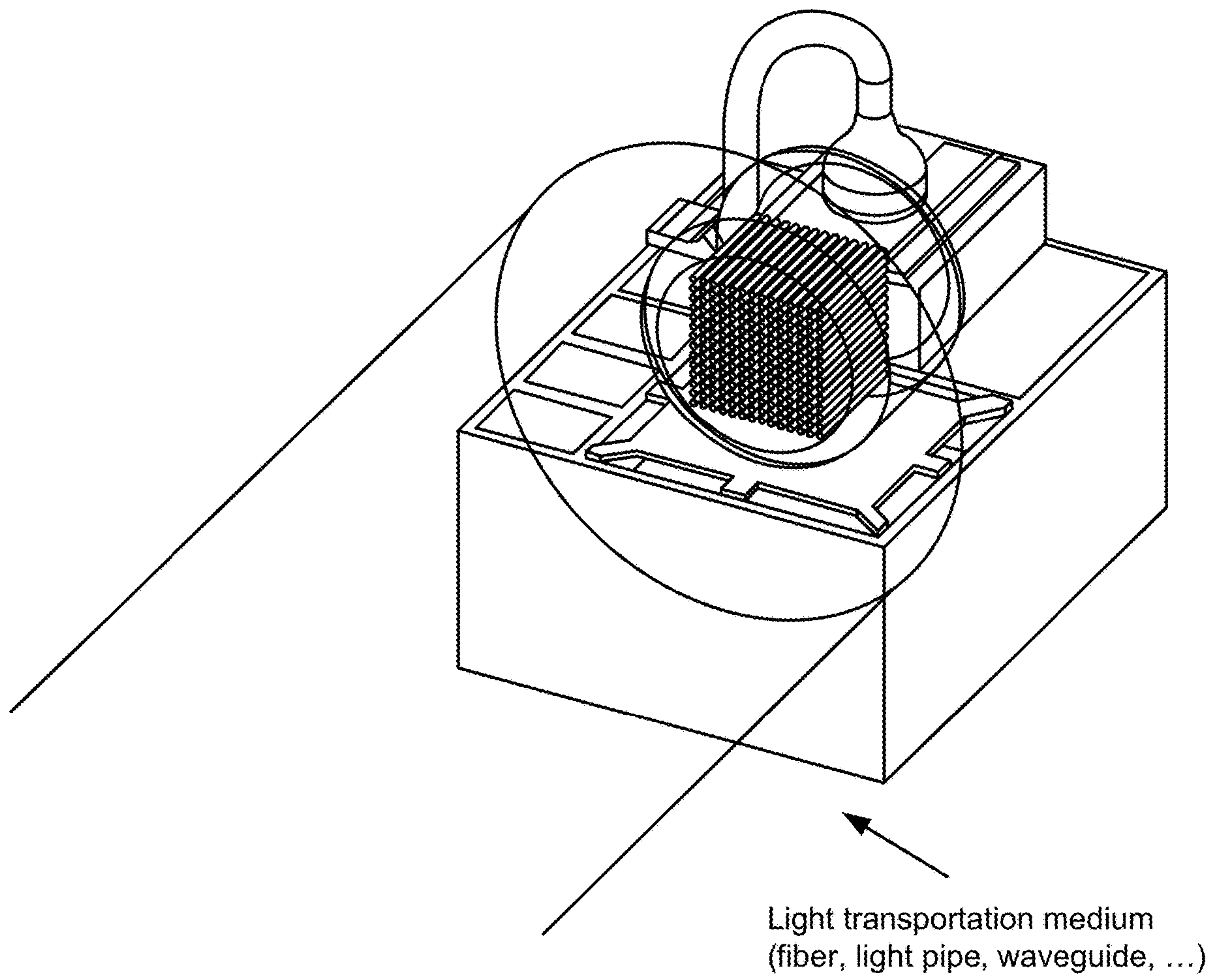
FIG. 22: Array or Module Configuration
