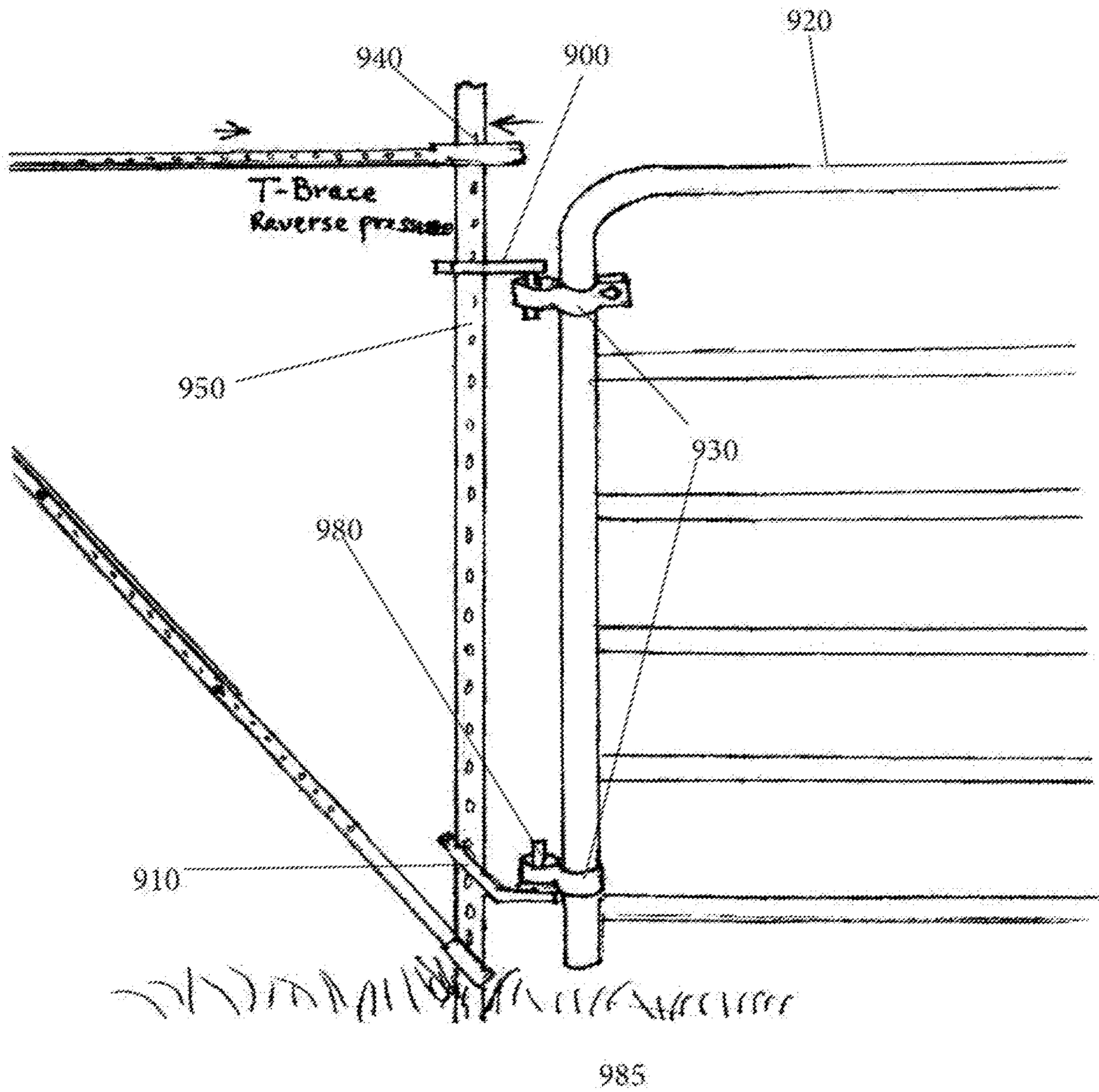
FIG. 10
