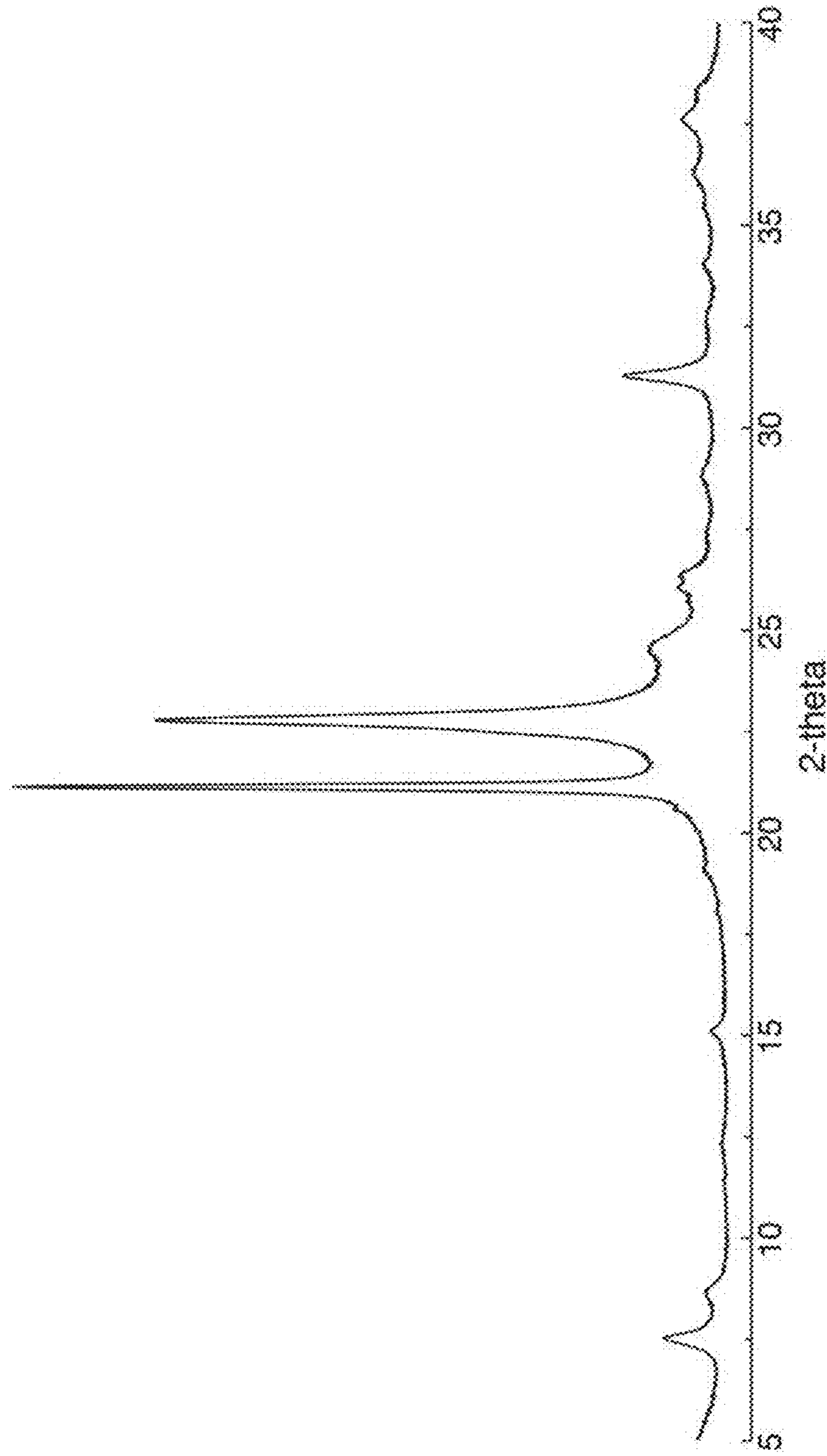
FIG. 5 (SSZ-91)
