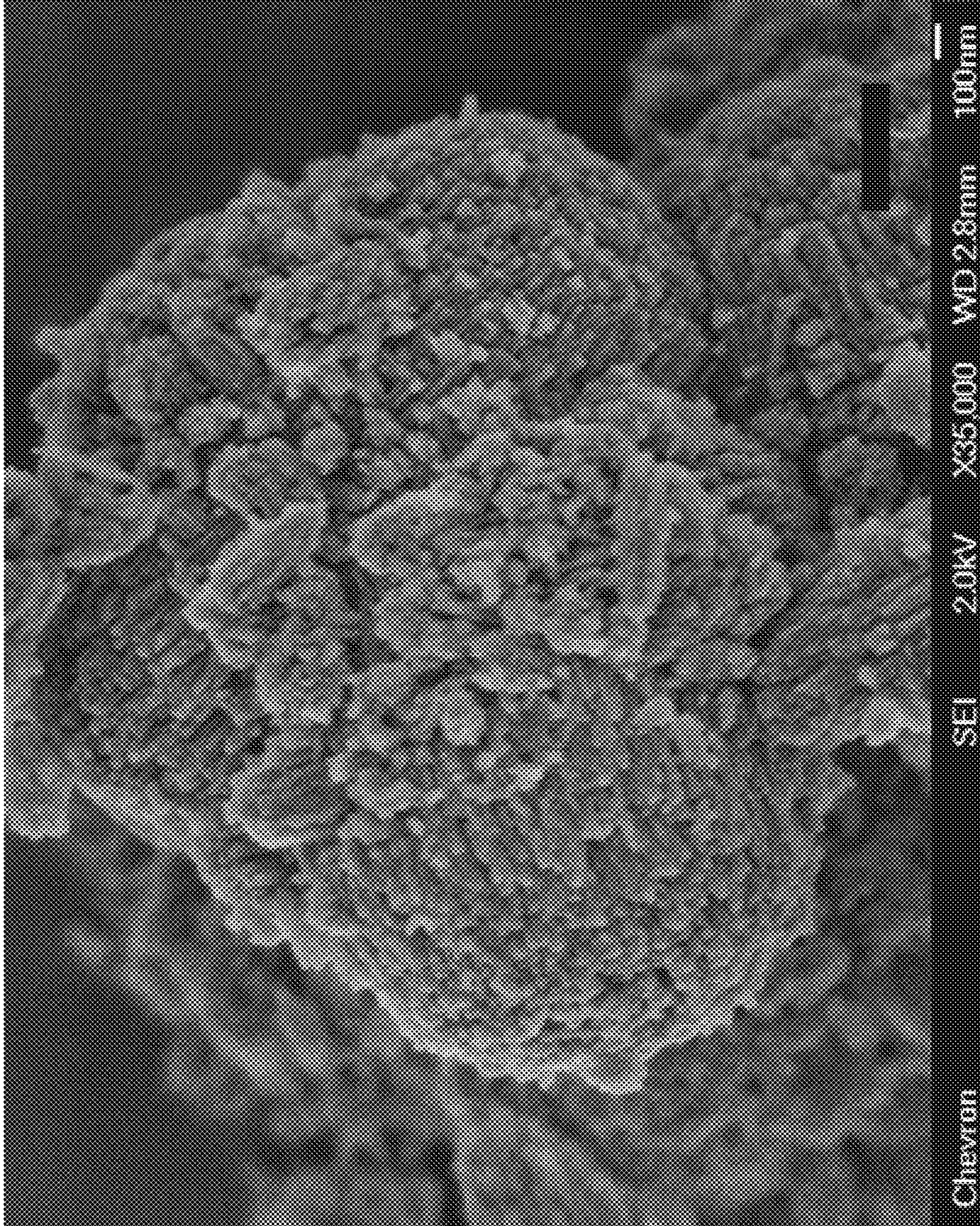
FIG. 7 (SSZ-91)
