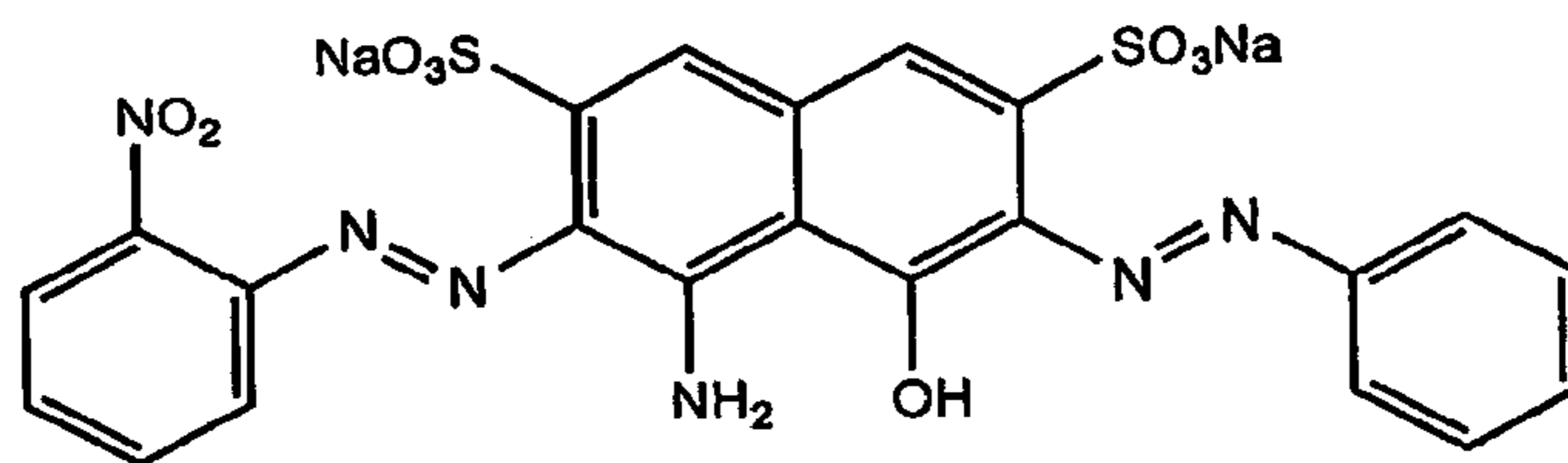
Acid Blue 29 (6) \lambda_{\max} : 602
