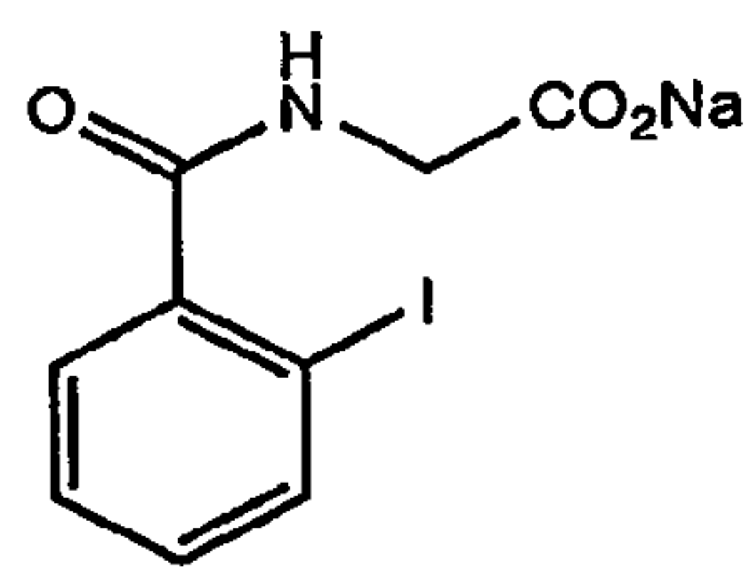
o-Iodohippurate (2) MW: 327
