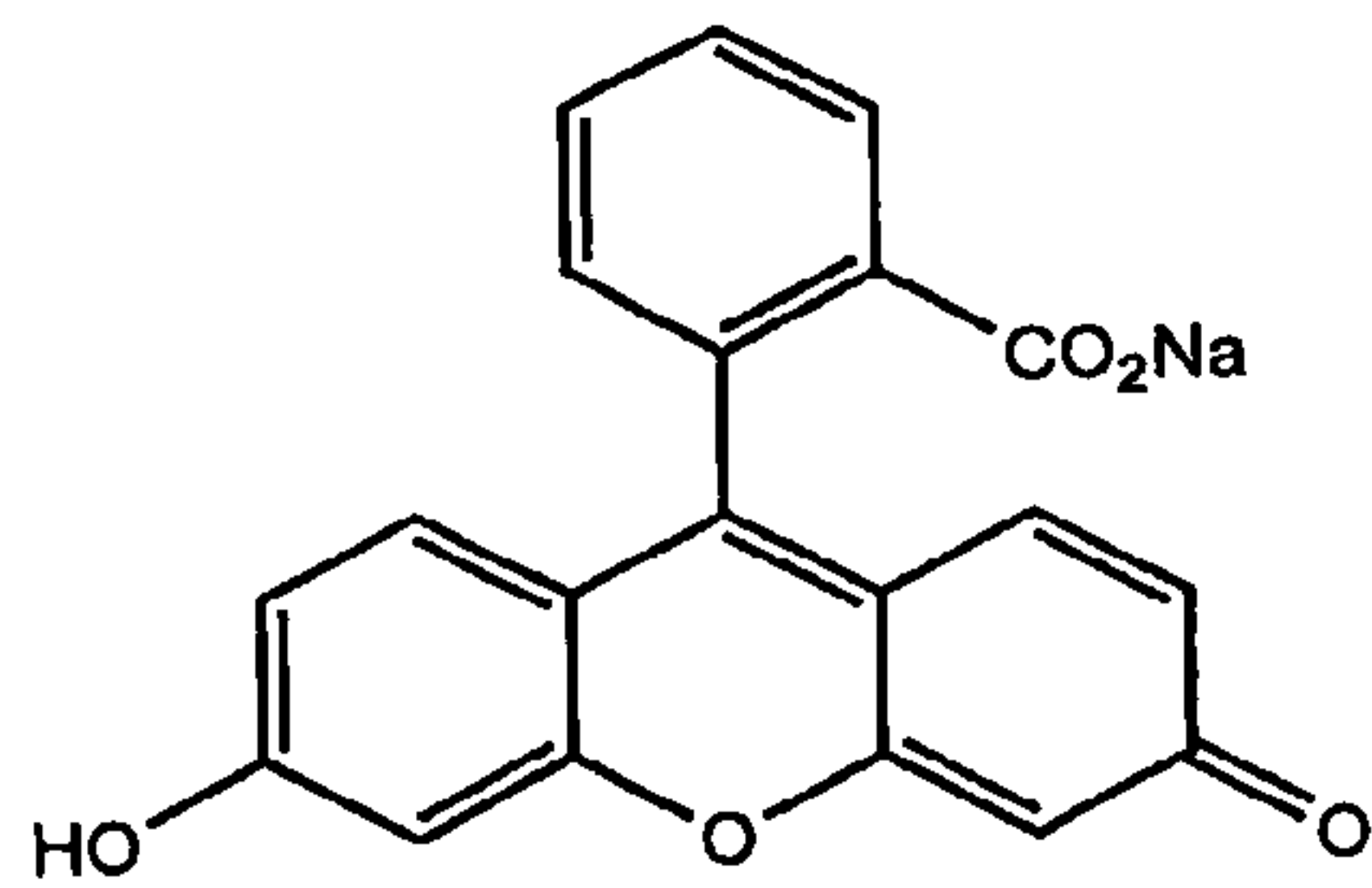
Fluorescein (5) \lambda_{\max} : 496
