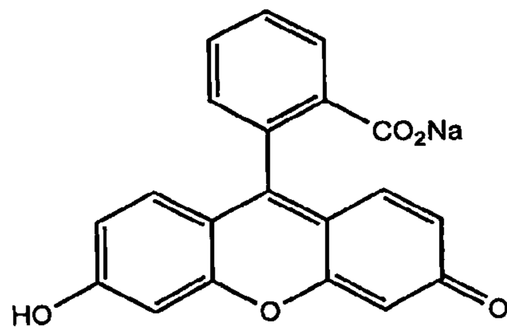
Fluorescein (5) \lambda_{\max} : 496
