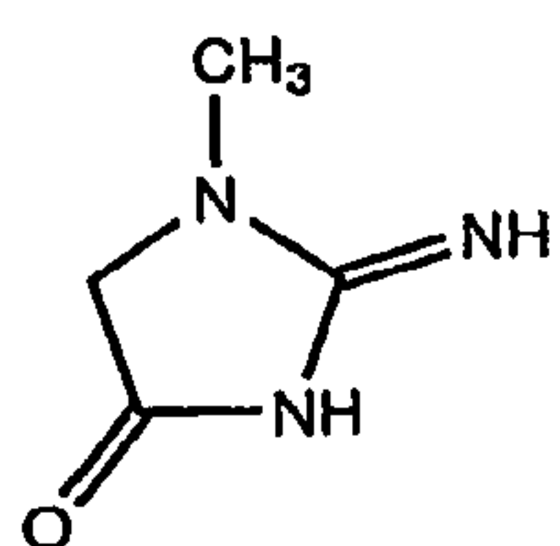
Creatinine (1) MW: 113
