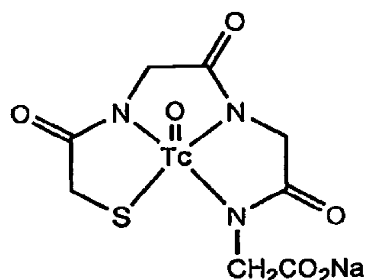
99m Tc-MAG3 (4) MW: 364
