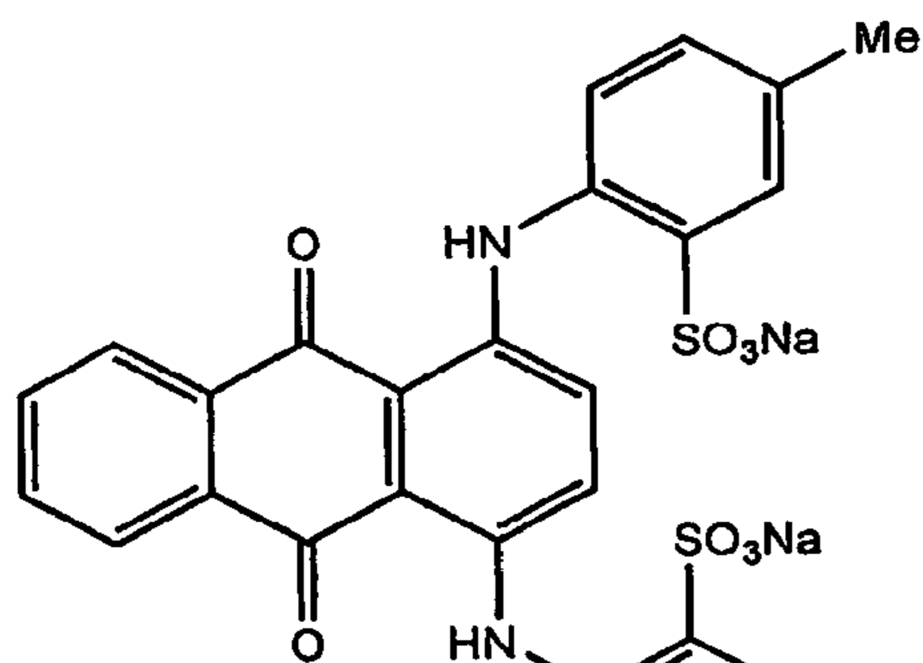
Acid Green 25 (7) \lambda_{\max} : 642
