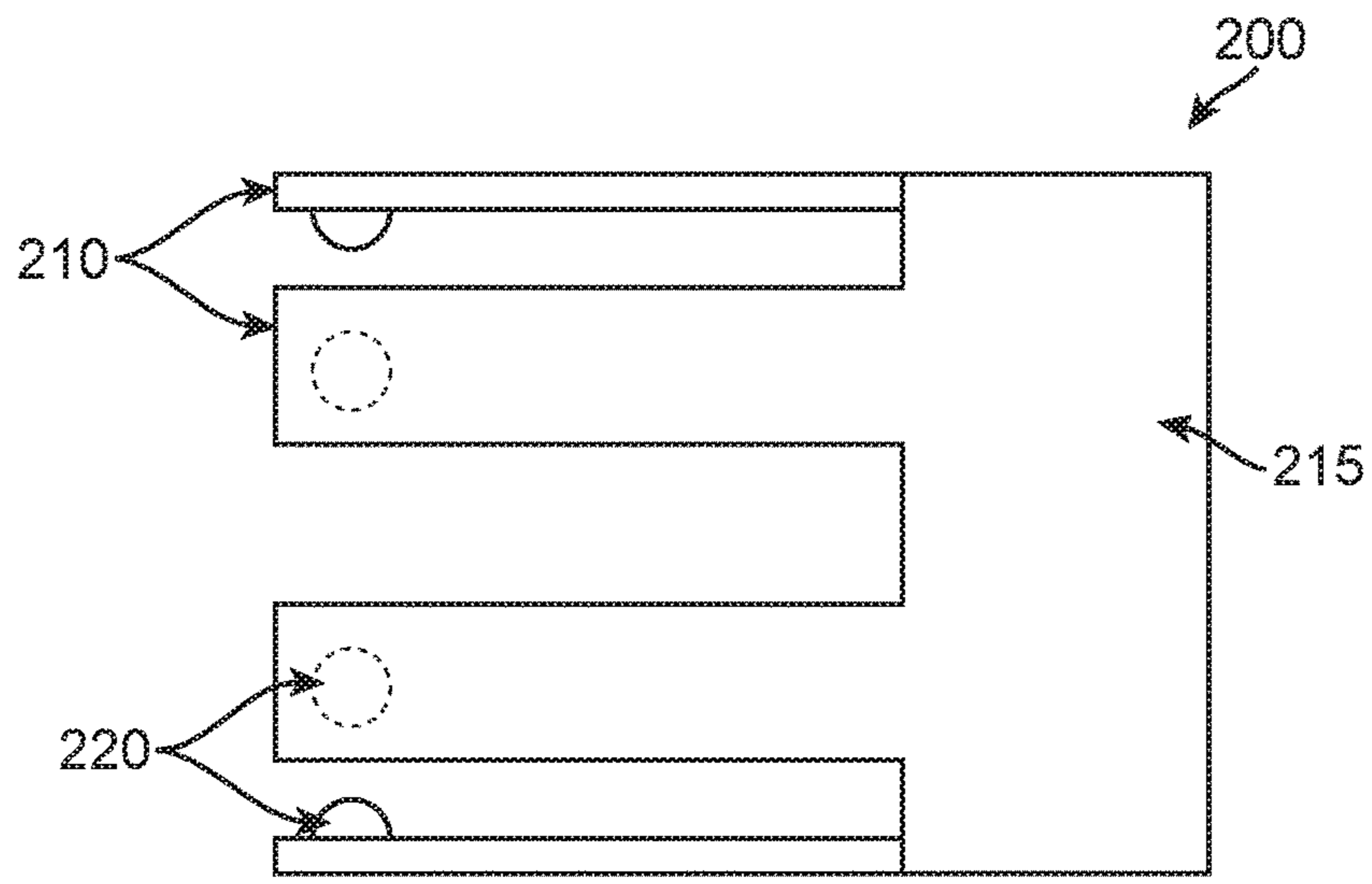
Top View FIG. 2A
