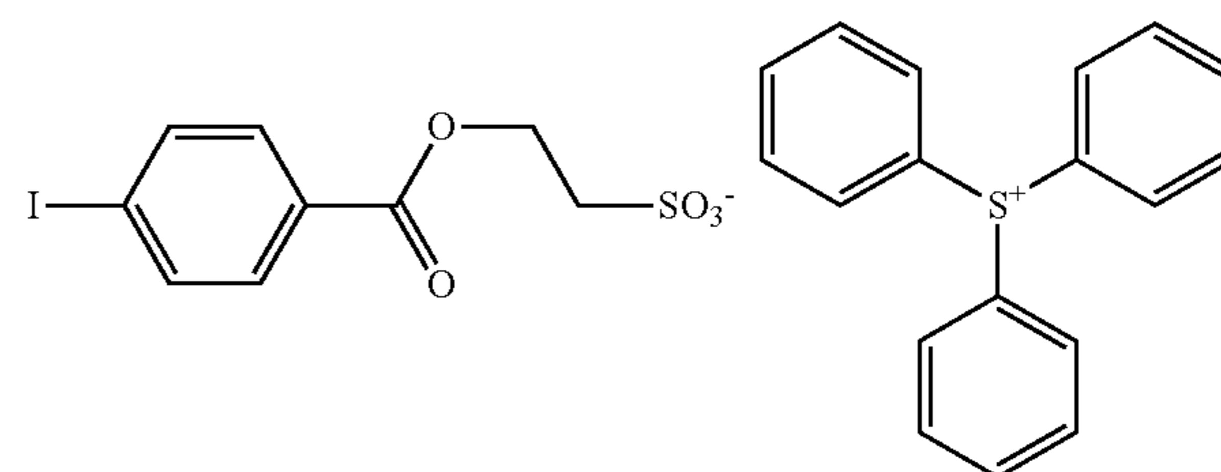
Sulfonium salt 1
