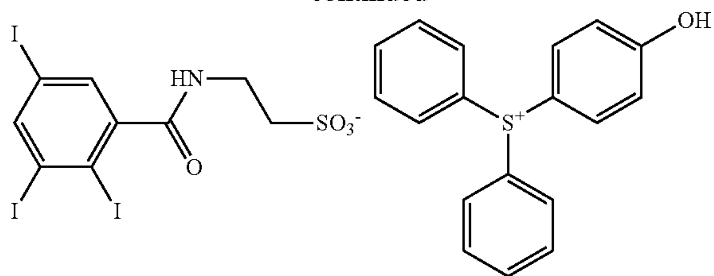
Sulfonium salt 5
