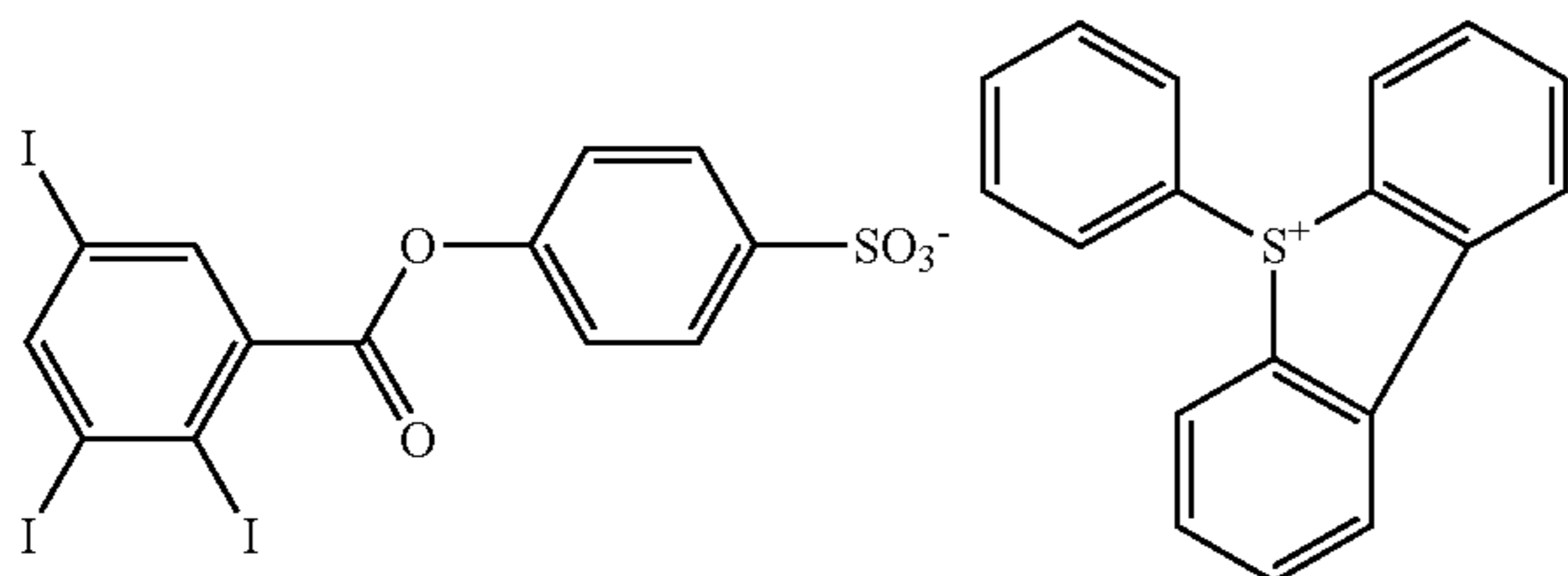
Sulfonium salt 10
