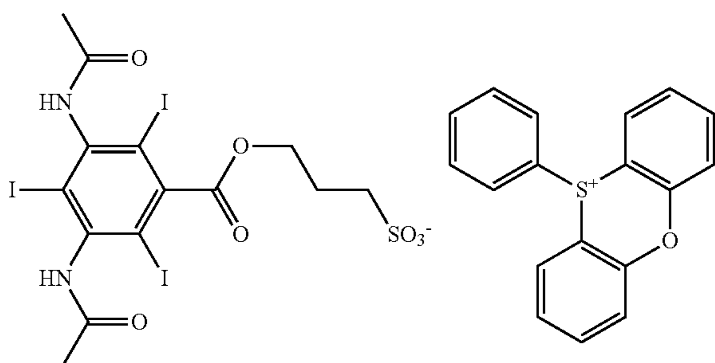
Sulfonium salt 7
