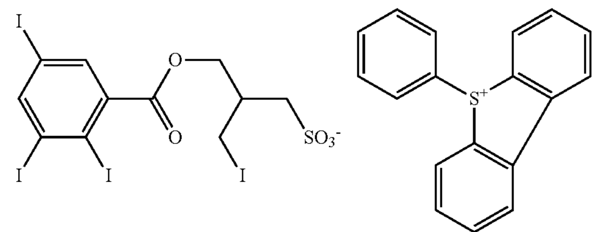
Sulfonium salt 9
