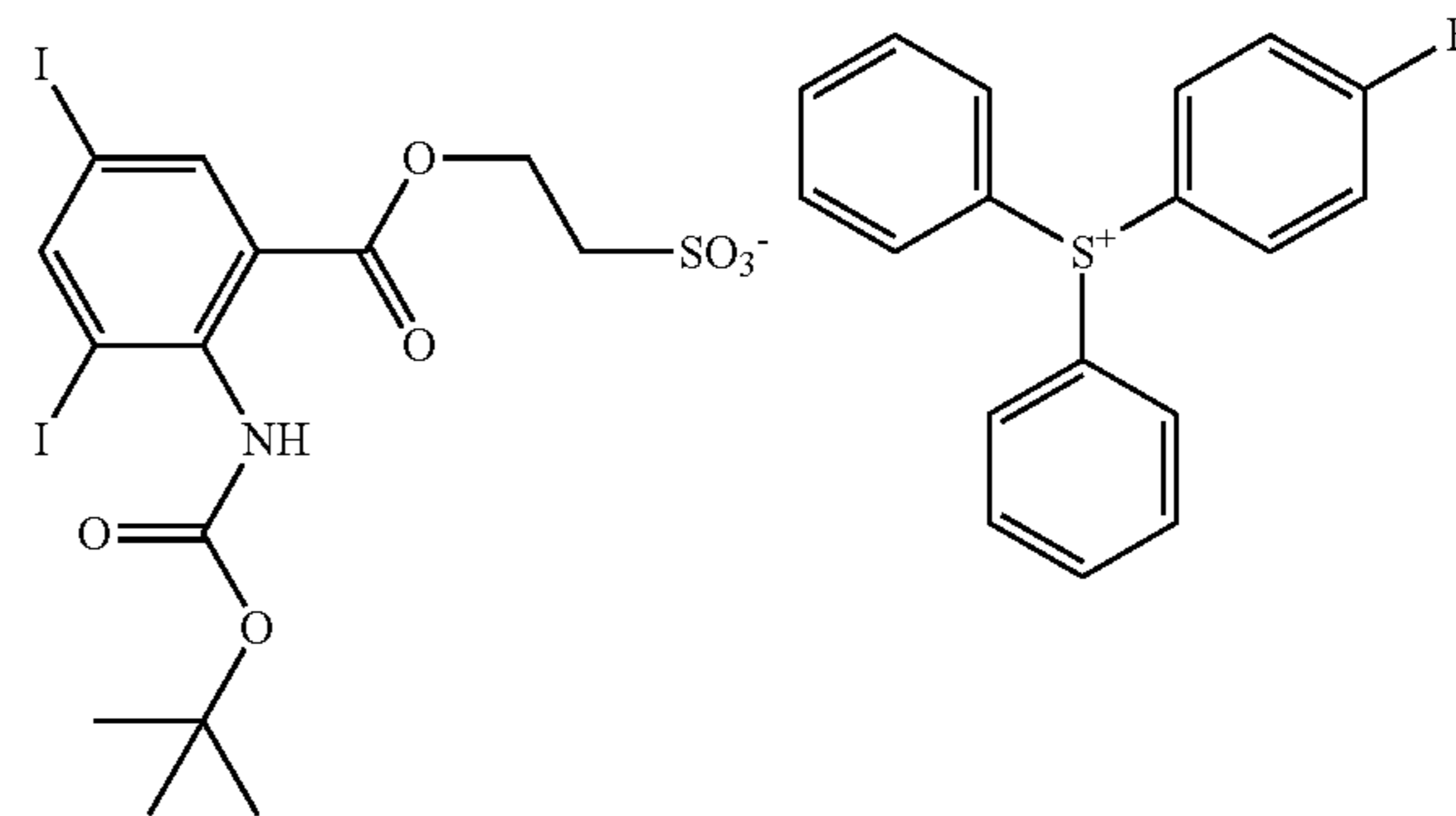
Sulfonium salt 3
