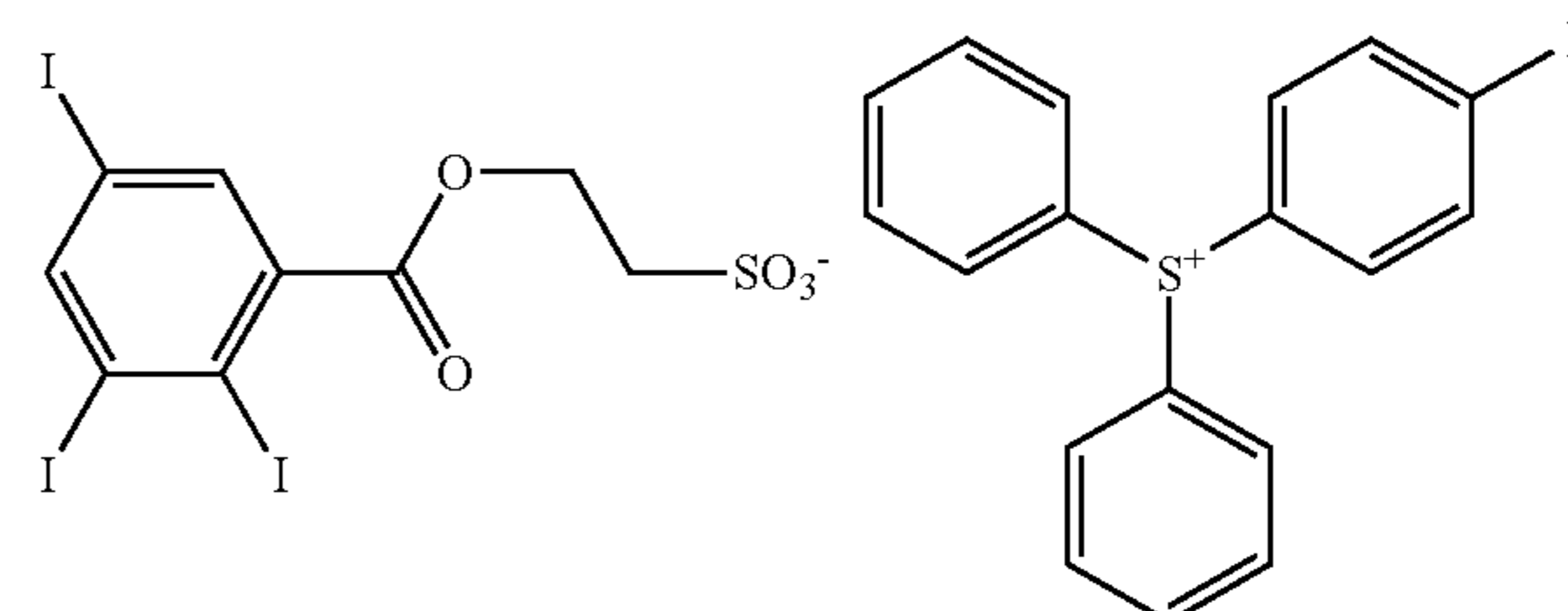
Sulfonium salt 4
