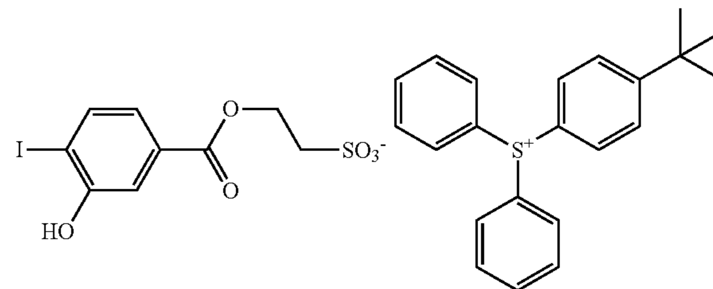
Sulfonium salt 2
